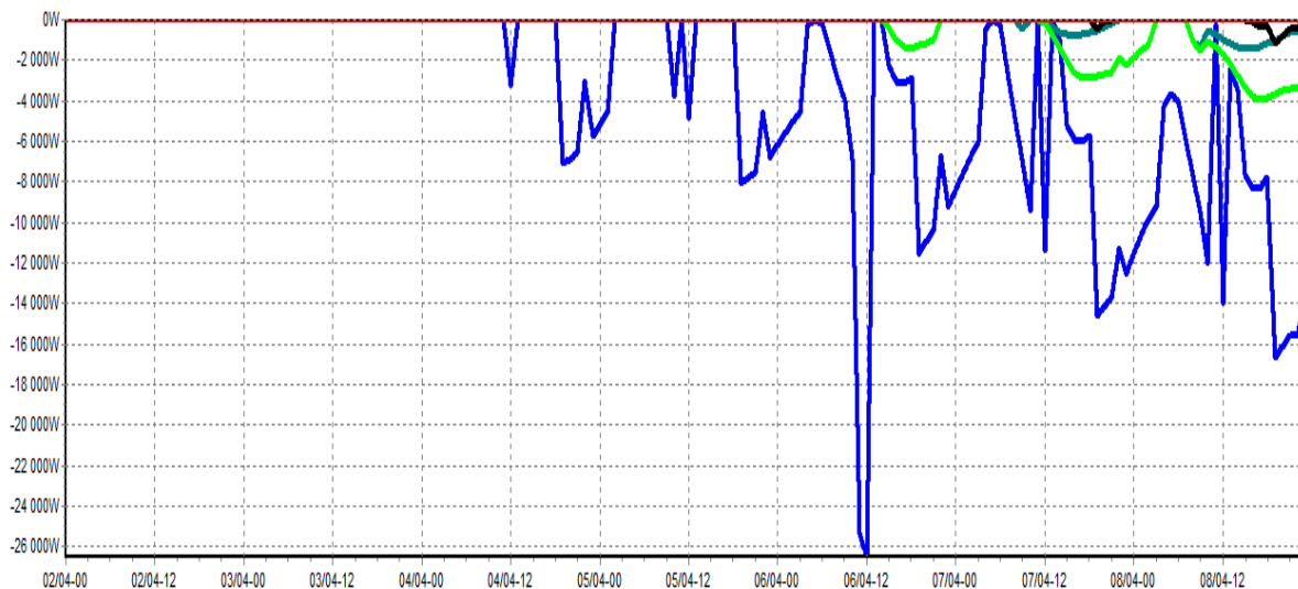
graphe3. 2 Diagramme de la puissance de climatisation consommé par les zones thermique [20]
