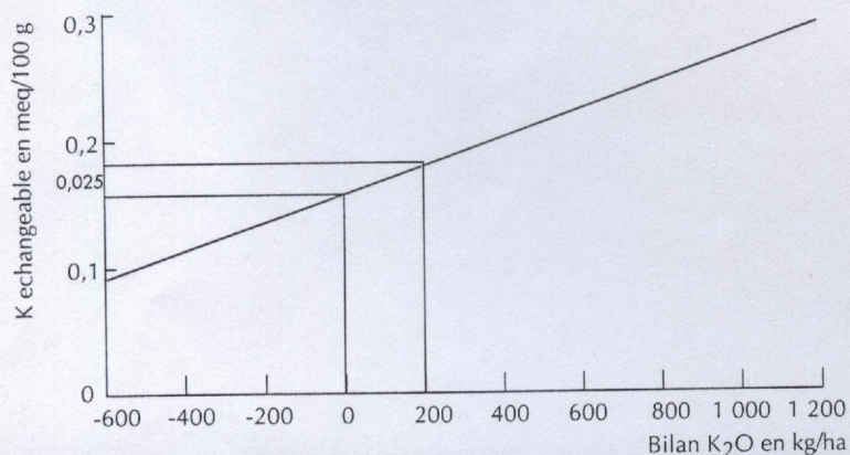
Figure 7. Relation entre le potassium échangeable et le bilan estimé en K_2O (essai de N'Tarla).
