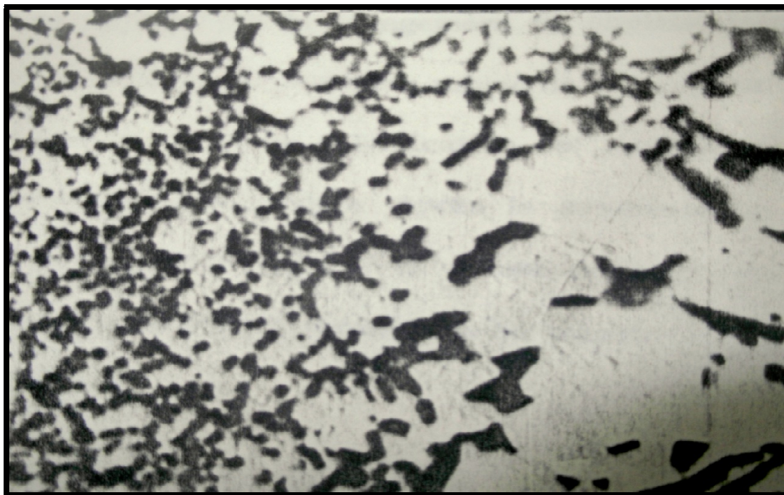
Figure V-12 : AS7 suivant la largeur du ruban (2000x) [7].
