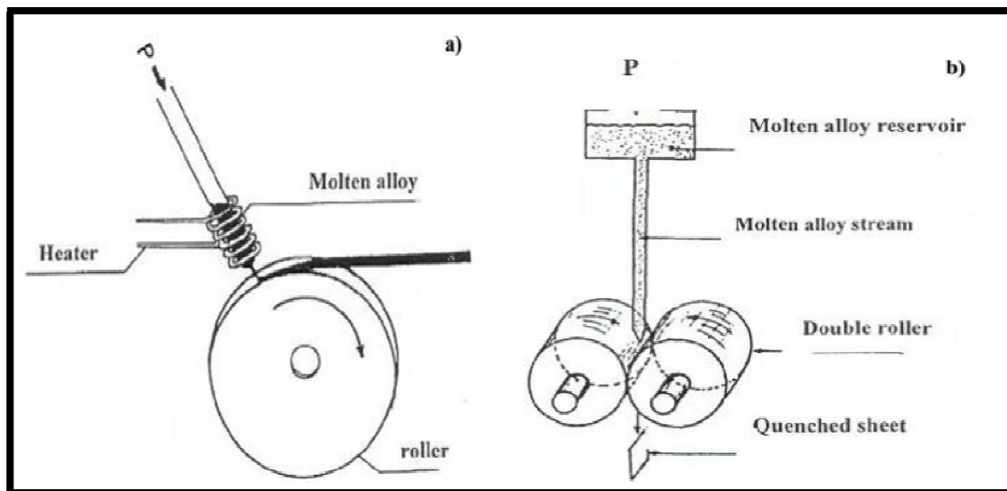
Figure II-3: Méthode de melt-spining a) avec une roue b) avec deux roues [1].
