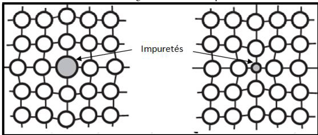
Figure I-4 : Défauts ponctuels [3].
