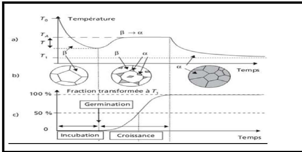
Figure I-3: Transformation allotropique \beta \rightarrow \alpha d'un corps pur à T_A .
