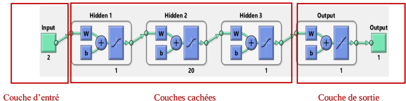
Figure II.11 : Architecture du réseau de neurone RNA (hiver).
