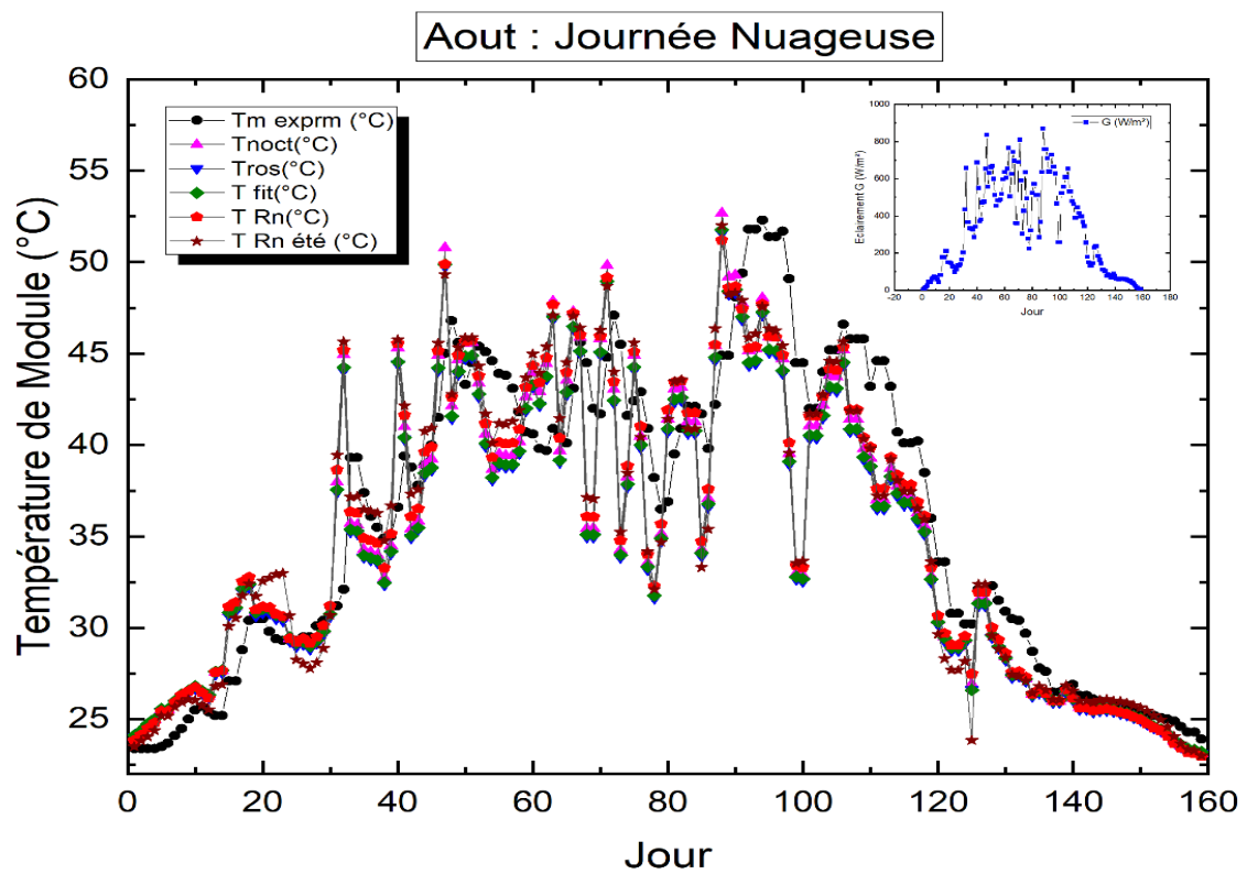
Figure III.06 : Validation d'une journée nuageuse du mois d'août.
