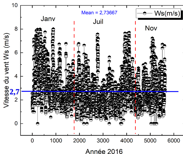
Figure II.03: Vitesse du vent ( W_s ) mesurée pour l'année 2016, mois : Janvier, Juillet et novembre.
