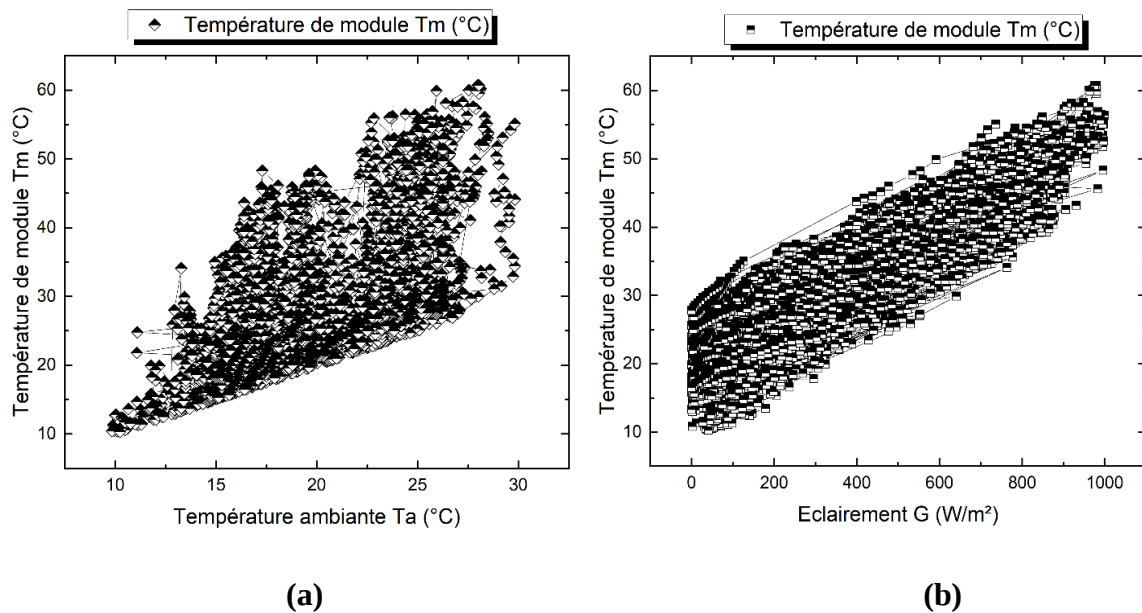
Figure II.06: Température de module PV ( T_m ) en fonction de la température ambiante ( T_a ) et de l'éclairement ( G ) : (a) T_m = f(T_a) (b) T_m = f(G) .
