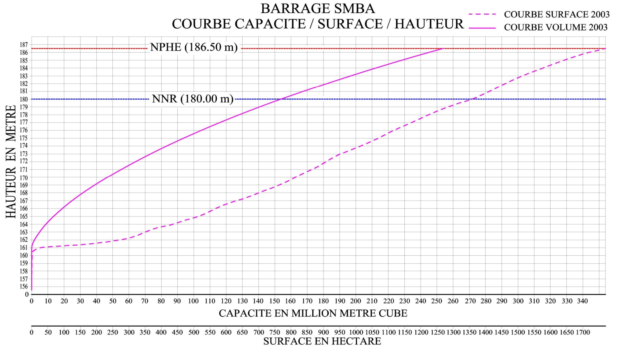
Fig. V.18: Courbe capacité/ surface/ hauteur du barrage SMBA, 2003 (ANBT).
