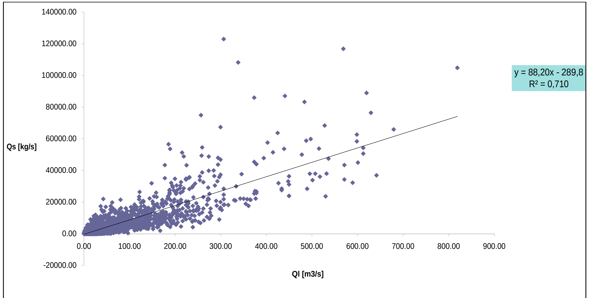
Fig. V.9: Relation entre le débit solide Q_s [kg/s] et le débit liquide Q_l [m³/s] de l'Oued Mina (Période 1971-2001)-annuel.
