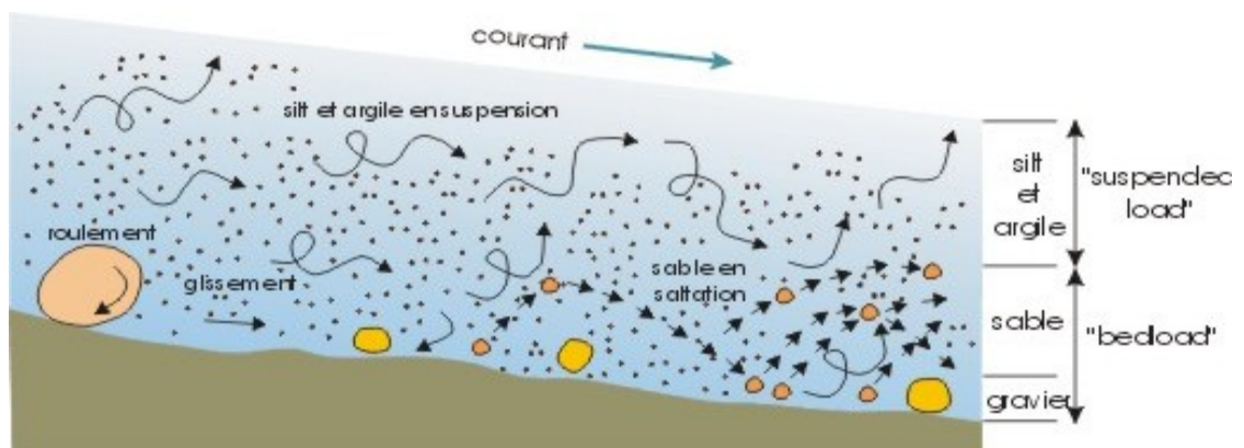
Fig. II.8: Différents types des particules qui se trouvent en suspension lors d'un écoulement.
