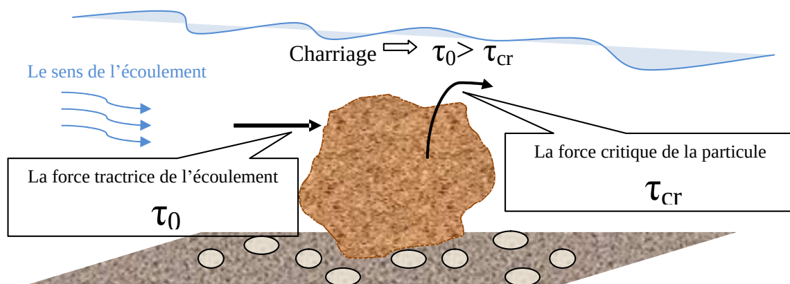
Fig. II.5: Principe du charriage d'une particule.
