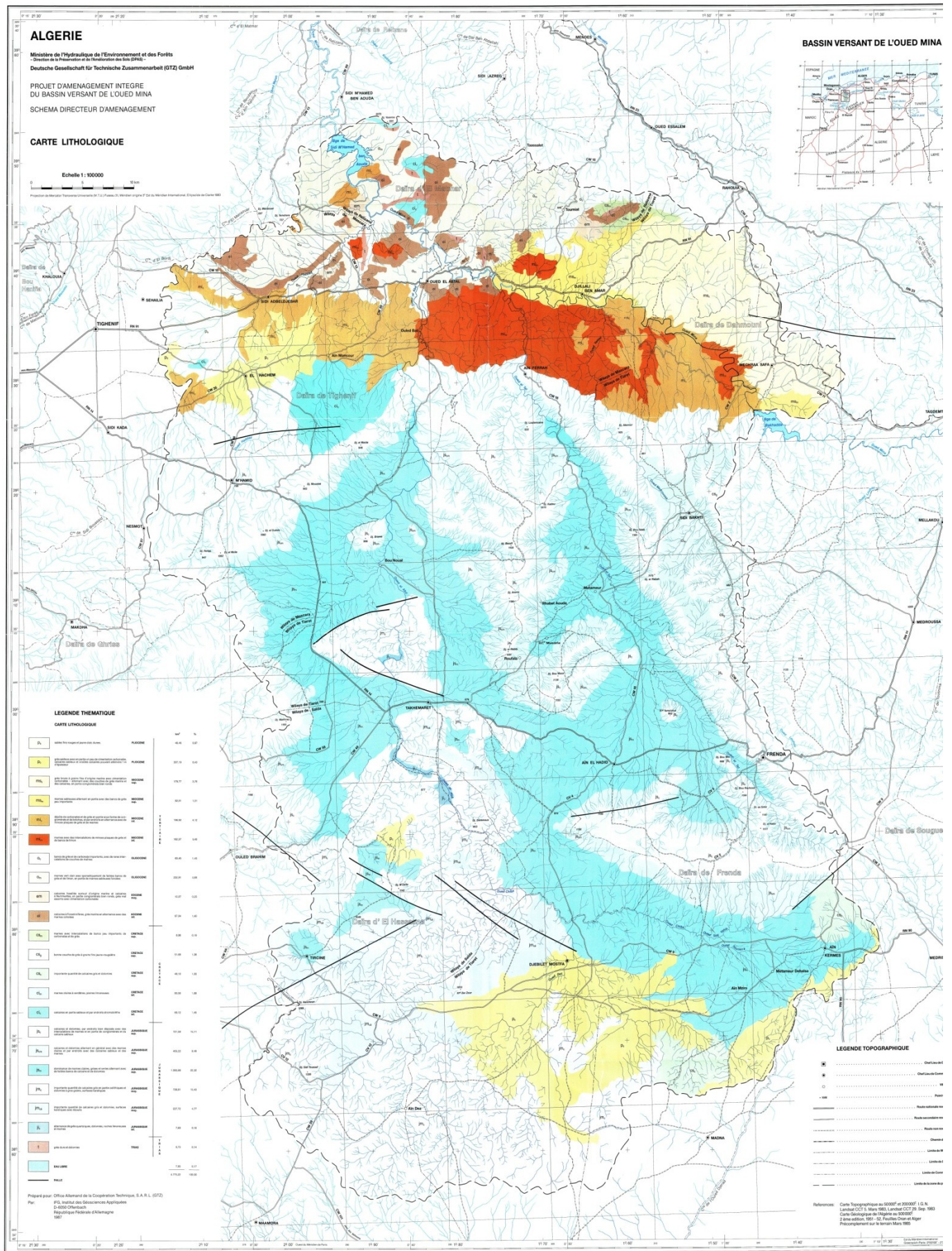
Fig. V.4: Carte lithologique du bassin versant de l'Oued Mina (Source : Ministère de l'Hydraulique de l'Environnement et des Forêts)
