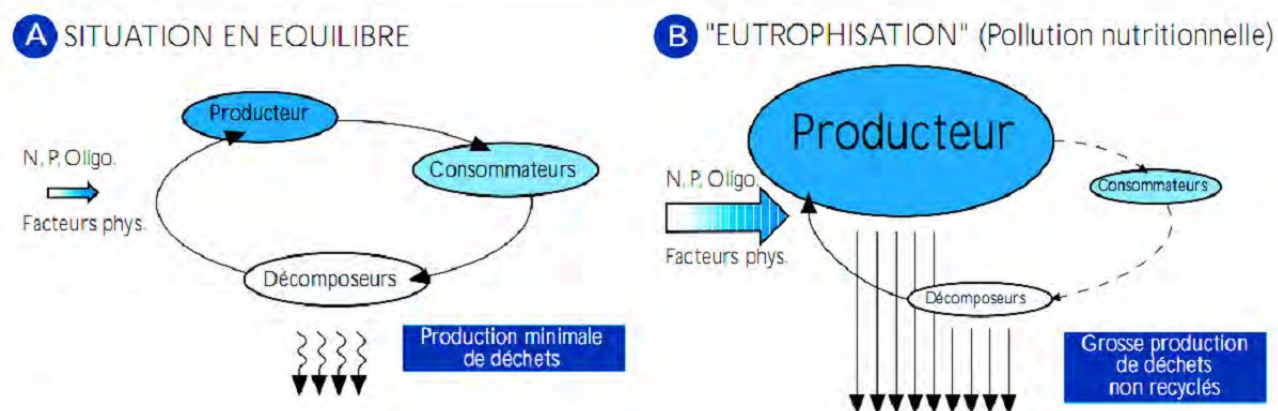
Fig. IV.1 Représentation schématique du phénomène d'eutrophisation. (BAVARD J., 2010)
