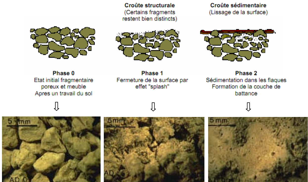
Fig. 1.2: Formation de la croûte de battance. (TRIBOUILLARD C., 2004)
