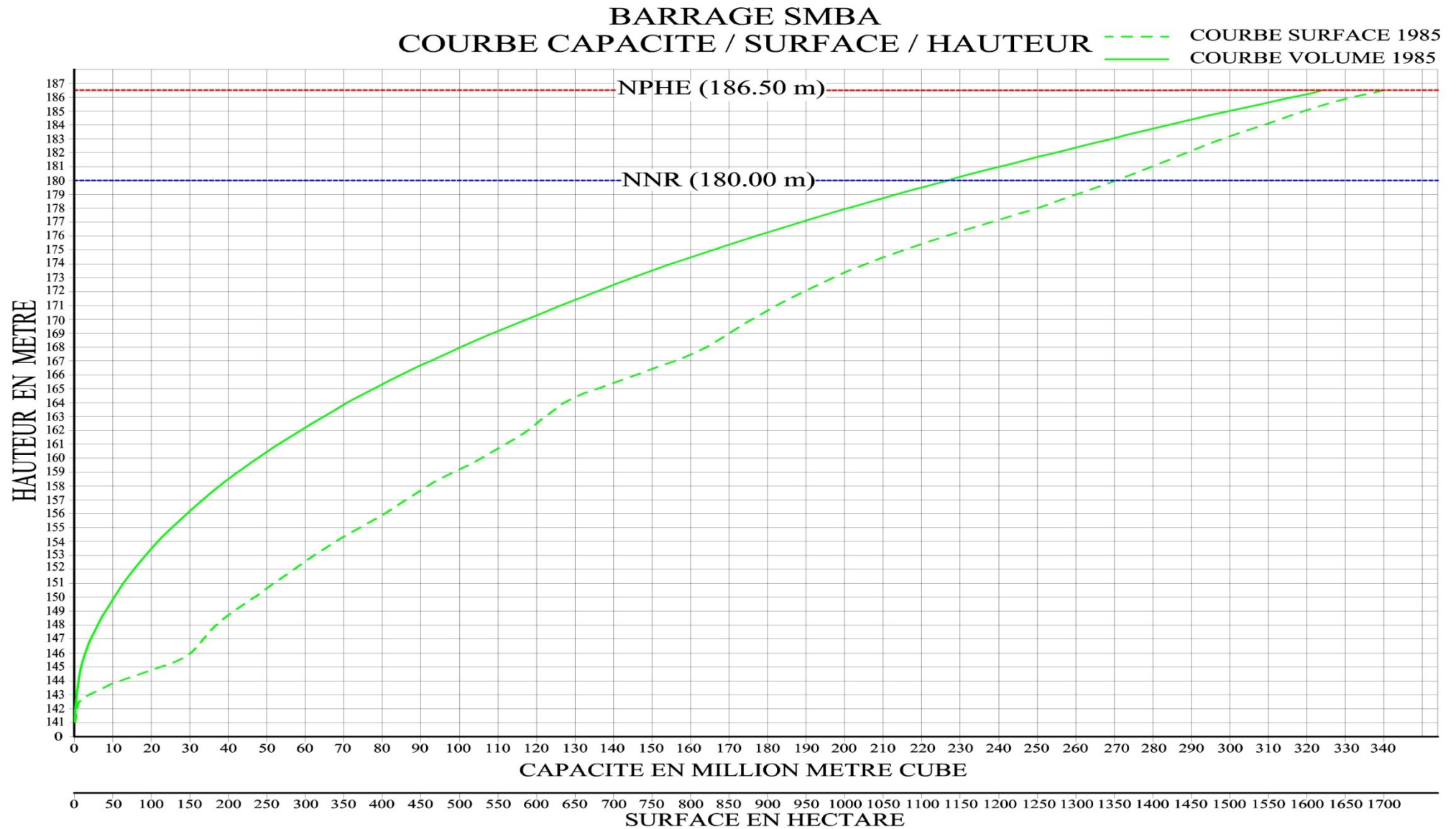
Fig. V.17: Courbe capacité/ surface/ hauteur du barrage SMBA, 1985 (ANBT).
