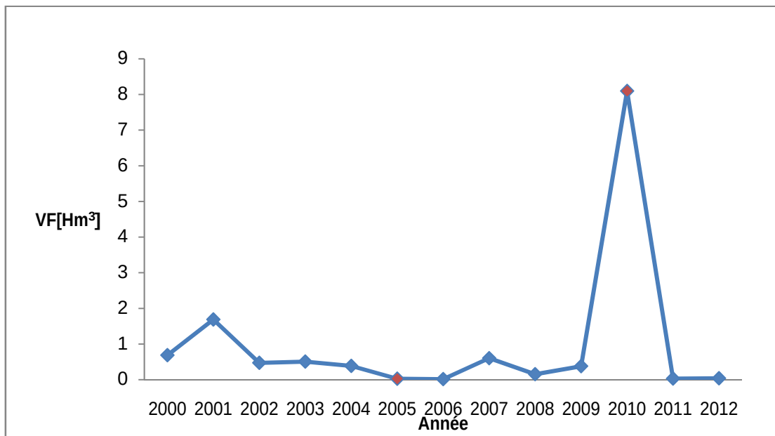
Fig. V.28: Variation annuelle du volume de dévasement pendant le Vidange de fond du barrage SMBA en fonction du temps (période: 2000-2012).
