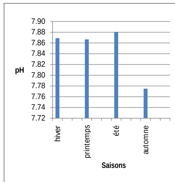
Fig. V.25: variation saisonnière du pH (période: 2000-2011).
