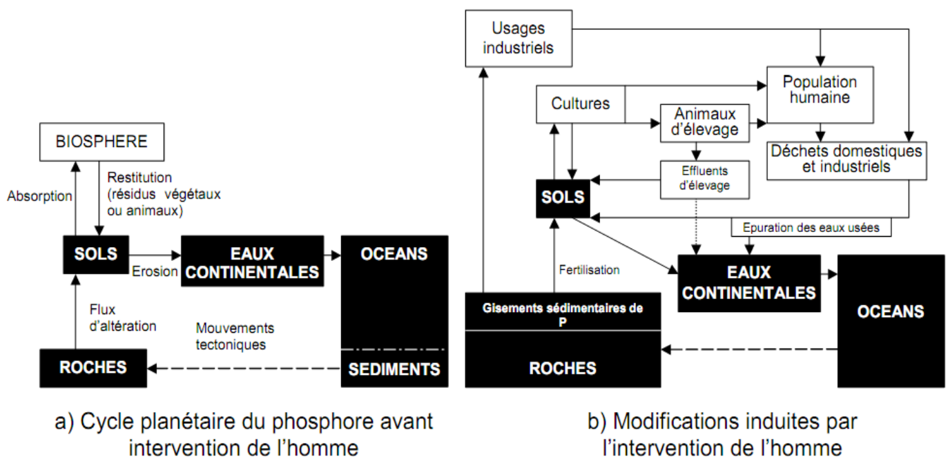
Fig. IV.2 Cycle du phosphore avec ou sans perturbation anthropique (d'après Pellerin S). (LEMERCIER B., 2003)
