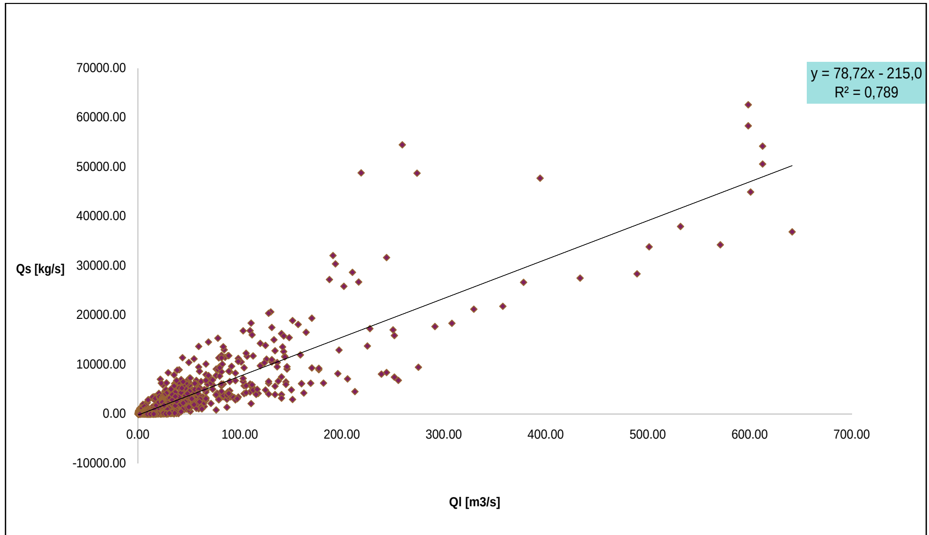
Fig. V.11: Relation entre le débit solide Q_s [kg/s] et le débit liquide Q_l [m³/s] de l'Oued Mina (période 1971-2001)-saison de printemps.
