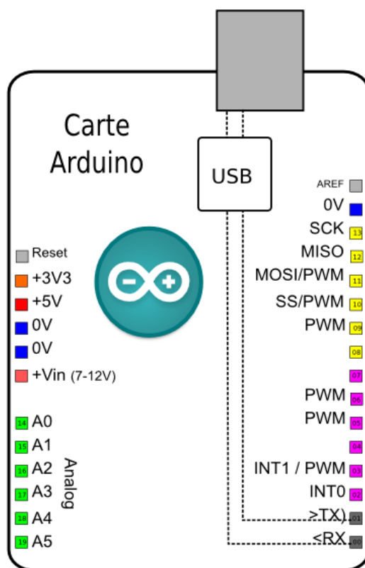
Figure 2.3 : Brochage de la carte Arduino Uno.
