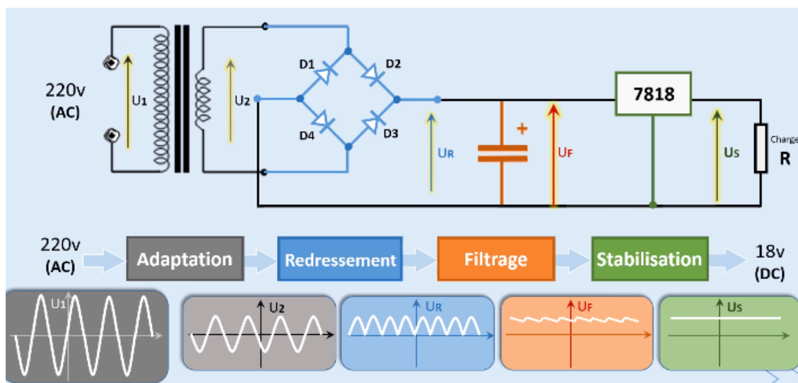
Figure 3.30 : Schéma d'alimentation stabilisé.
