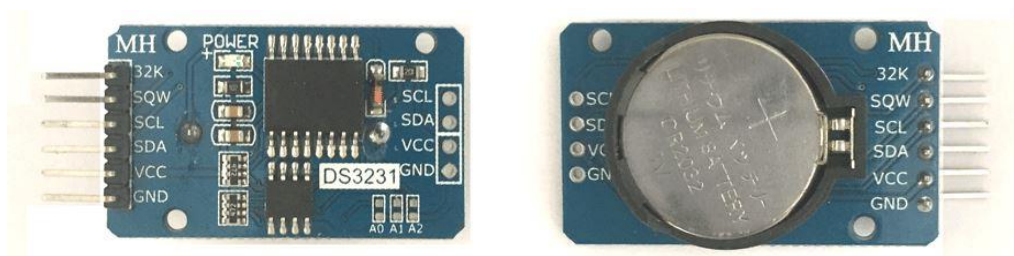
Figure 3.11 : RTC DS3231 du haut and et en bas.
