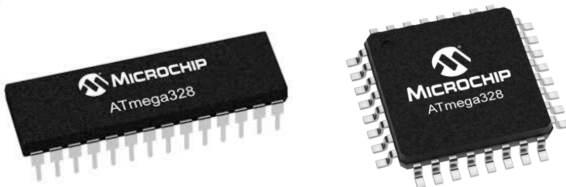
Figure 2.2 : ATmega238 classique et CMS.
