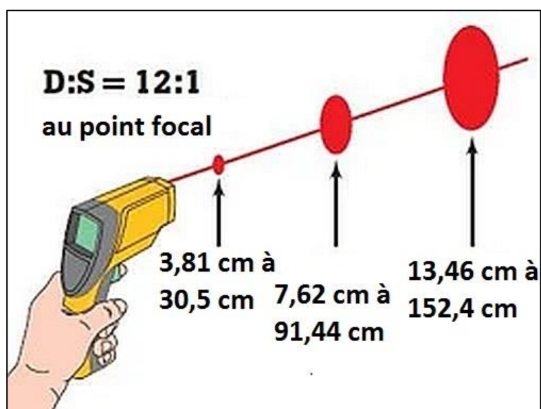
Figure 1.7 : le diamètre du point de mesure relevé à trois distances avec un thermomètre infrarouge.
