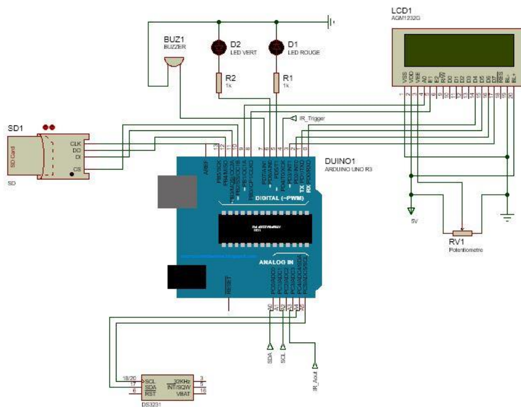
Figure 3.39 : Schéma général partie 1.
