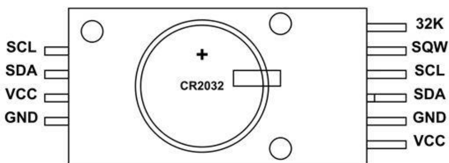
Figure 3.12 : Les pins du DS3231.
