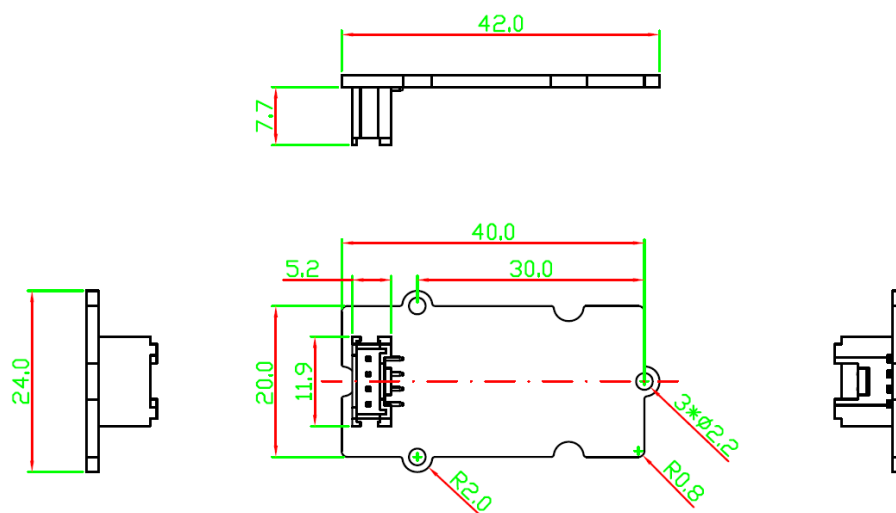
Figure 3.4 : Le dessin technique d'un capteur Grove 20X40 SMD vertical.
