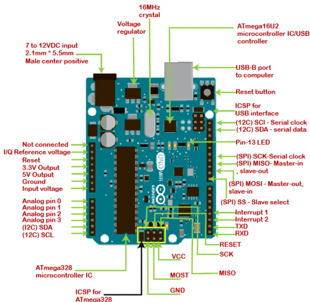
Figure 2.1 : Les spécifications de la carte ARDUINO UNO.
