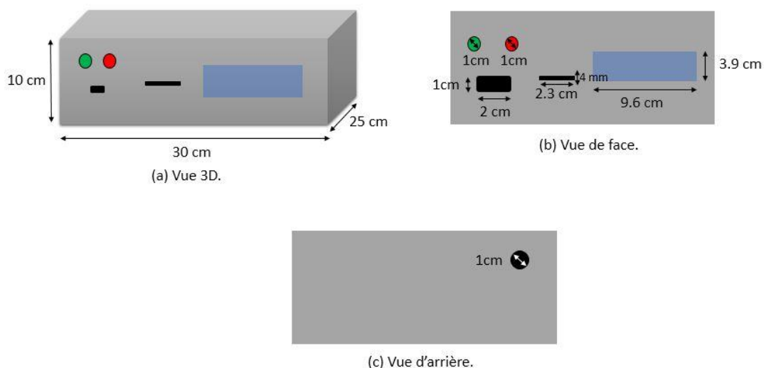
Figure 3.42 : Les dimensions de la boîte.
