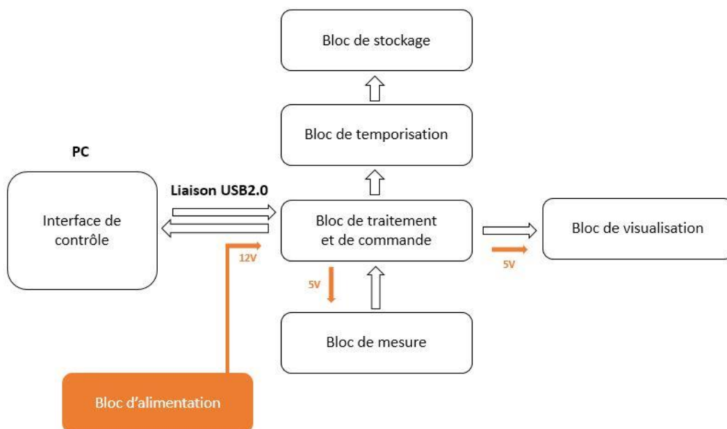
Figure 3.1 : Schéma synoptique général du projet.
