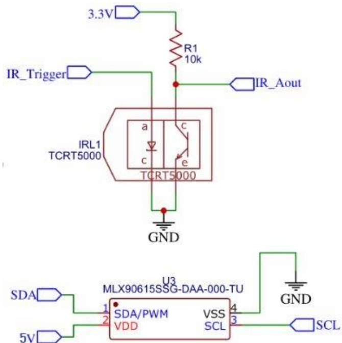
Figure 3.39 : Schéma général partie 1.
