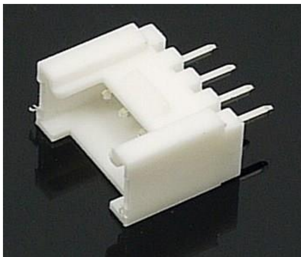
Figure 3.5 : Connecteur Grove.
