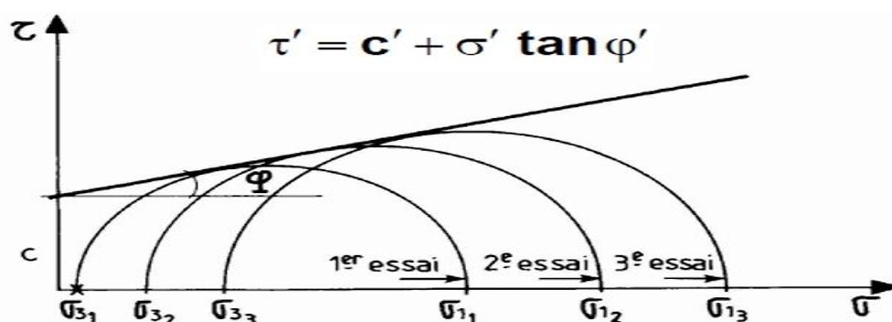
Figure 0.3: exemple des cercles de Mohr essai triaxial
