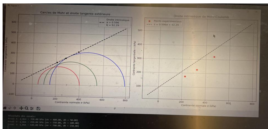
Figure 0.1 : le cercle de Mohr de Geo_Code_Lab avec le problème de point pik
