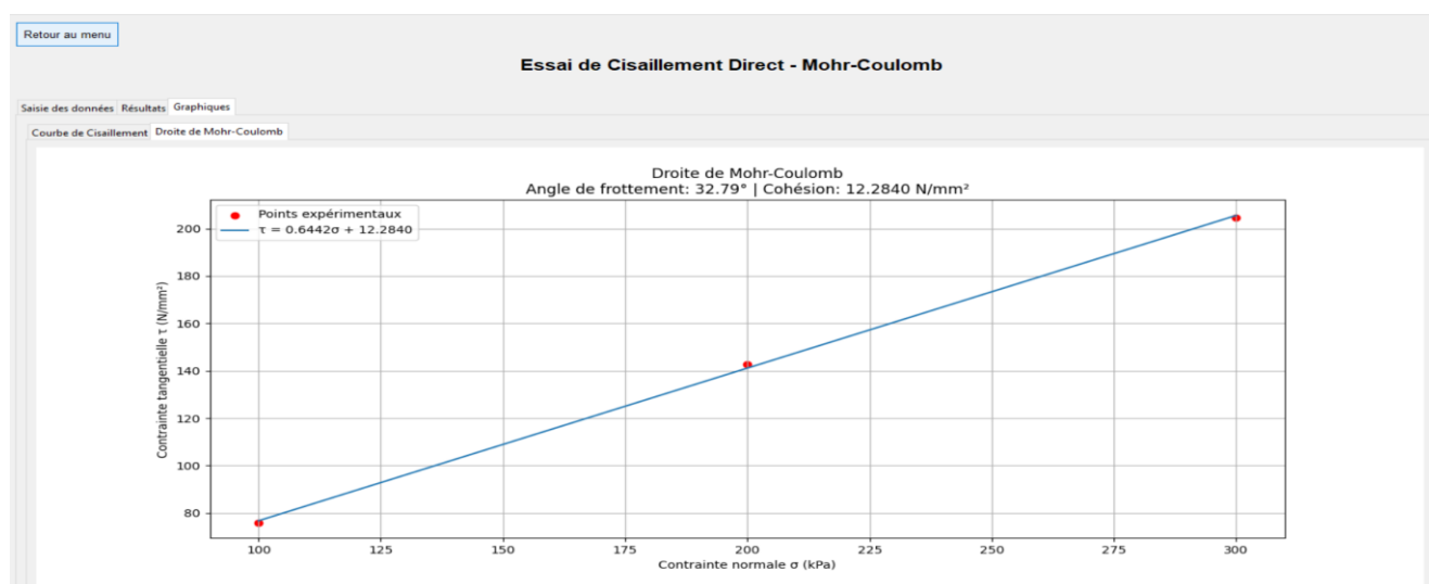
Figure 0.11: Droite de Mohr-Coulomb de l'essai cisaillement direct
