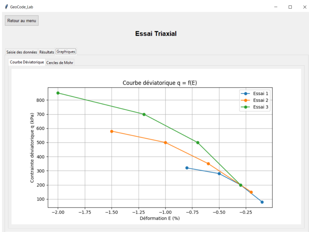
Figure 0.6: Courbe diviatorique de l'essai triaxial
