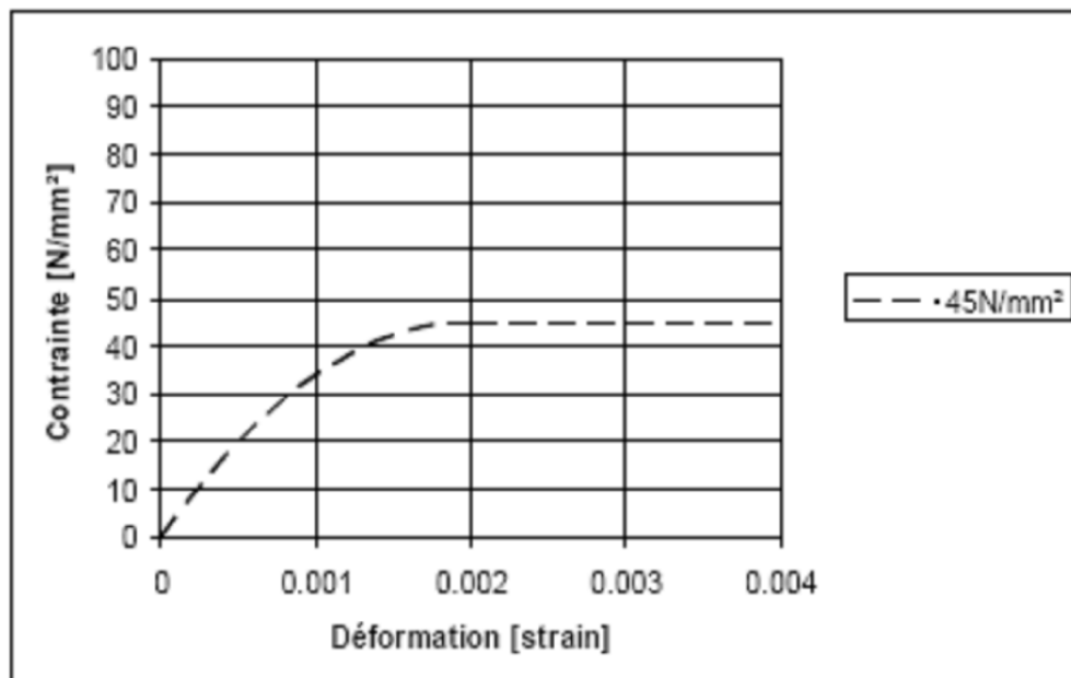
La figure 2.4 : Courbe « Parabole - Rectangle » pour un béton de résistance 45 \text{ N/mm}^2 [32].
