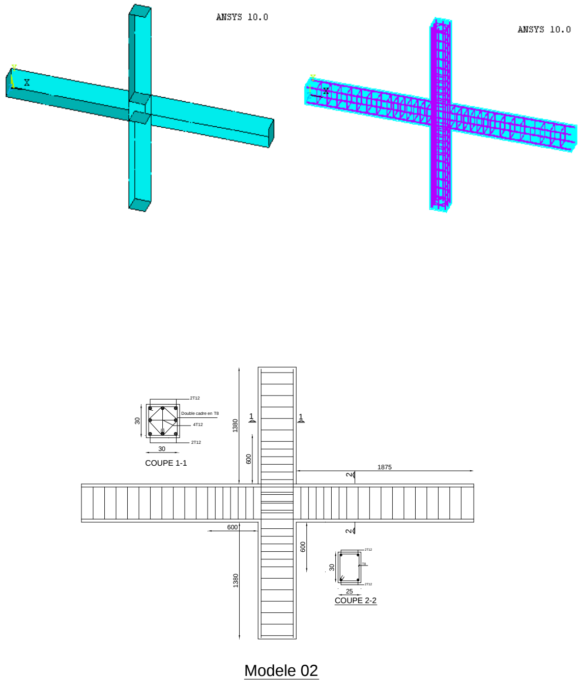
Figure (3.14) : Les dimensions typiques des nœuds avant le renforcement (NM2).
