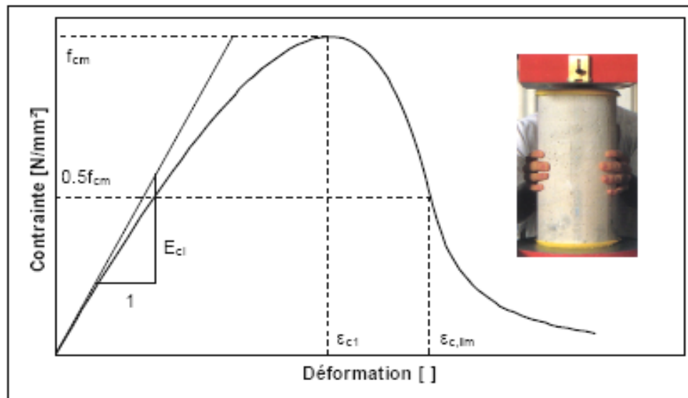
Figure 2.5 : Diagramme \sigma - \epsilon pour le béton comprimé [34].
