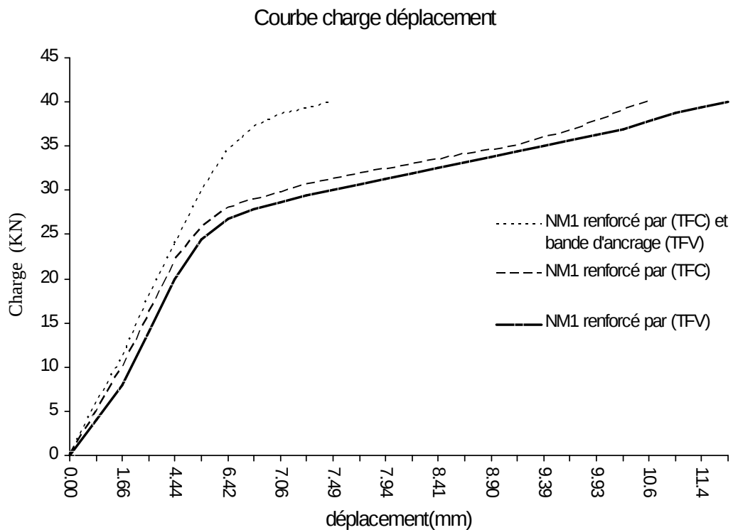
Figure (4.11) : Comportement global du nœud de référence et des nœuds renforcés par collage des bandes et tissu en forme de (L) ( F=40\text{KN} )
