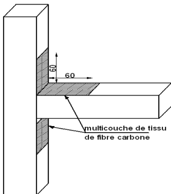
Figure (4.3) : Configuration de renforcement des nœuds par collage de tissu multicouches en fibres de carbone.
