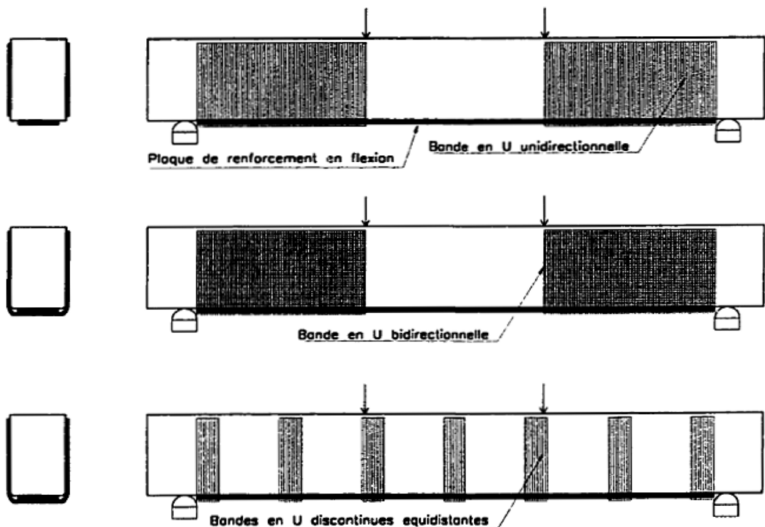
Figure 1.22 : méthode d'ancrage [17].
