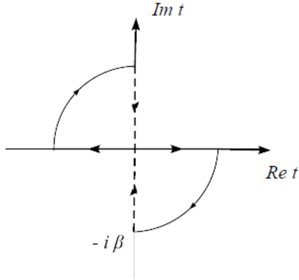
Figure 1.2 : La rotation de Wick dans l'espace des temps imaginaires.
