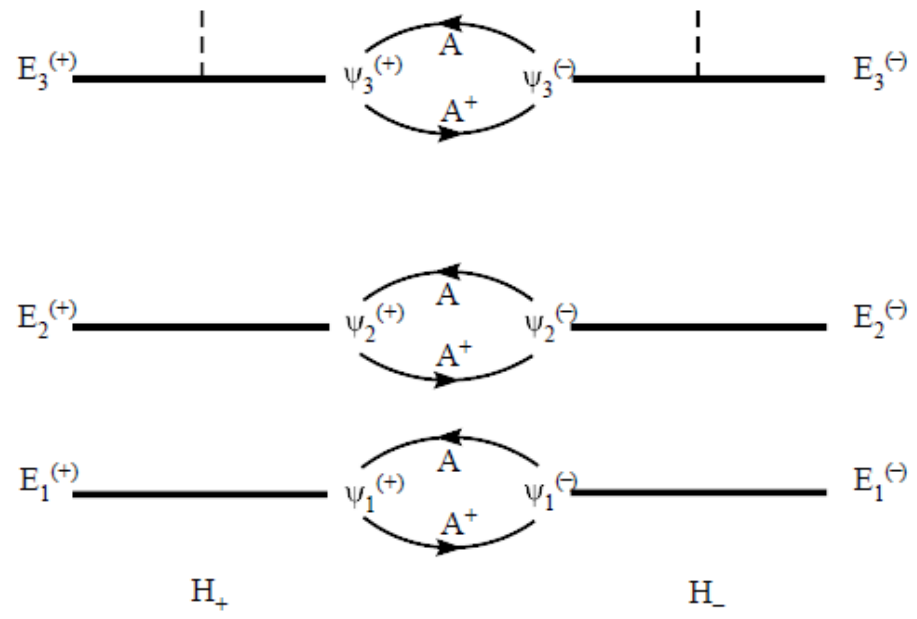
Figure 4.3 : La brisure spontanée de la supersymétrie.
