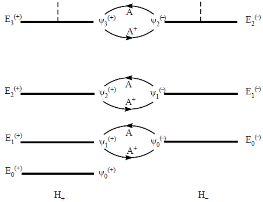
Figure 4.2 : L'action des opérateurs de création et d'annihilation sur les fonctions d'onde.
