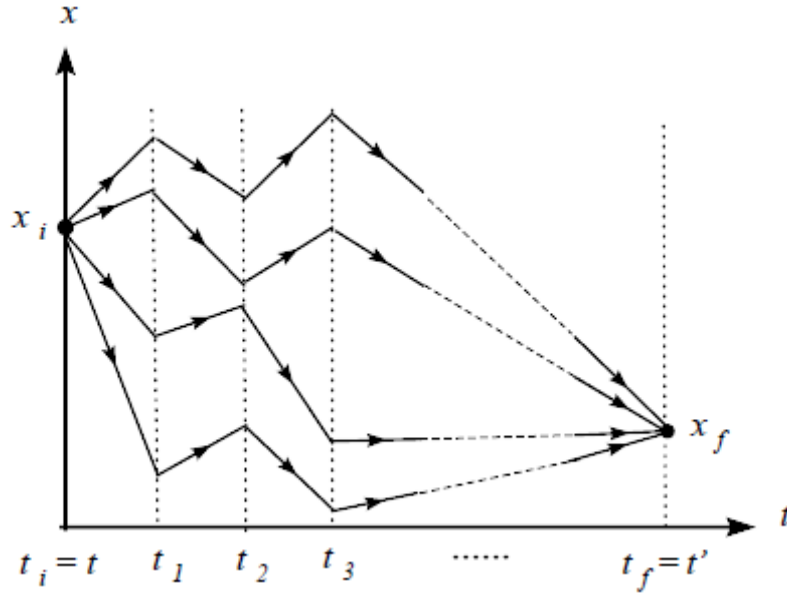
Figure 1.1 : Les trajectoires possibles entre les états initial et final.
