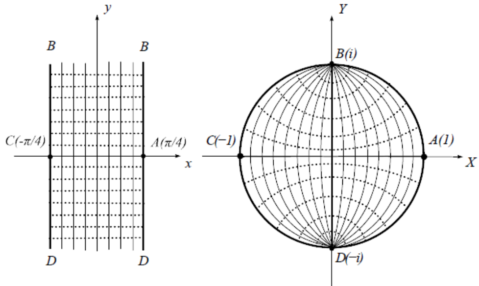
Figure B.1: Représentation conforme des familles orthogonales.
