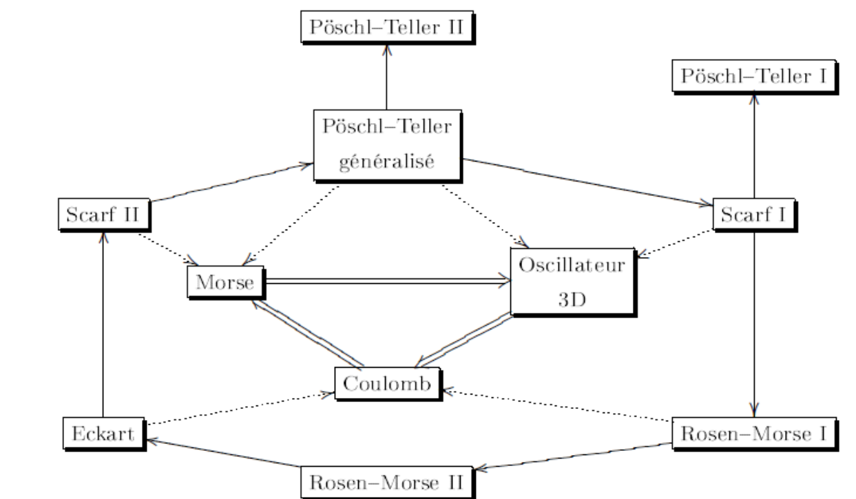
Figure 8.1 : La connexion entre les potentiels aux formes invariantes.
