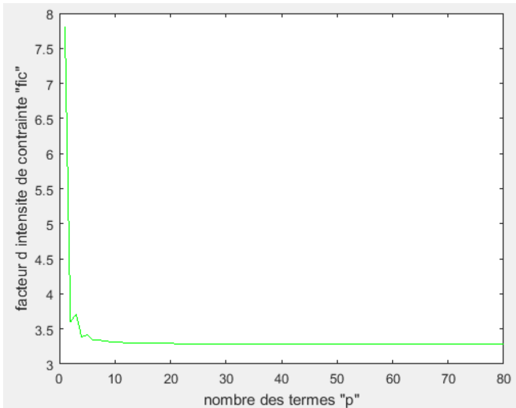
Figure A3-49 : facteur d'intensité de contrainte K_{III} en fonction de p ( f=1.5 )
