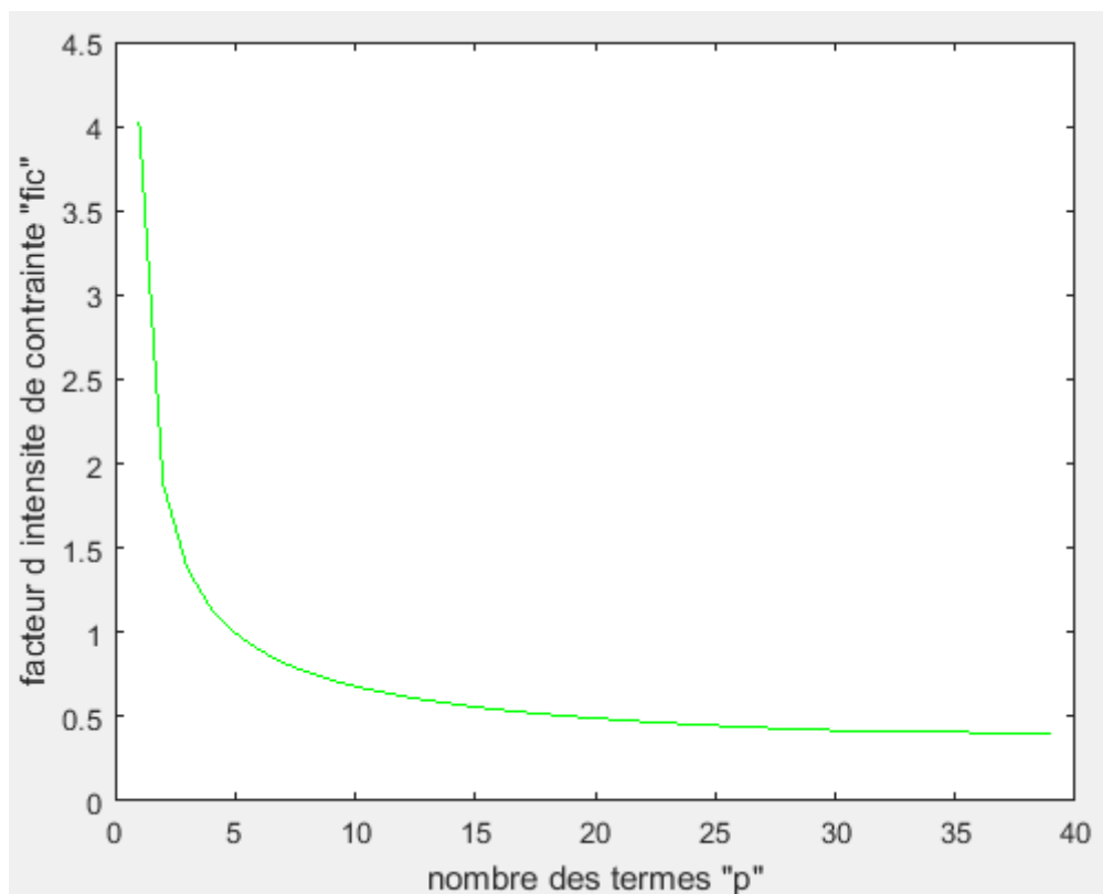
Figure A3-7 : facteur d'intensité de contrainte K_{III} en fonction de p (f=0.03)
