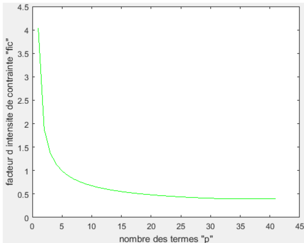
Figure A3-6 : facteur d'intensité de contrainte K_{III} en fonction de p ( f=0.025 )
