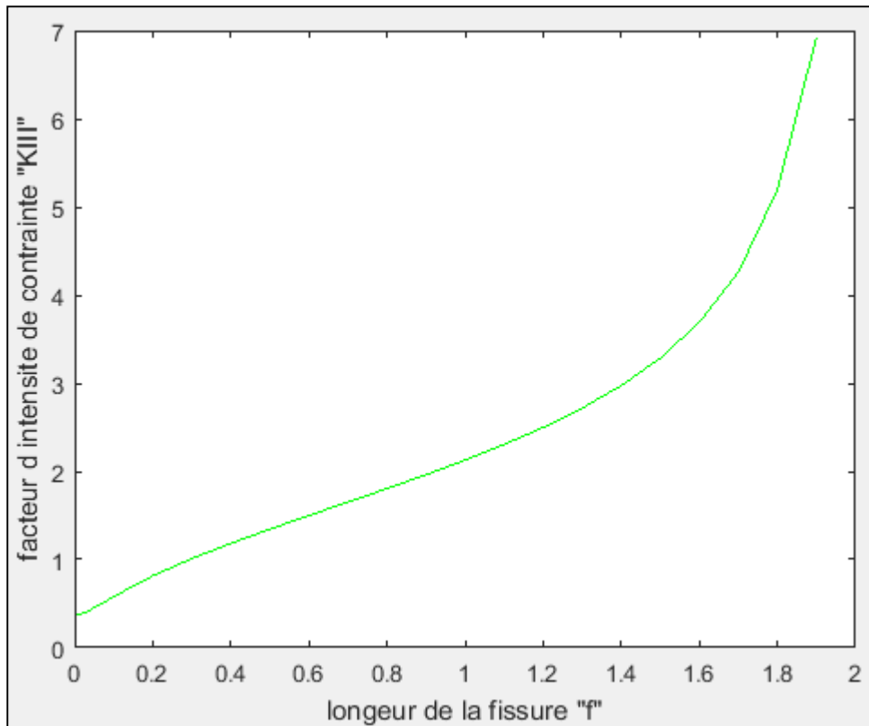
Figure III-10 : La courbe de K_{III} en fonction de f .
