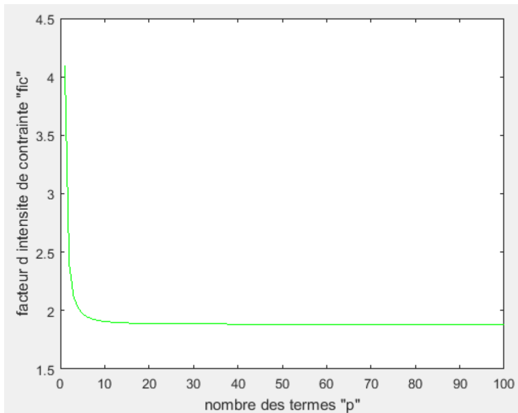
Figure A3-36 : facteur d'intensité de contrainte K_{III} en fonction de p (f=0.85)
