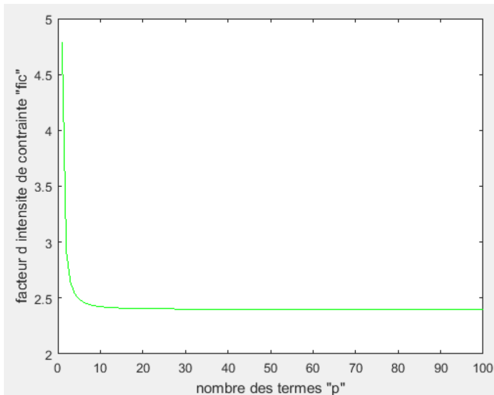
Figure A3-42 : facteur d'intensité de contrainte K_{III} en fonction de p (f=1.15)
