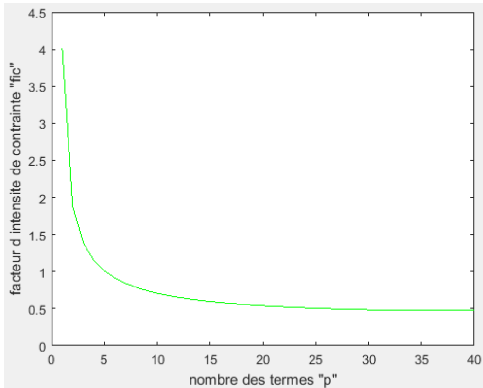
Figure A3-13 : facteur d'intensité de contrainte K_{III} en fonction de p ( f=0.06 )
