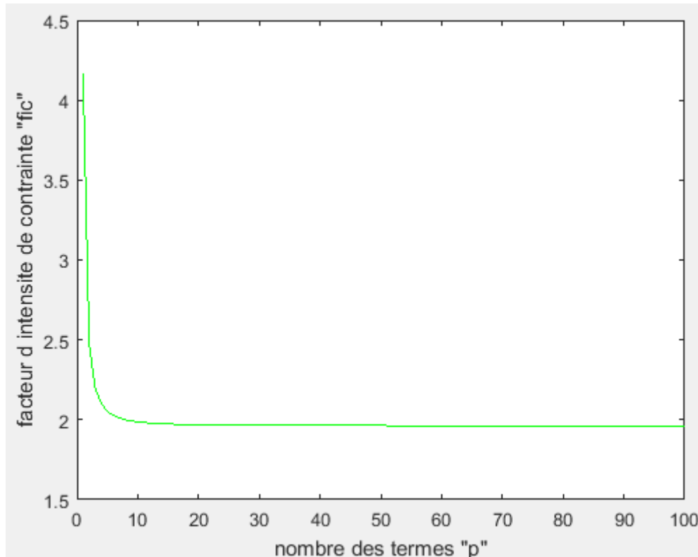
Figure A3-37 : facteur d'intensité de contrainte K_{III} en fonction de p (f=0.9)
