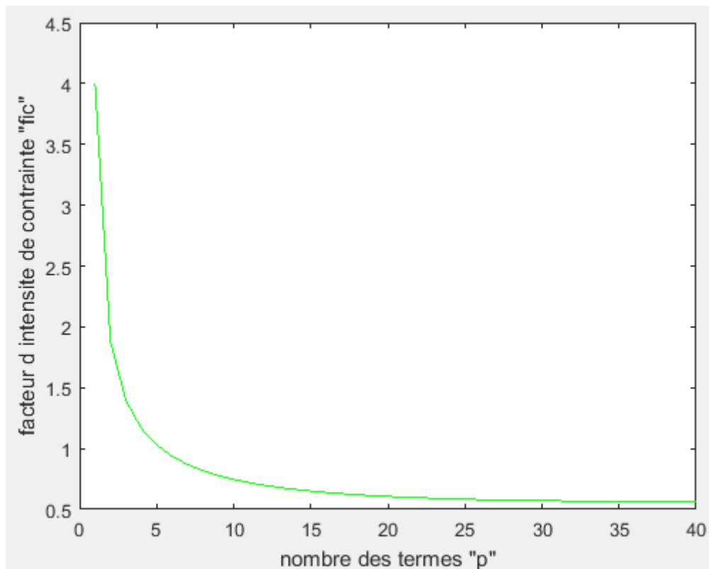
Figure A3-20 : facteur d'intensité de contrainte K_{III} en fonction de p (f=0.095)
