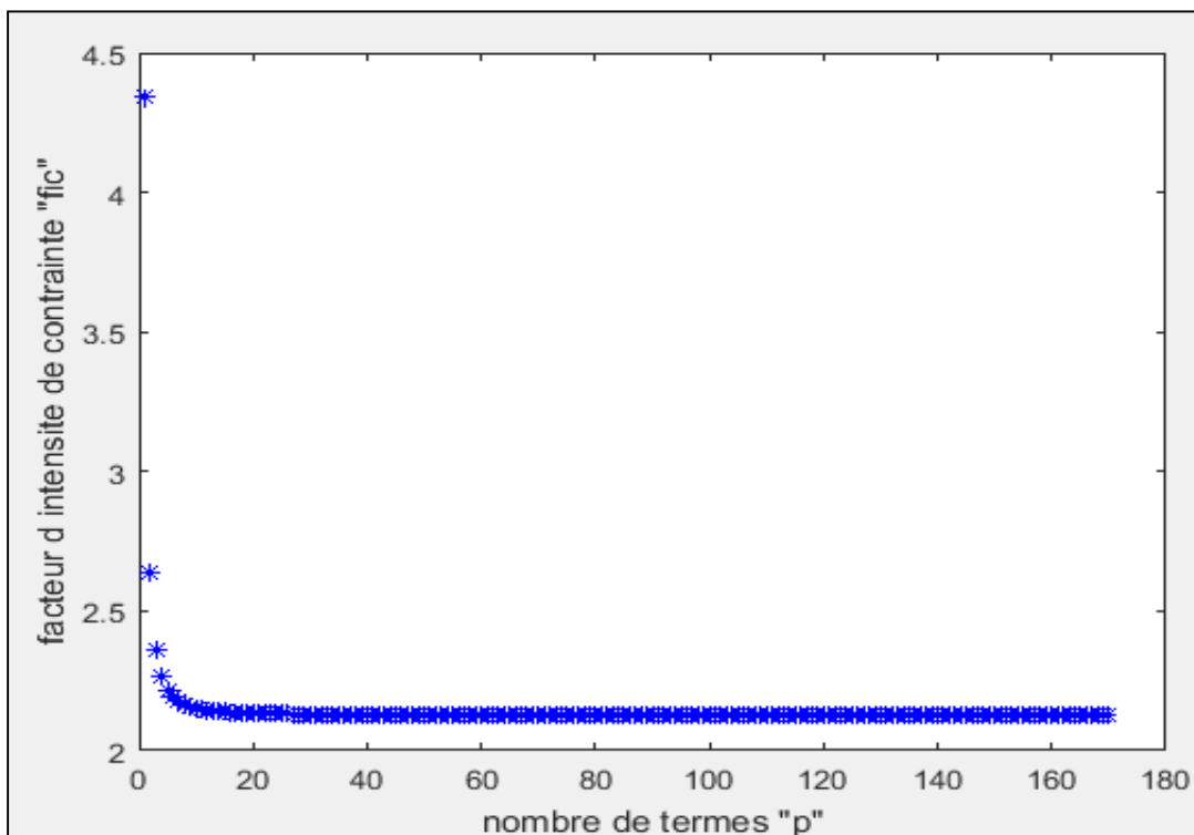
Figure III-3 : K_{III} en fonction de nombre des points de collocation p pour une fissure centrale dans une section circulaire [10].
