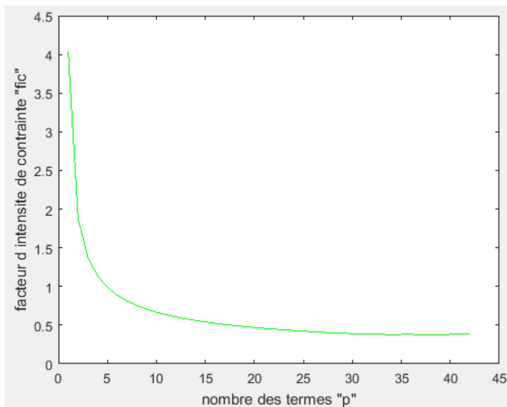
Figure A3-4 : facteur d'intensité de contrainte K_{III} en fonction de p (f=0.015)
