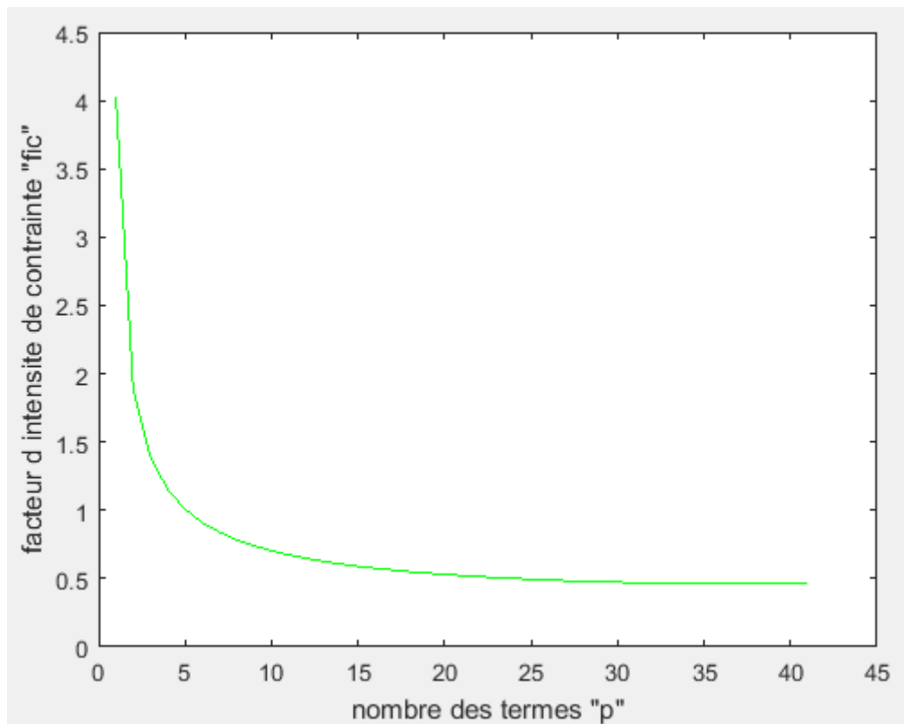
Figure A3-12 : facteur d'intensité de contrainte K_{III} en fonction de p ( f=0.055 )
