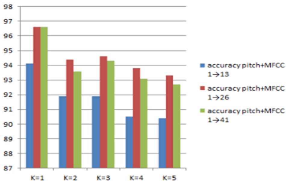
Figure 3.11 : Histogramme des acuuracy avec 13, 26 et 41 MFCC + pitch.
