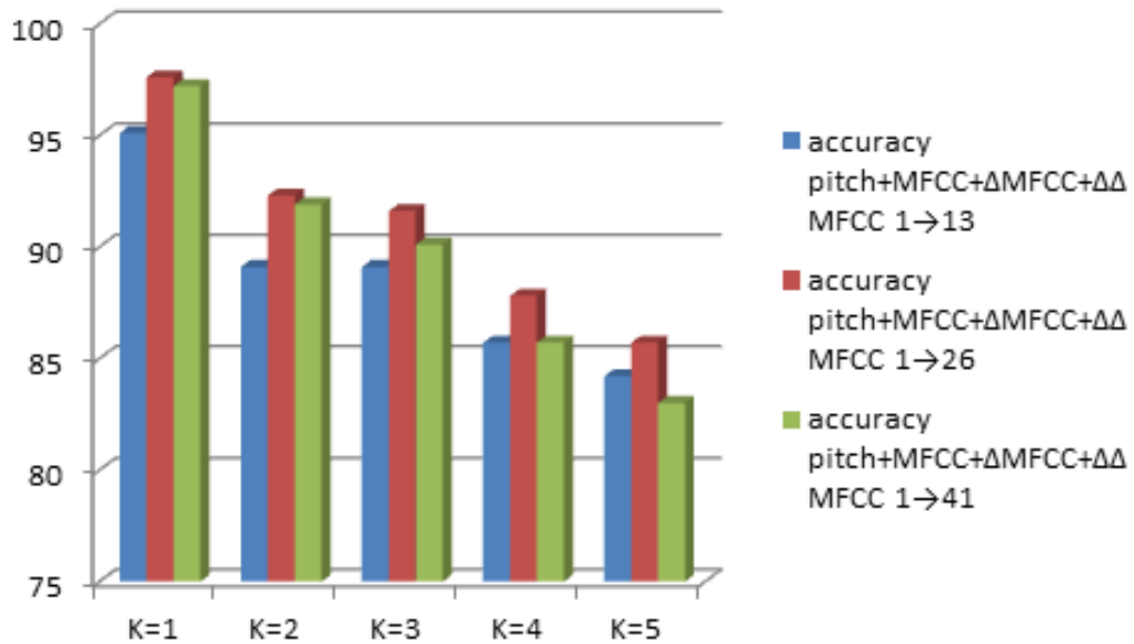
Figure 3.15 : Histogramme des accuracy avec 13, 26, 41 (MFCC+ \Delta\Delta MFCC+ \Delta MFCC)+ pitch.
