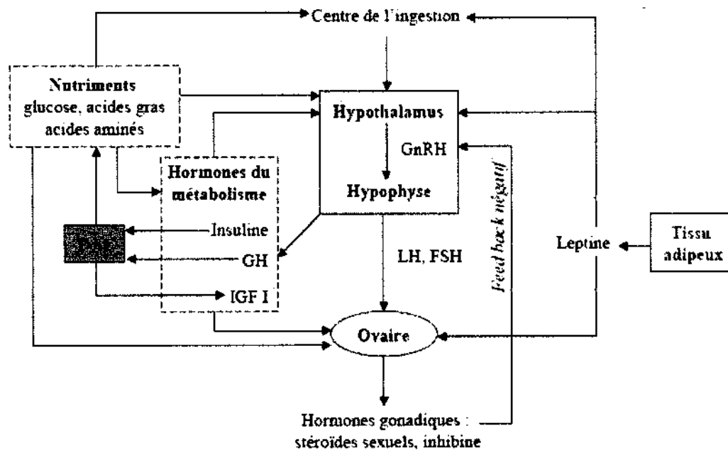
Figure 7 : Principaux mécanismes physiologiques impliqués dans les effets de la nutrition sur la reproduction (Fortun-Lamothe, 2003)
