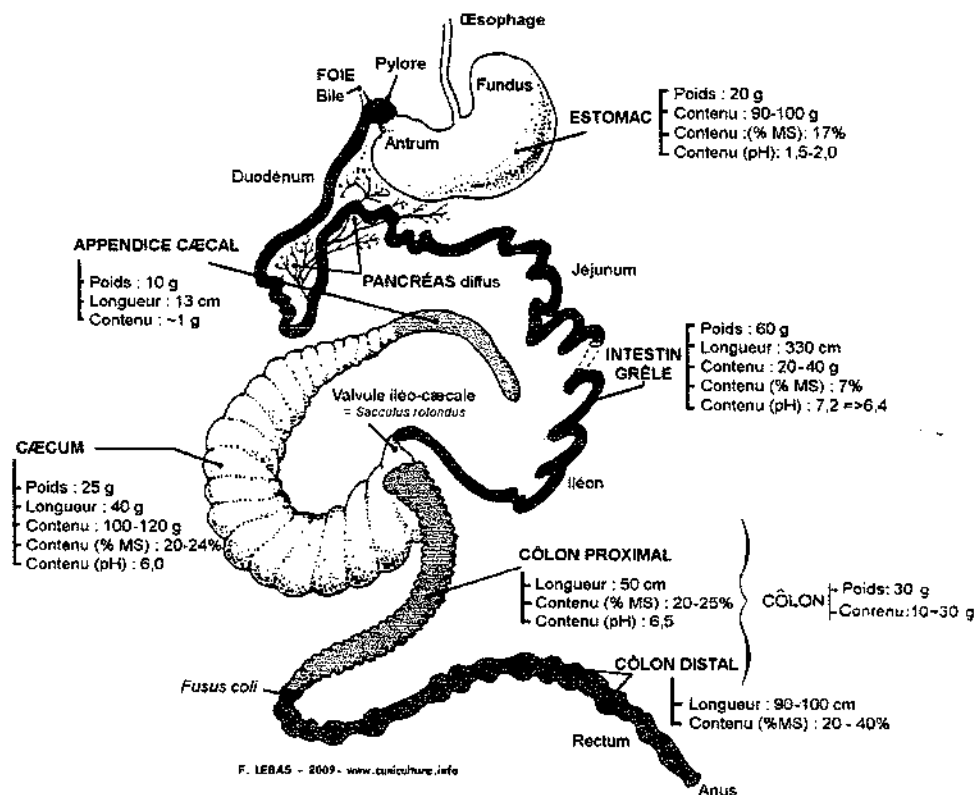
Figure 5 : Anatomie générale du tube digestif du lapin (Lebas, 2011).
