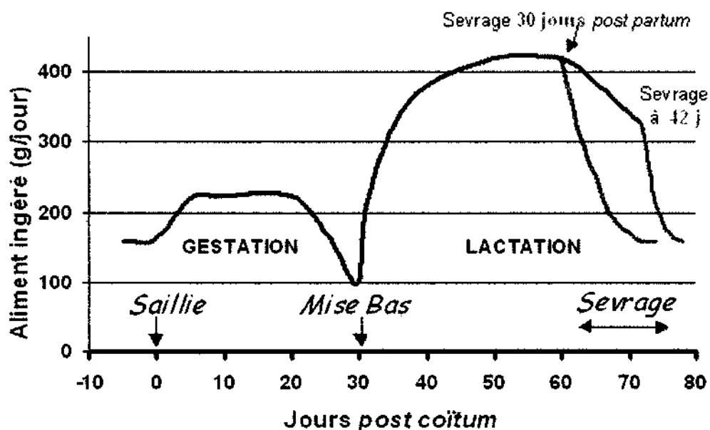
Figure 9 : Évolution de la consommation d'aliment complet équilibré par une lapine au cours d'un cycle de reproduction (Lebas, 2011)
