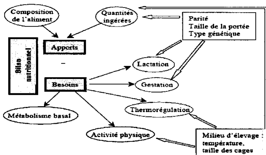
Figure 8 : Bilan énergétique des lapines et facteurs de variation
