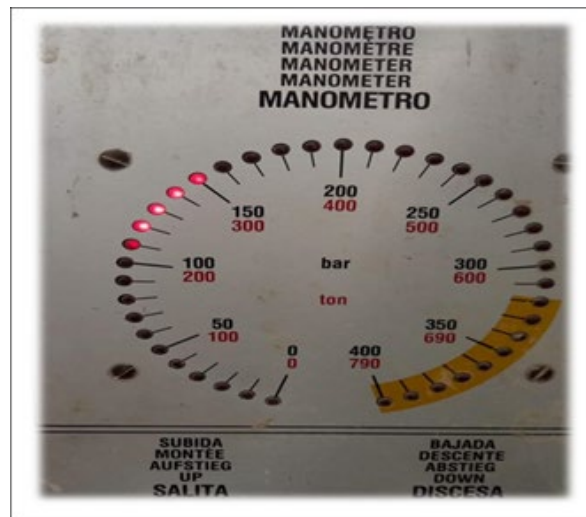
Figure IV.2 : Photo numérique montre révision la valeur de pression sur format de carreaux céramiques 8 × 45 (cm)
