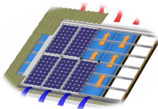
Figure II.10 : Mode d'intégration du capteur sur une partie d'une toiture en pente
