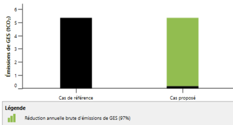
Figure IV.7 : Réductions émissions GES (Batna).
