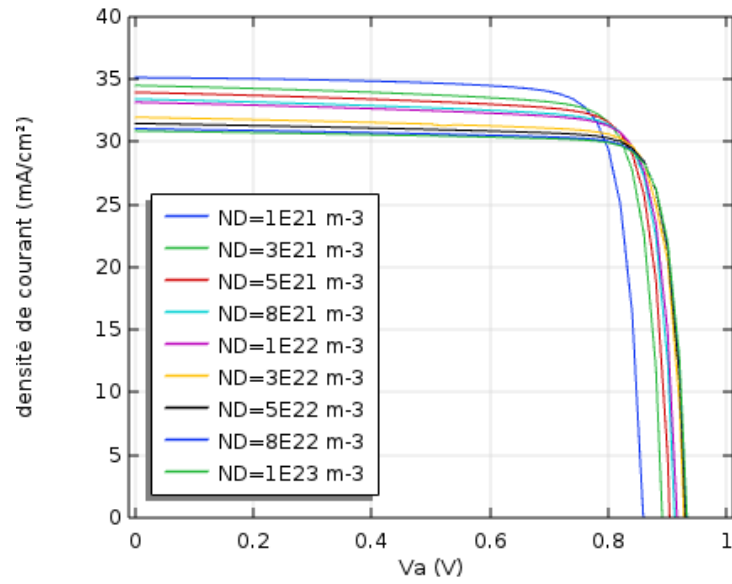
Figure 3.6. Caractéristiques courant-tension pour différentes valeurs de ND de la couche GaAs
