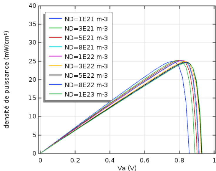
Figure 3.7. Caractéristiques puissance/ tension pour différentes valeurs de ND de la couche Ga
