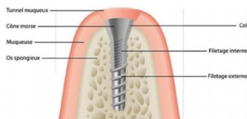
Figure 97 : schéma d'un implant ostéo-intégration
