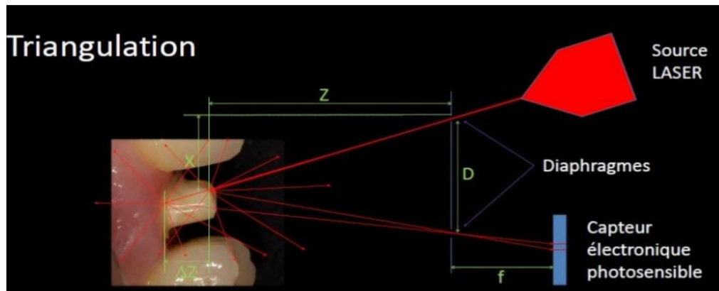
Figure 125 : principe de l'imagerie par triangulation
