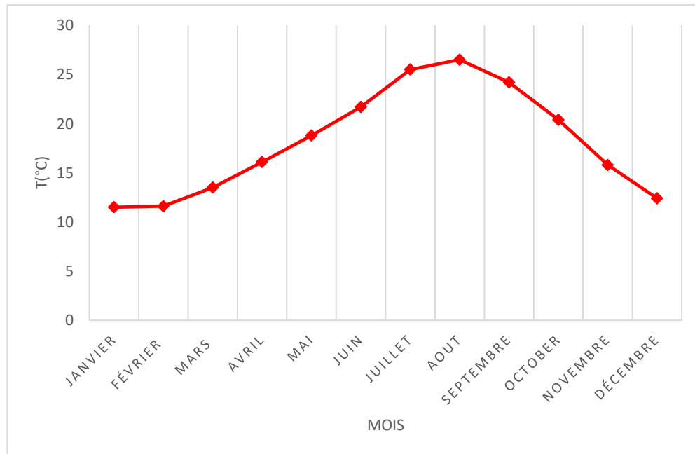
Figure 08: Courbe des températures mensuelles moyennes de la région de Bejaïa (2008/2017).
