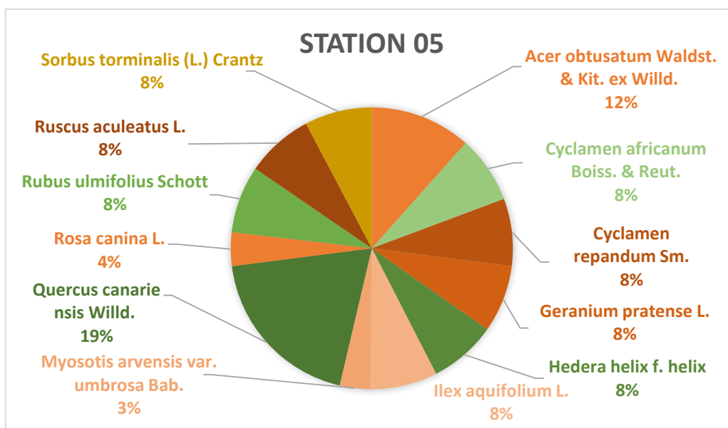
Figure 27 : Spectre des contributions spécifiques de la station 05
