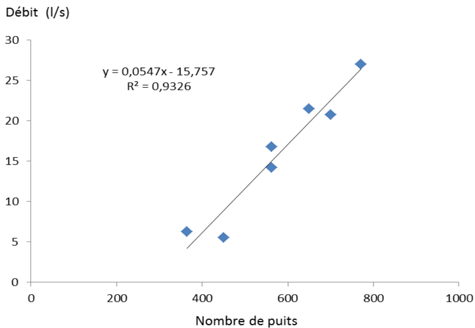
Fig. 3.8. Corrélation débit – Nombre de puits
