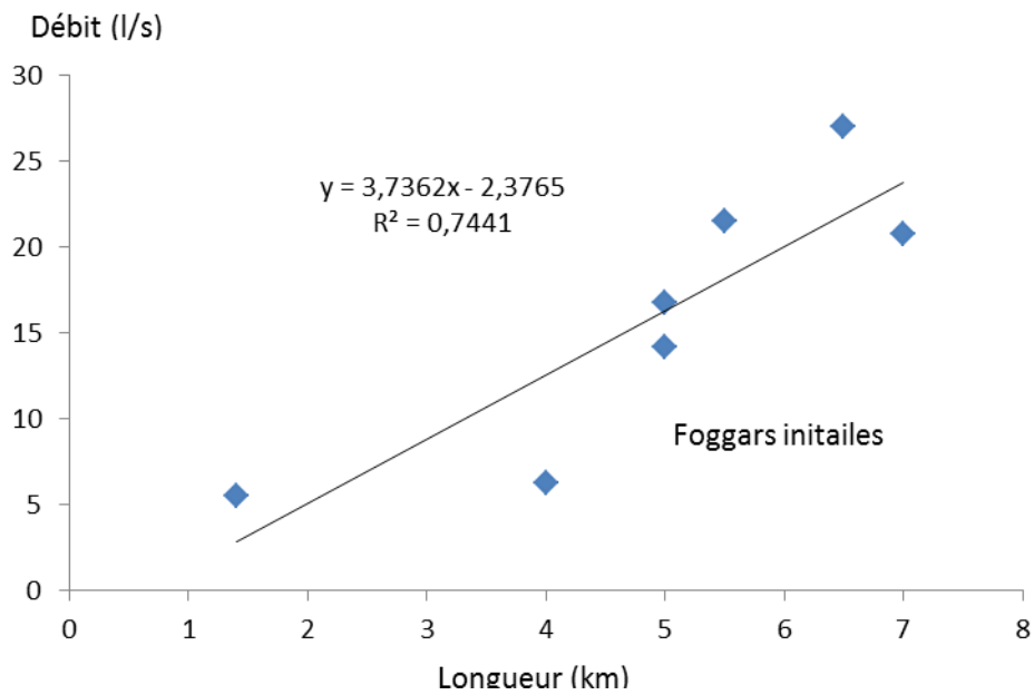
Fig. 3.7. Corrélation débit – galerie de la foggara (foggaras initiales)
