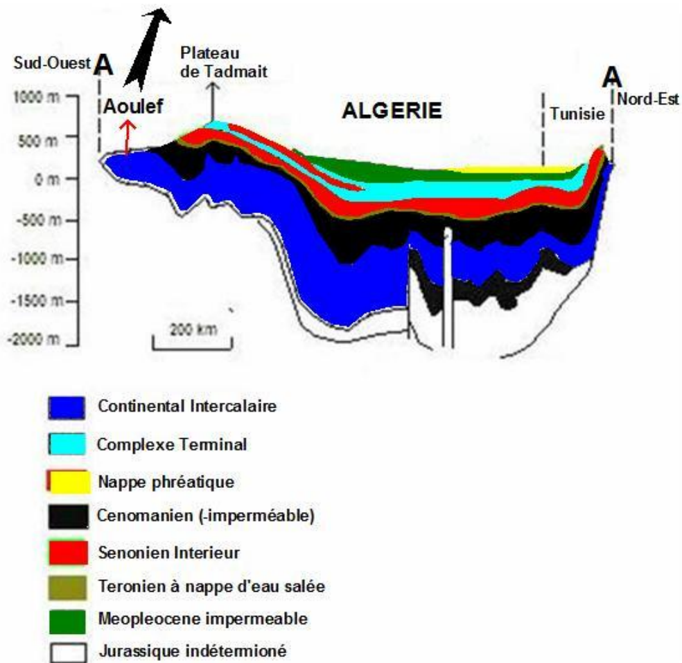
b) Coupe longitudinale de la nappe du Continental Interrcalaire (REMINI.B 2014)
