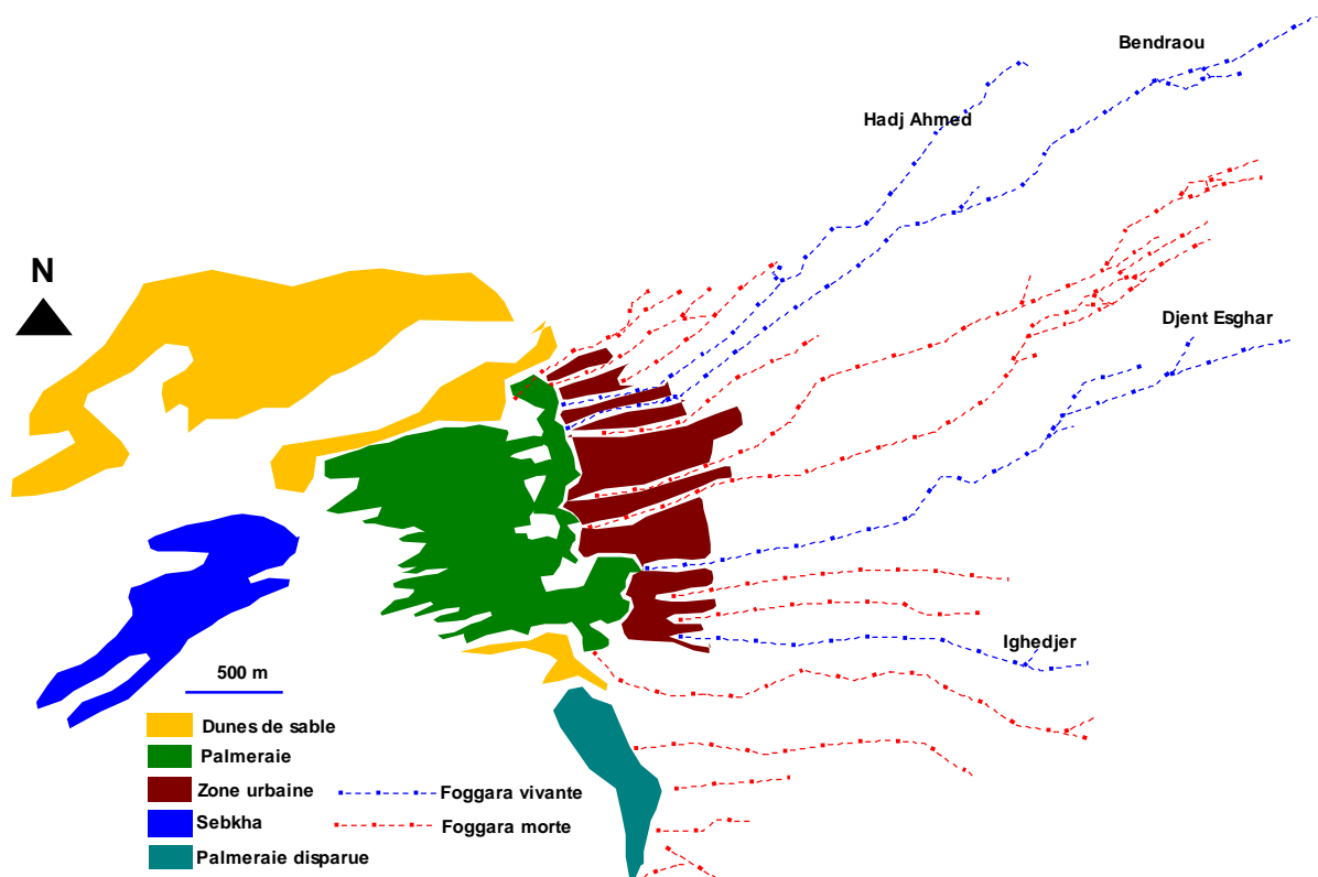
Fig. 3.3. Foggaras de l'oasis d'Arab en 2011 (REMINI.B 2014)
