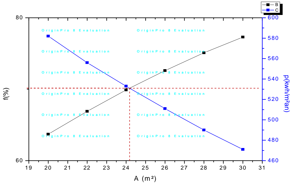
figure 4.2 : variation de productivité annuelle et de taux de couverture solaire en fonction de la surface dans le site de Alger et pour un système de ballon extérieur et échangeur noyé
