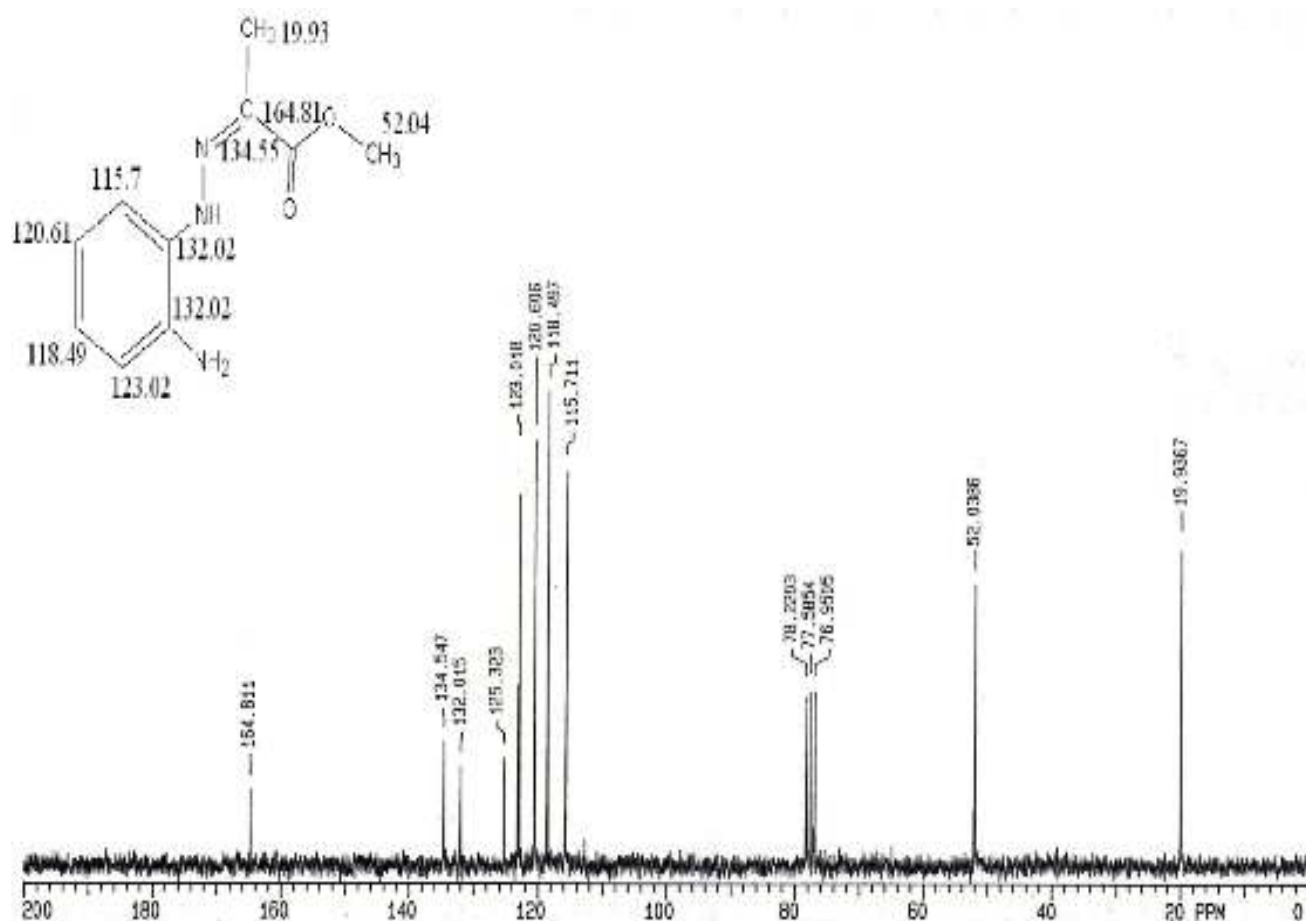
Figure 13 : Spectre 1 H-RMN de (Z)-2-aminophénylhydrzono pyruvate de méthyle
