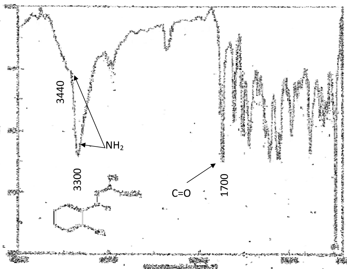
Figure 11 : Spectre IR (Z)-2-aminophénylhydrzono pyruvate de méthyle
