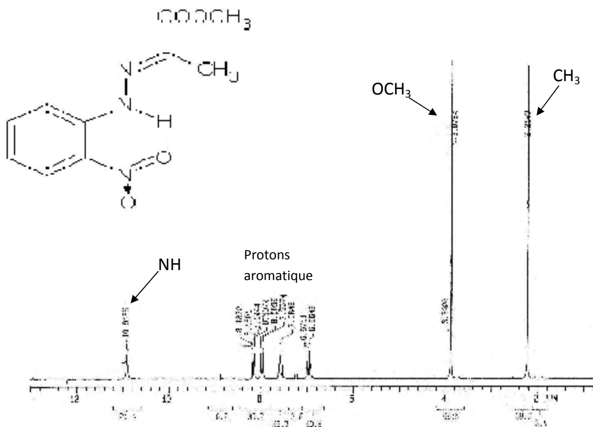
Figure 2 : Spectre ^1\text{H} -RMN de (E)-2-nitrophénylhydrazono pyruvate de méthyle
