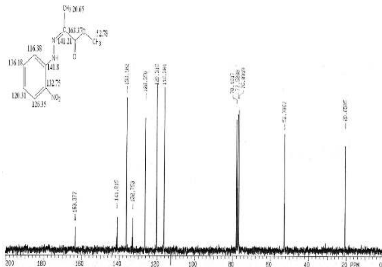
Figure 5 : Spectre ^{13}\text{C} -RMN de (Z)-2-nitrophénylhydrazone pyruvate de méthyle
