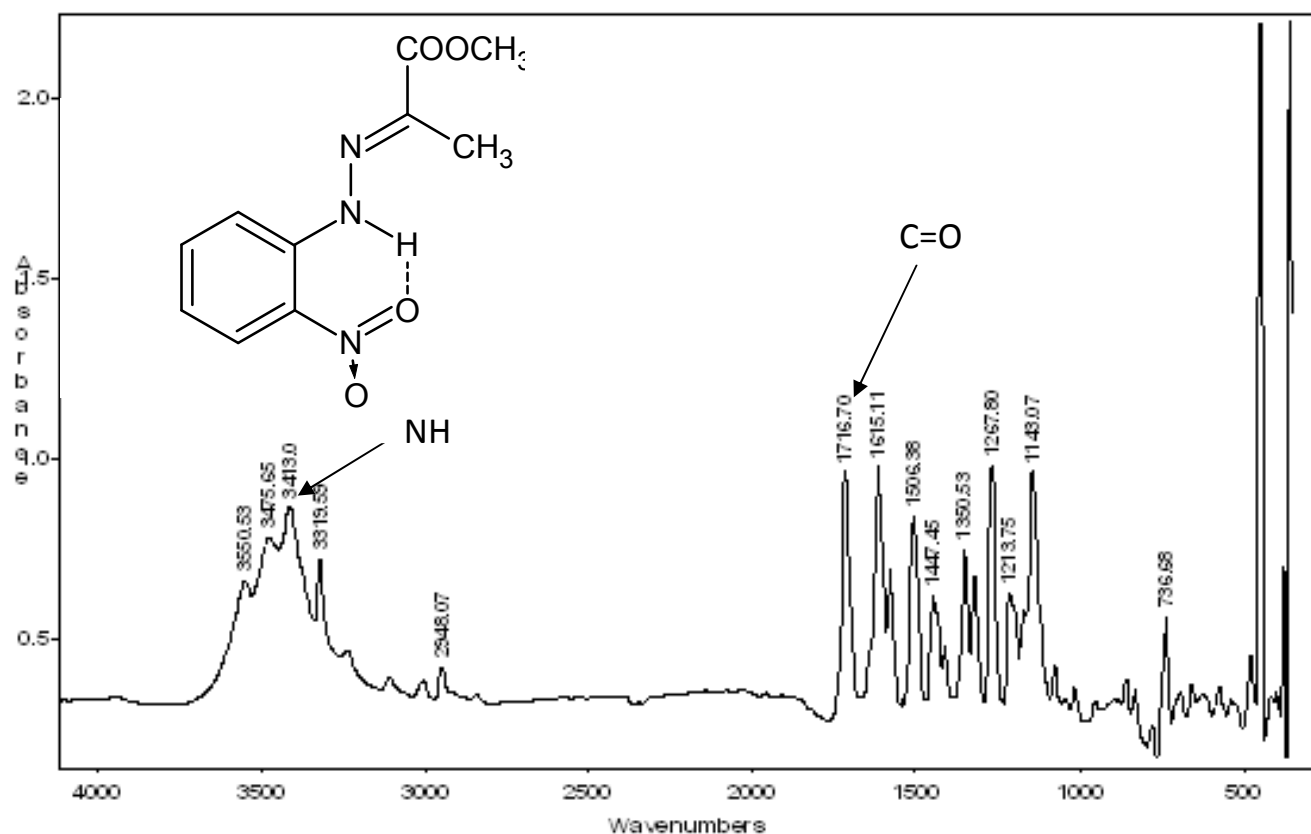
Figure 6 : Spectre IR de (E)-2-nitrophénylhydrazone pyruvate de méthyle
