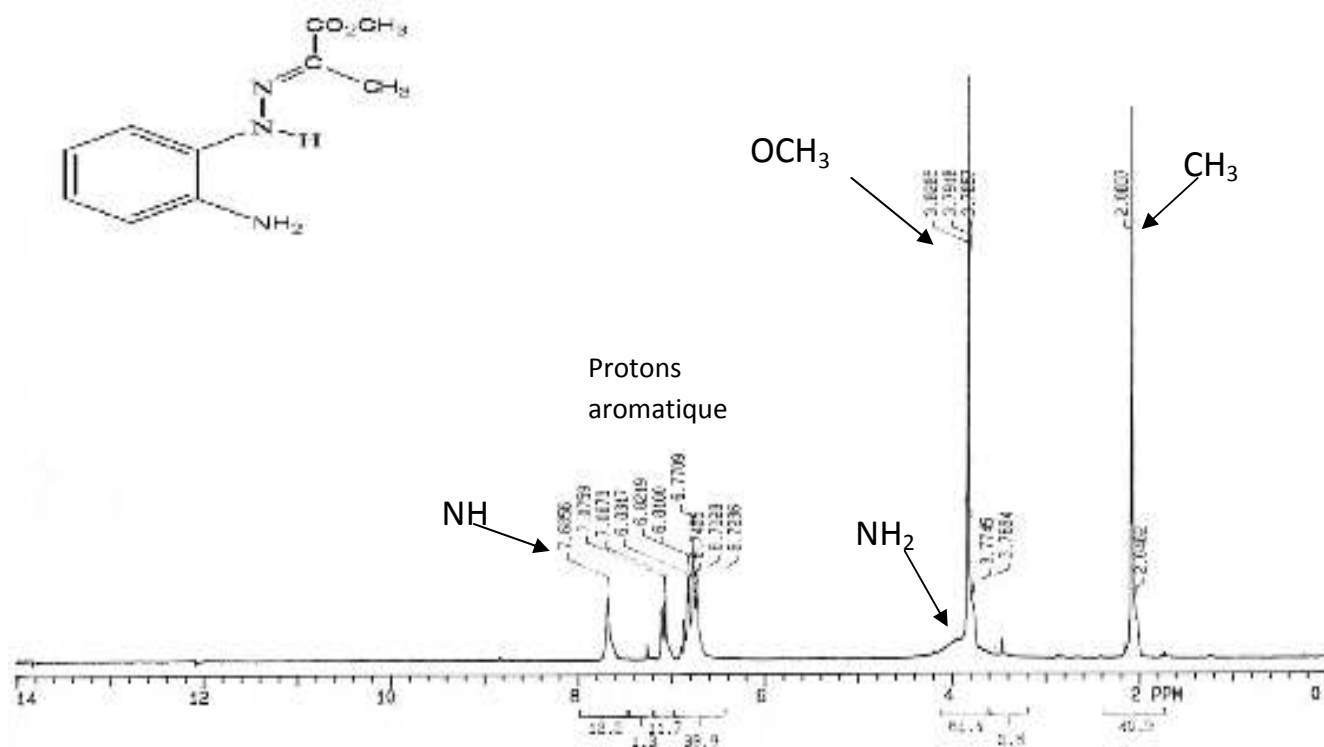
Figure 9 : Spectre ^1\text{H} -RMN de 2-aminophénylhydrzono pyruvate de méthyle
