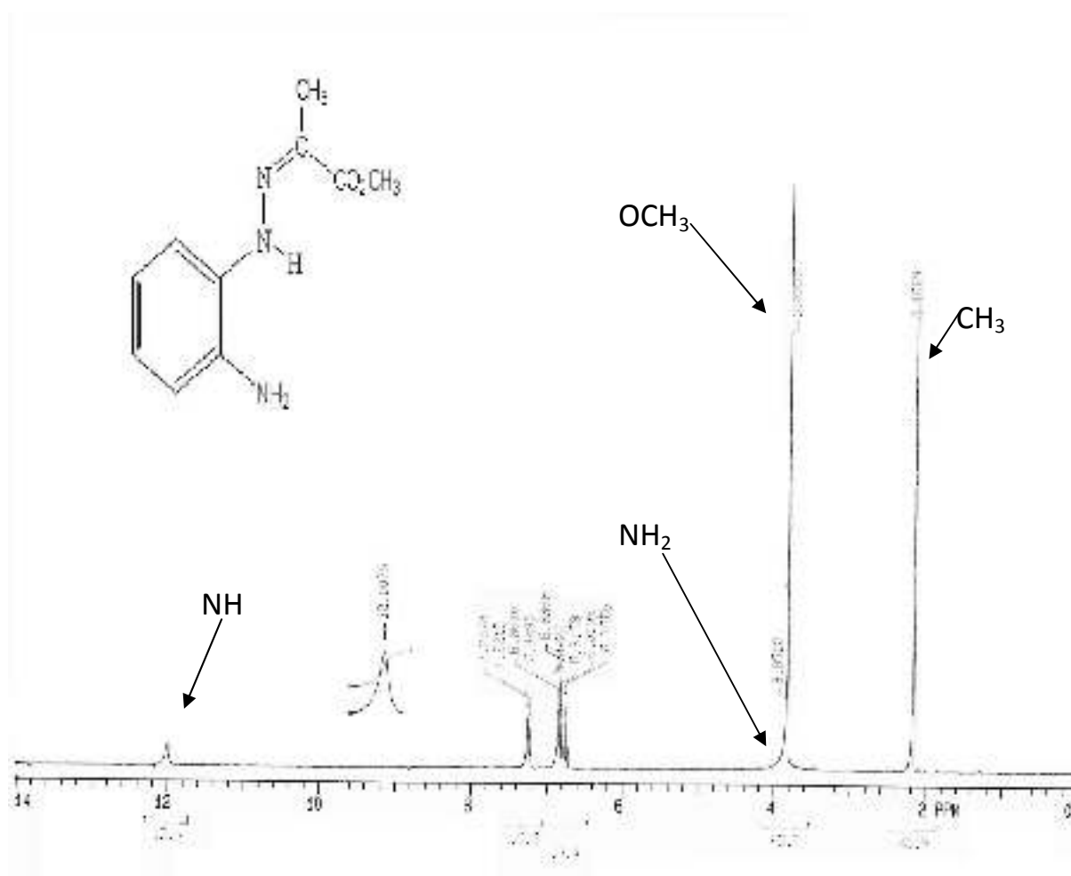
Figure 12 : Spectre ^1\text{H} -RMN de (Z)-2-aminophénylhydrzono pyruvate de méthyle
