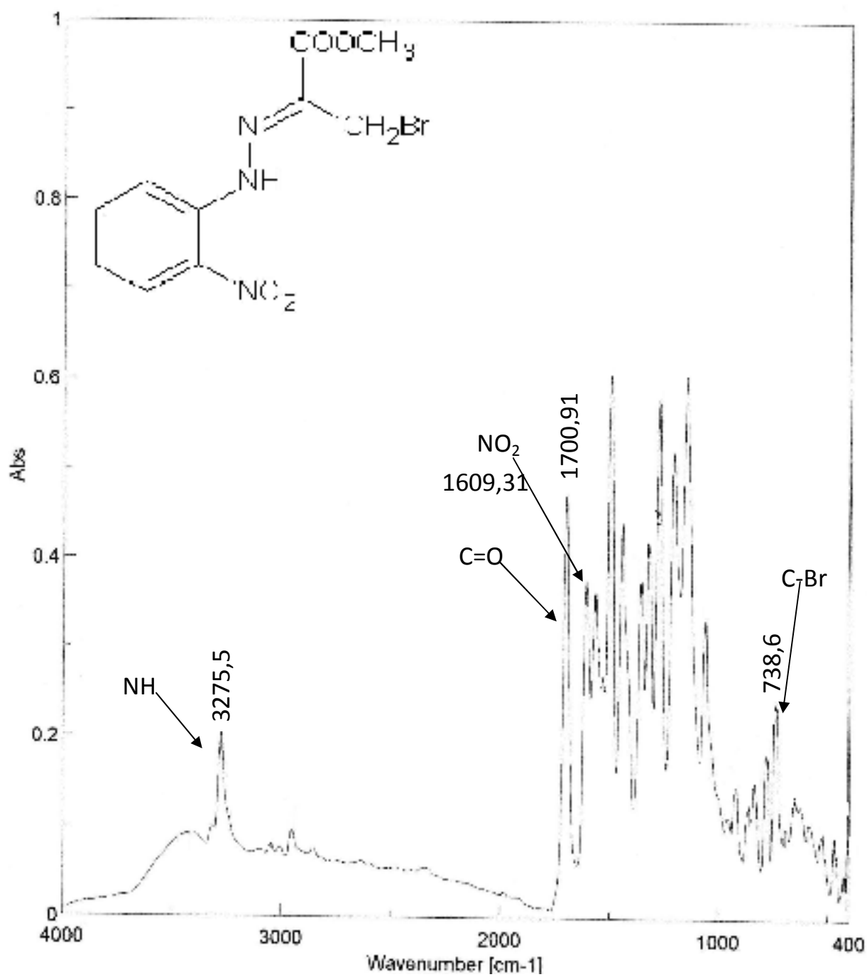
Figure 17 : Spectre IR de (E)-3-bromo-2-(2'-nitrophenyl)hydrazone propanoate de méthyle
