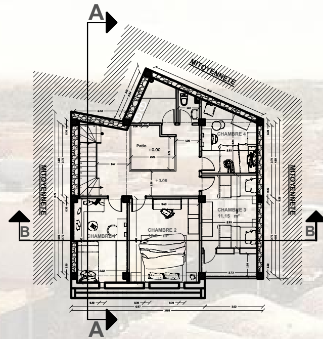
PLAN 1er ETAGE
