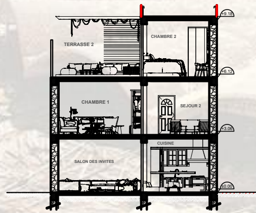
COUPE AA
