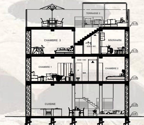
COUPE BB
