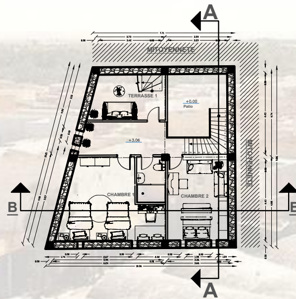
PLAN 1er ETAGE
