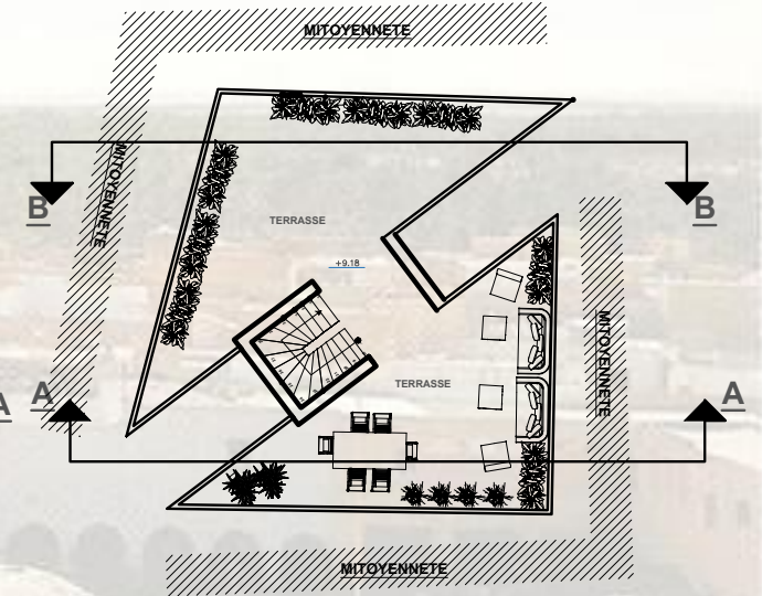
PLAN TERRASSE
