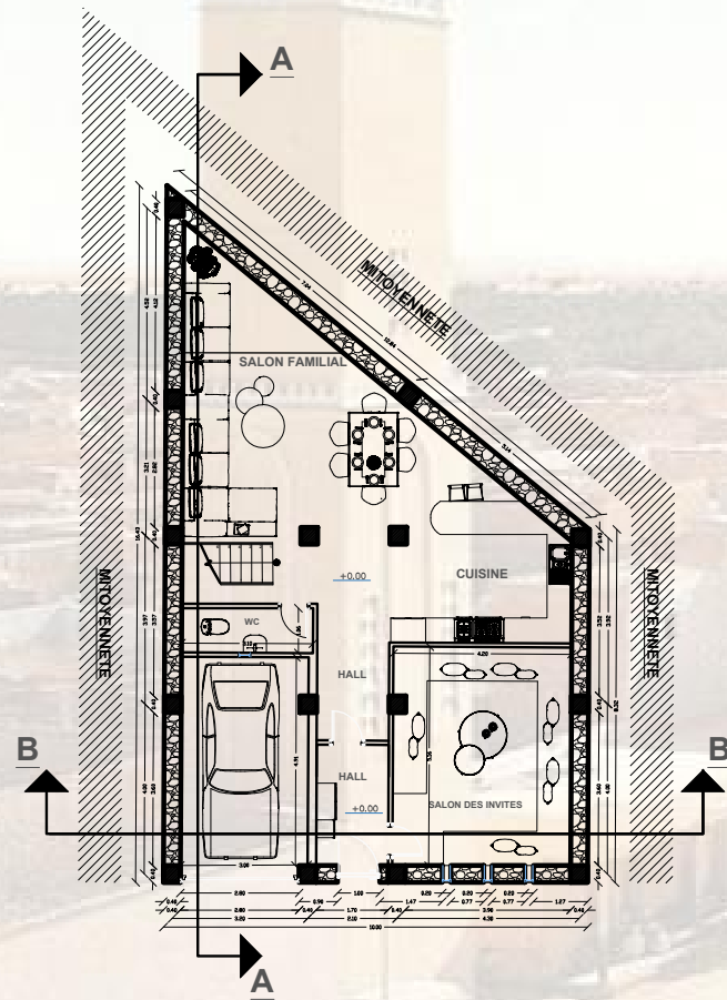
PLAN REZ DE CHAUSSEE
