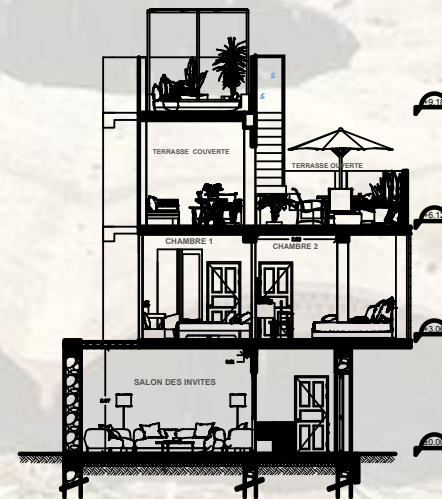
COUPE AA
