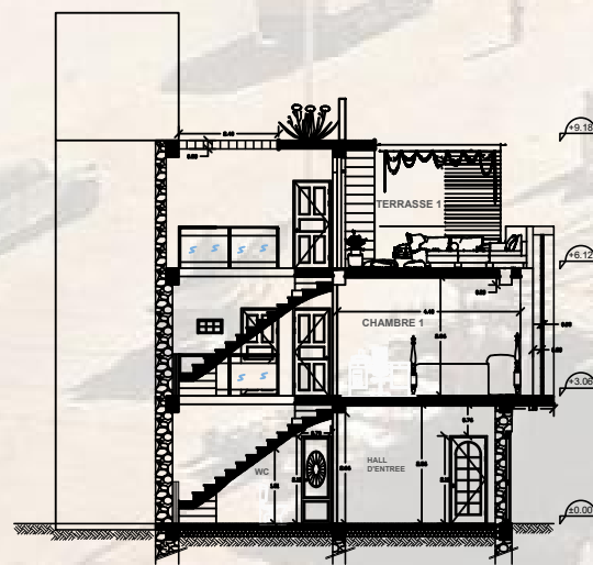
COUPE AA
