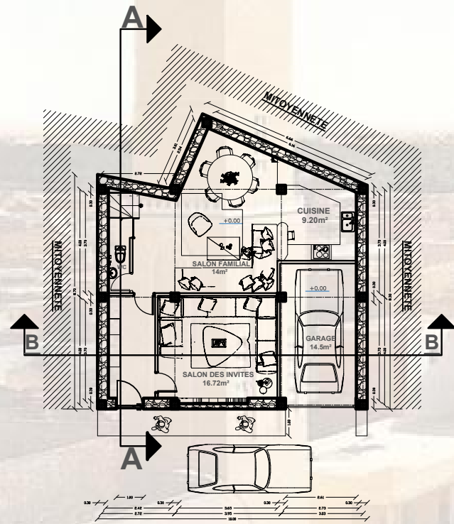
PLAN REZ DE CHAUSSE
