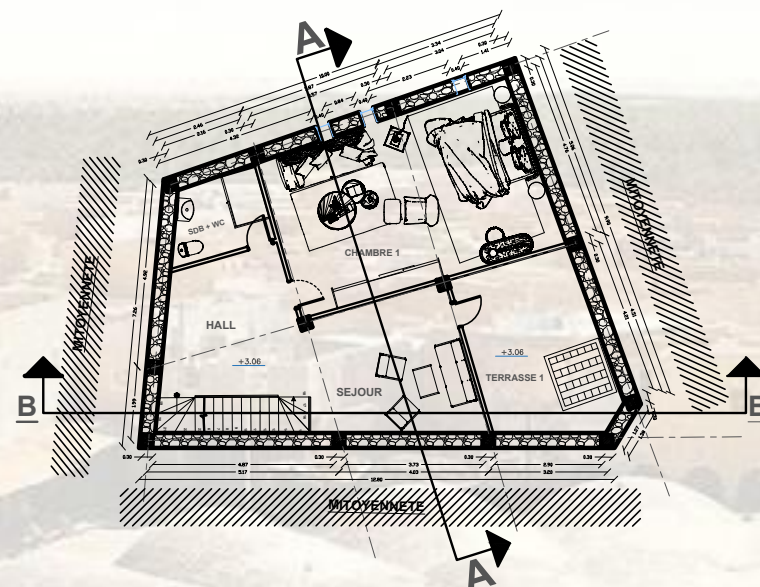
PLAN 1er ETAGE
