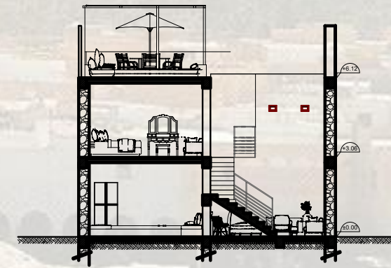
COUPE AA
