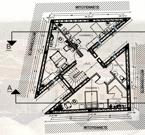
PLAN 2eme ETAGE
