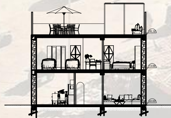
COUPE BB
