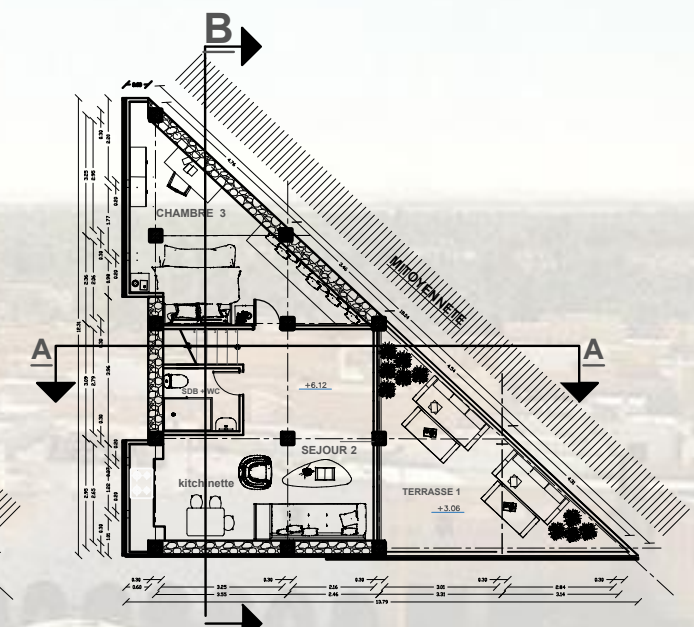
PLAN 2eme ETAGE
