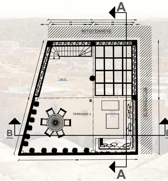
PLAN TERRASSE
