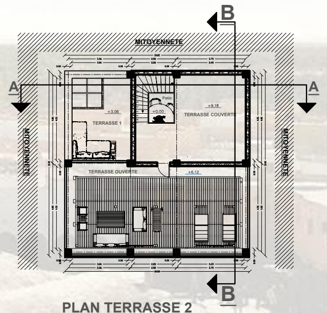
PLAN TERRASSE 2
