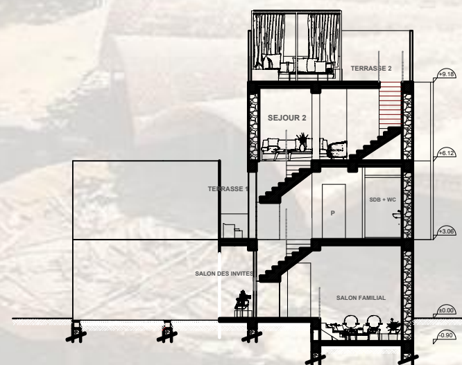
COUPE AA
