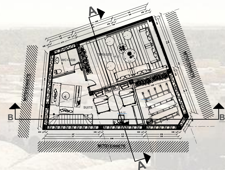
PLAN 2eme ETAGE
