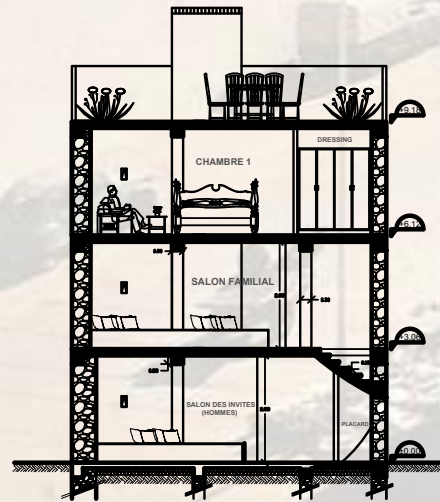
COUPE AA
