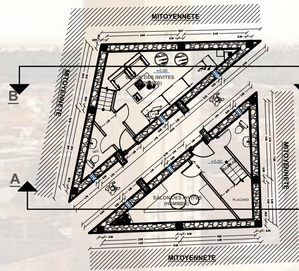
PLAN REZ DE CHAUSSEE
