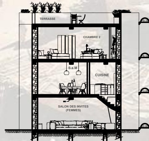
COUPE BB
