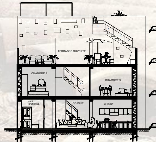
COUPE BB
