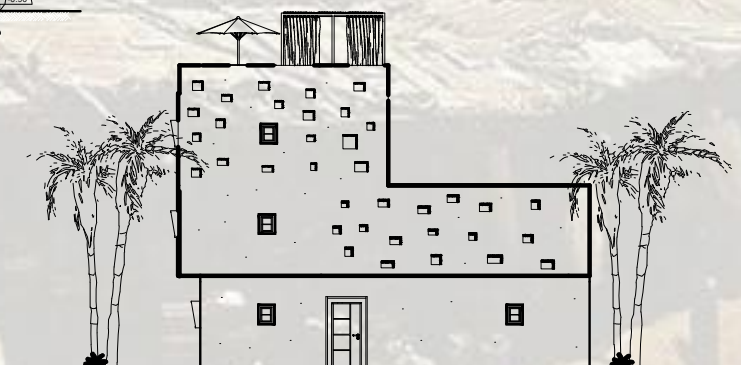
FACADE DROITE
