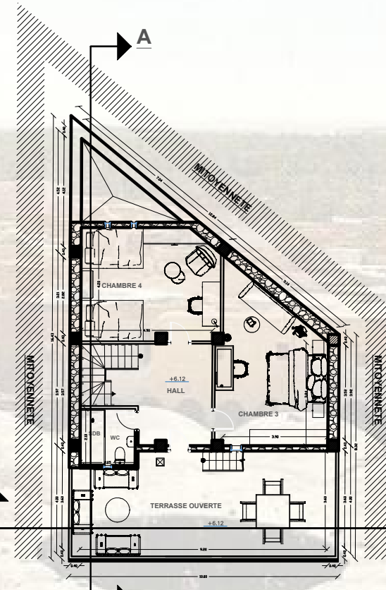
PLAN 2eme ETAGE
