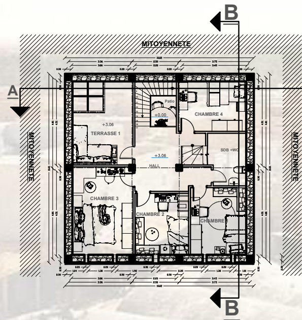
PLAN 1er ETAGE
