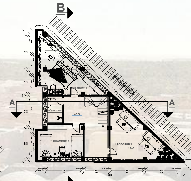
PLAN 1er ETAGE
