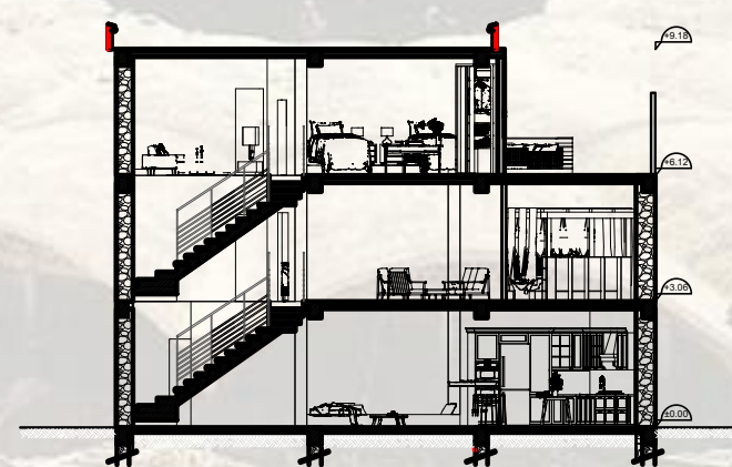
COUPE BB
