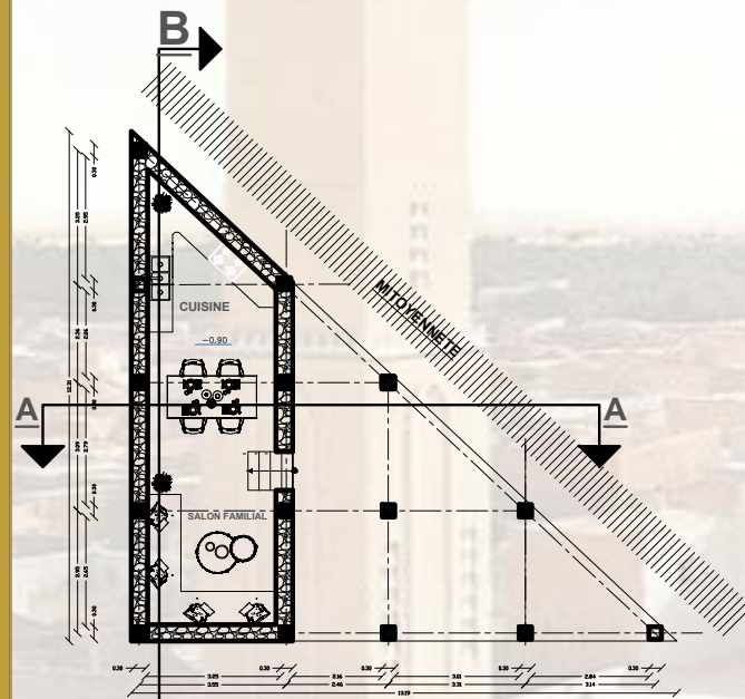
PLAN SOUS-SOL
