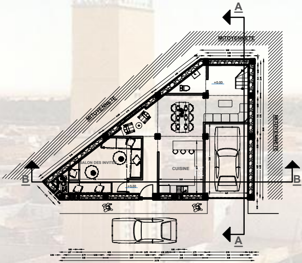
PLAN REZ DE CHAUSSEE
