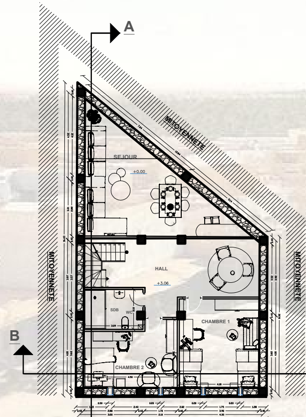
PLAN 1er ETAGE
