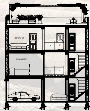
COUPE AA
