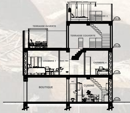
COUPE BB
