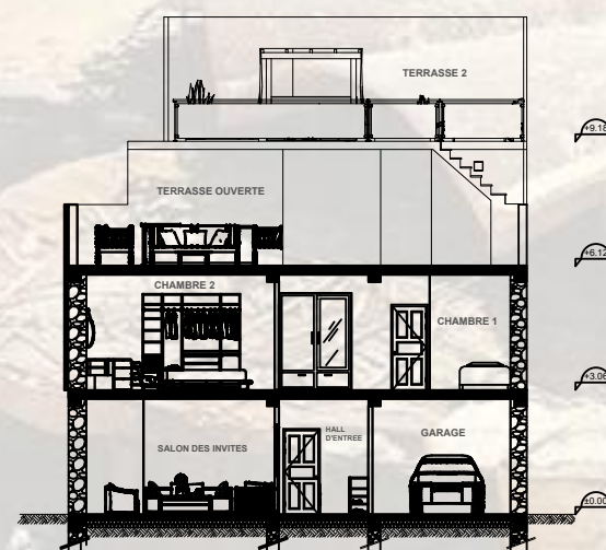
COUPE BB
