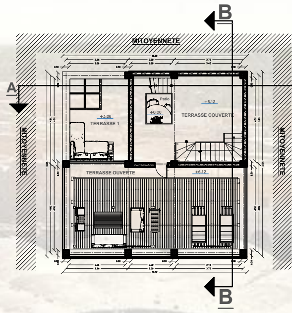
PLAN TERRASSE 1
