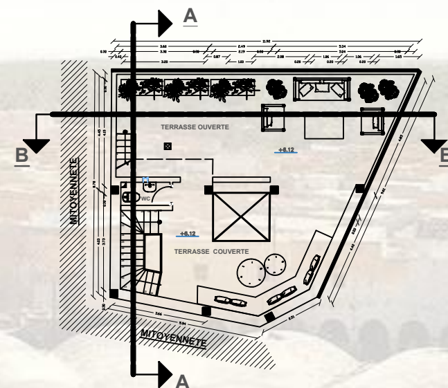
PLAN TERRASSE 1
