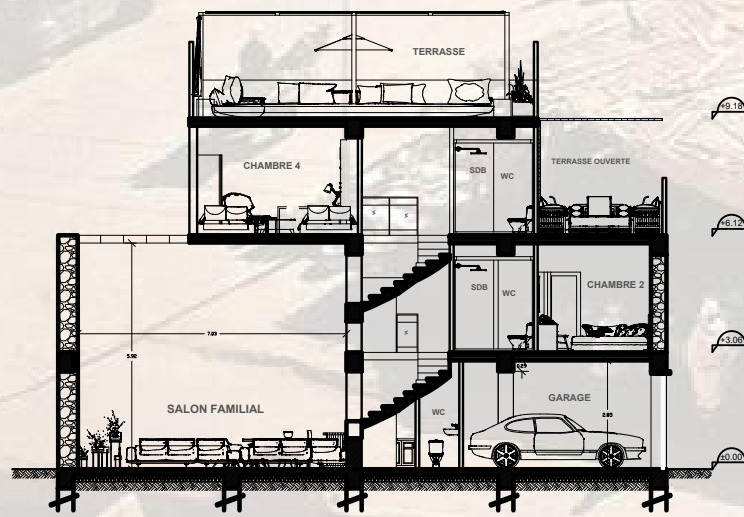
COUPE AA
