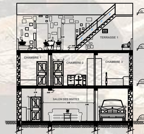
COUPE BB
