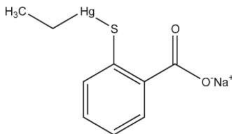
Figure 16: Structure chimique de thimérosal (67)
