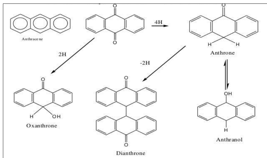
Figure 7 : Dérivés anthracéniques. (123)
