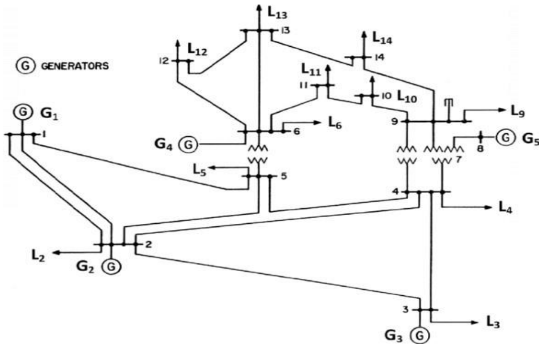
Figure A.1 : Le schéma unifilaire du réseau électrique IEEE 14-Bus.
