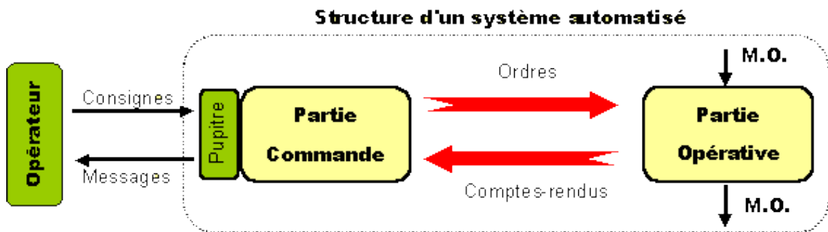
Figure2.1:Structure d'un système automatisé
