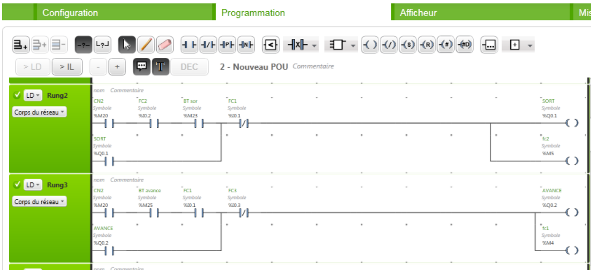
Figure 4.14: Sortie et avance du vérin.
