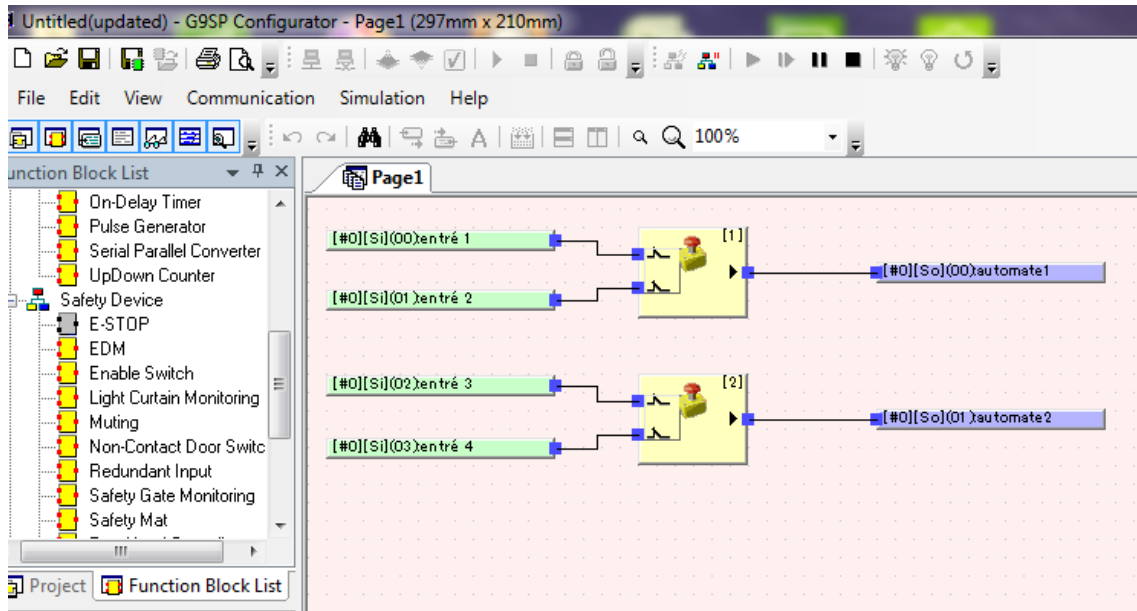
Figure 4.21: Contrôleur de sécurité.
