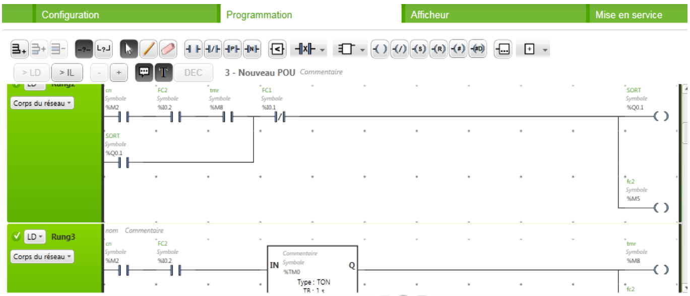
Figure 4.7: Activation du capteur de fin de course 2 et du temporisateur.
