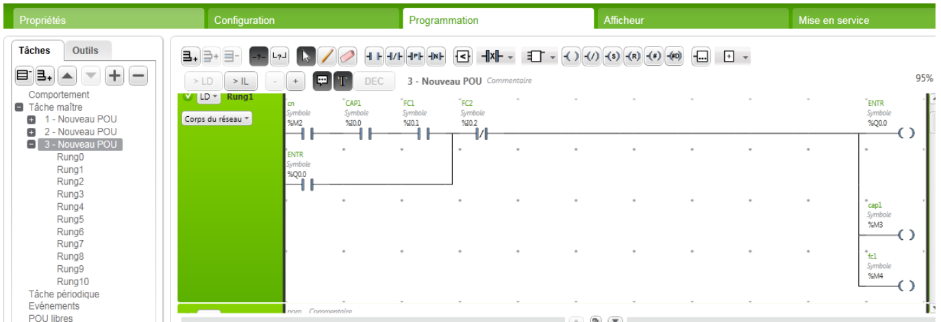
Figure 4.6: Réseau des conditions initiales.
