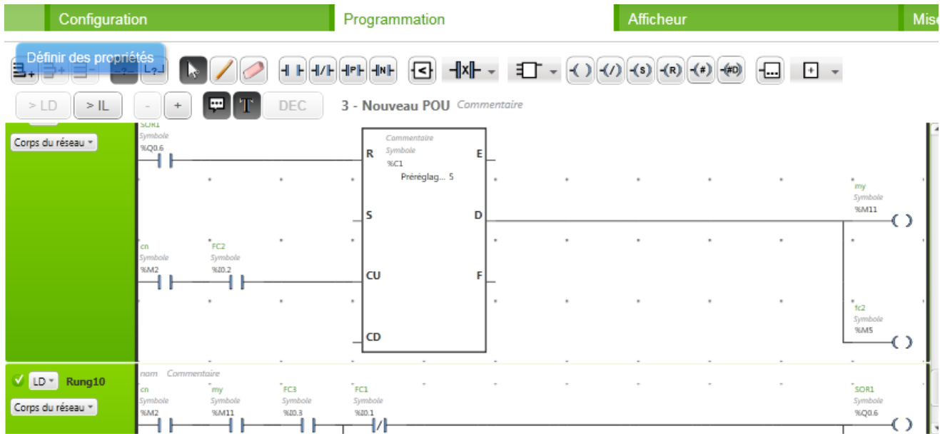
Figure 4.12: Compteur 2 et le retour à l'état initial.
