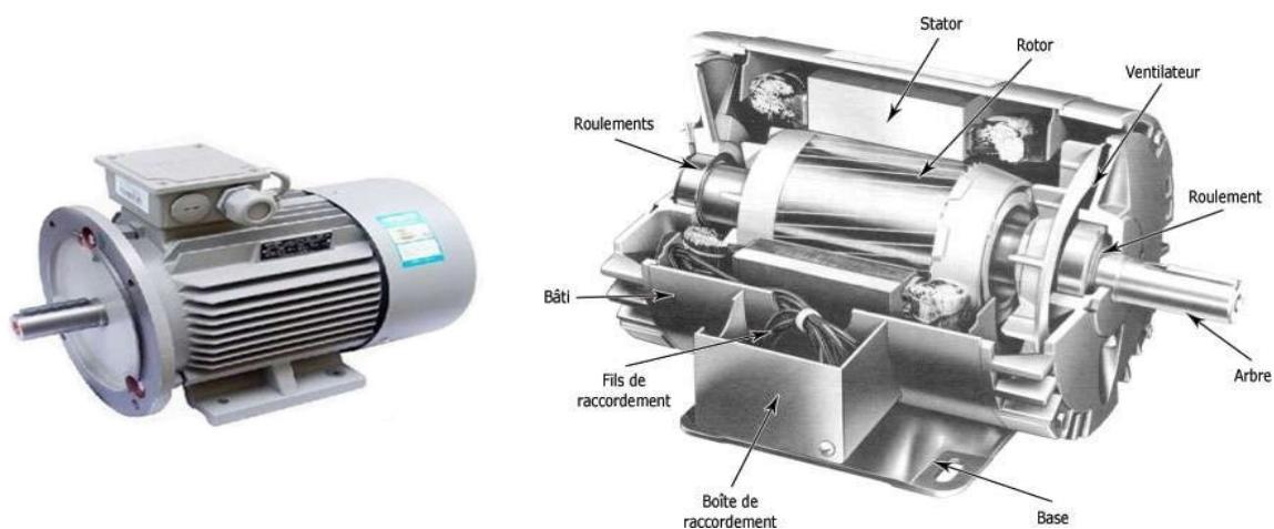
Figure 3.20: Moteur asynchrone triphasé.
