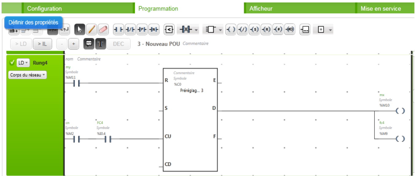
Figure 4.8:Compteur 1.
