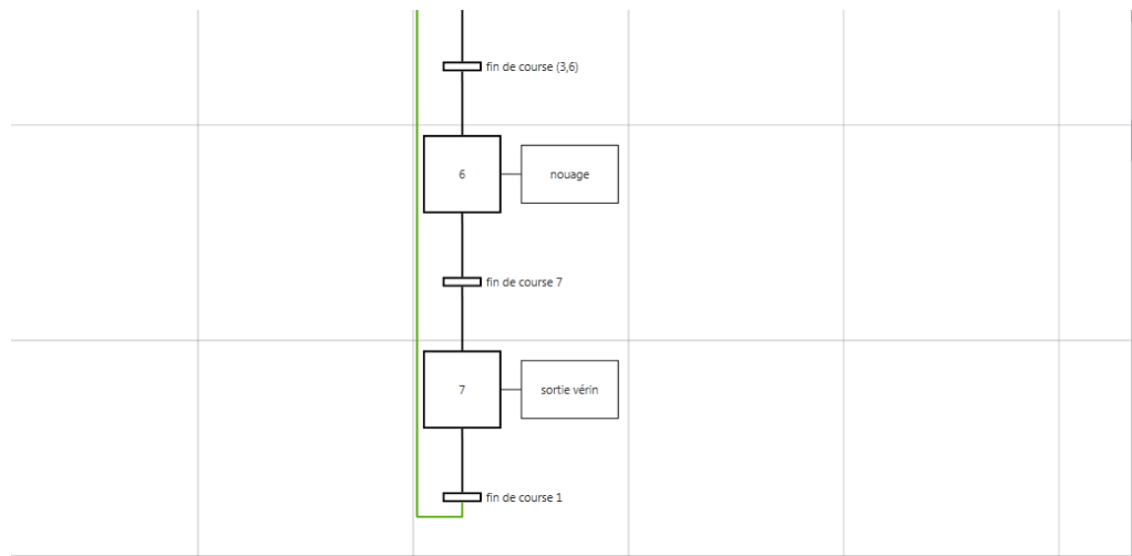
Figure 4.3: Nouage et sortie du vérin a l'état initiale.
