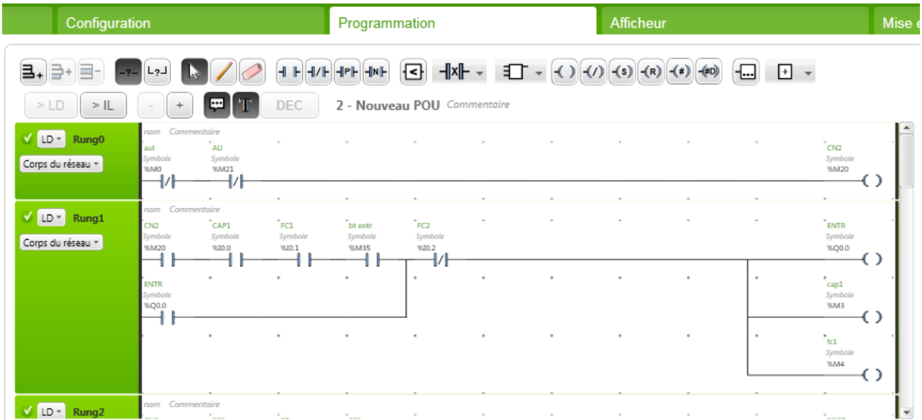
Figure 4.13: Condition de démarrage et sortie du vérin.
