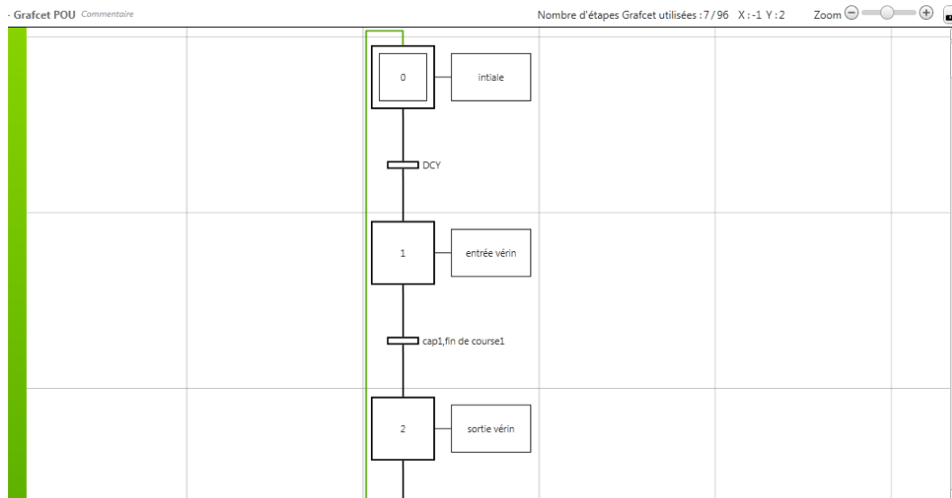
Figure 4.1: entré et sortie du vérin.
