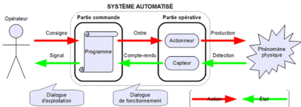
Figure 2.3: Principe de fonctionnement d'un système automatisé.
