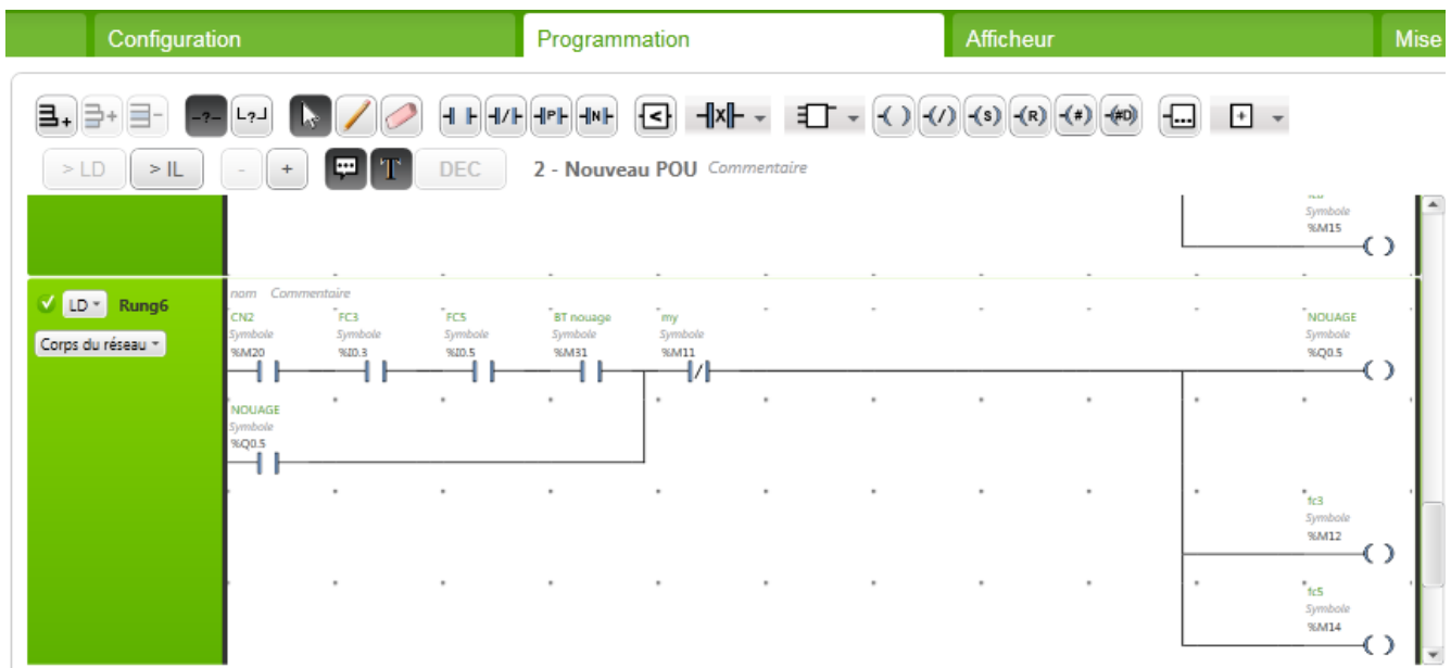
Figure 4.16: Nouage et retour à l'état initial.
