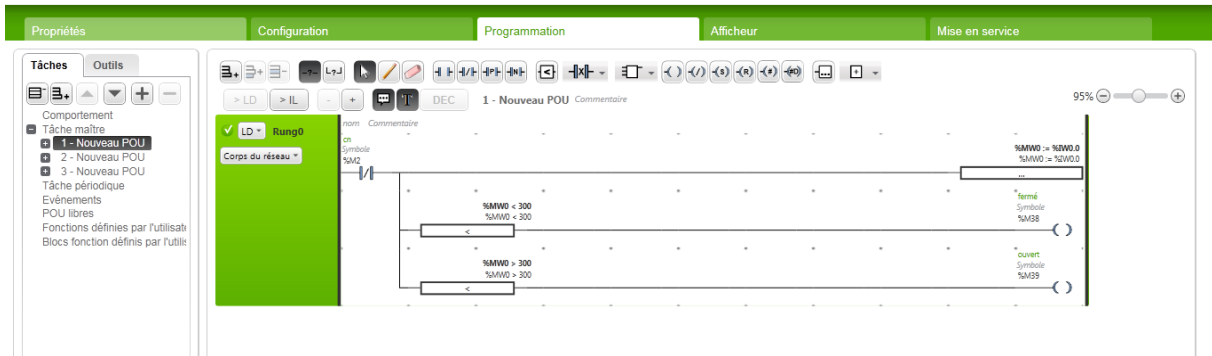
Figure 4.17: Capteur analogique.
