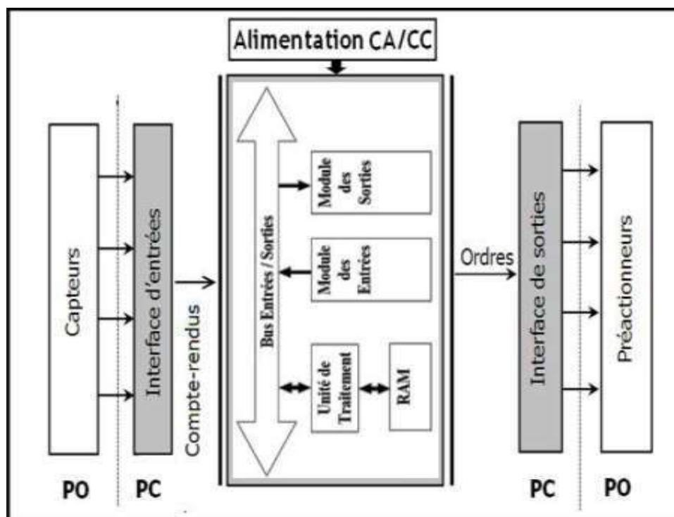
Figure 3.10: Structure interne d'un API.
