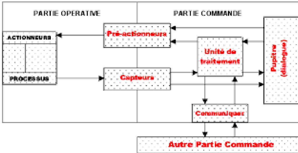
Figure 2.2: Structure interne de la partie commande et la partie opérative.
