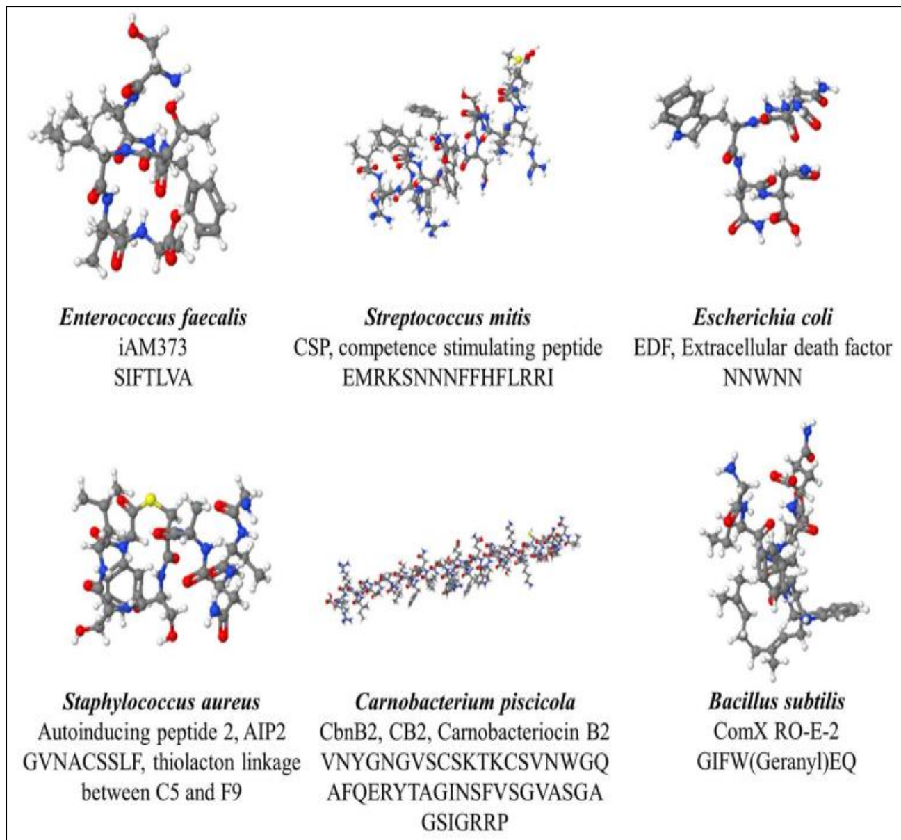
Figure 17 : Divers peptides de détection du quorum, illustrant la diversité structurelle observée parmi les peptides de détection du quorum (Verbeke et al. , 2017).
