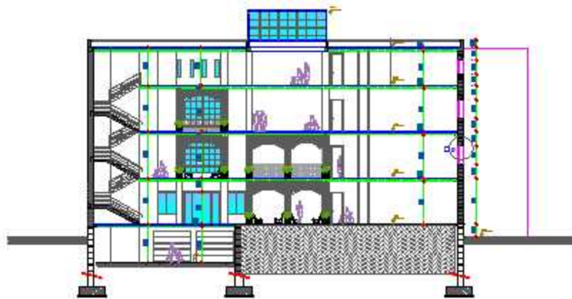
COUPE B-B
