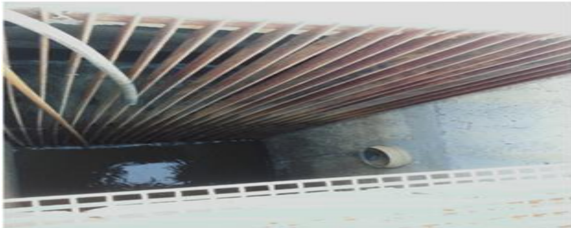
Figure 2.4 : Dégrilleur Grossier.
