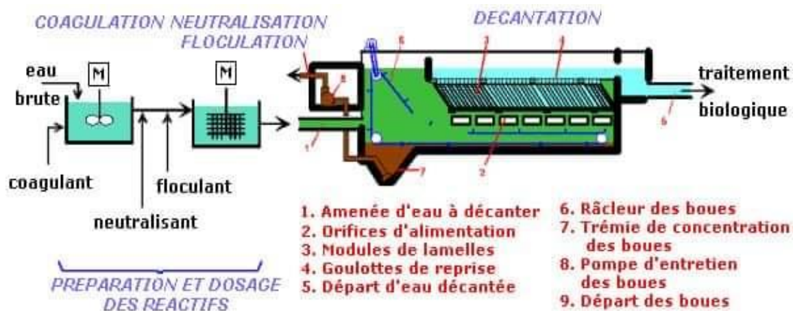
Figure 1.4 : Traitement physico-chimique des eaux usées.
