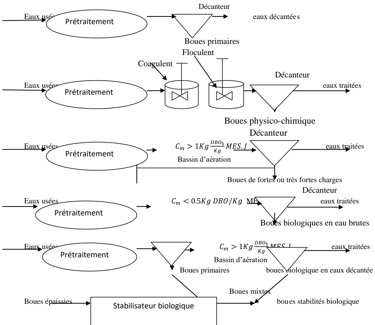
Figure 1.6 : Différent type de boues selon le traitement [27].
