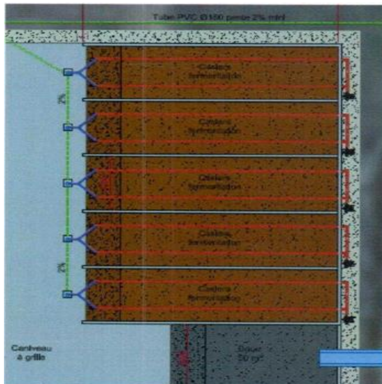
Figure 3.4 : casiers de fermentation.
