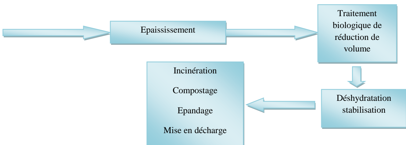
Figure 1.8 : Différentes étapes du traitement des boues [35].
