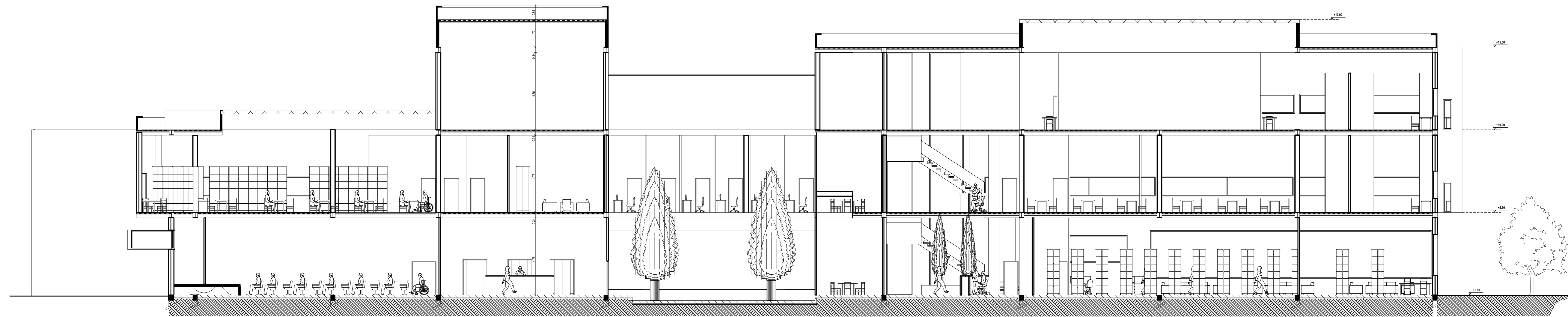
COUPE A-A
