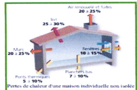
Figure 25 : schéma des déperditions thermiques dans une maison. Source : http://www.seol.fr/isolation-2-51.html consulté le 30-06-2017
