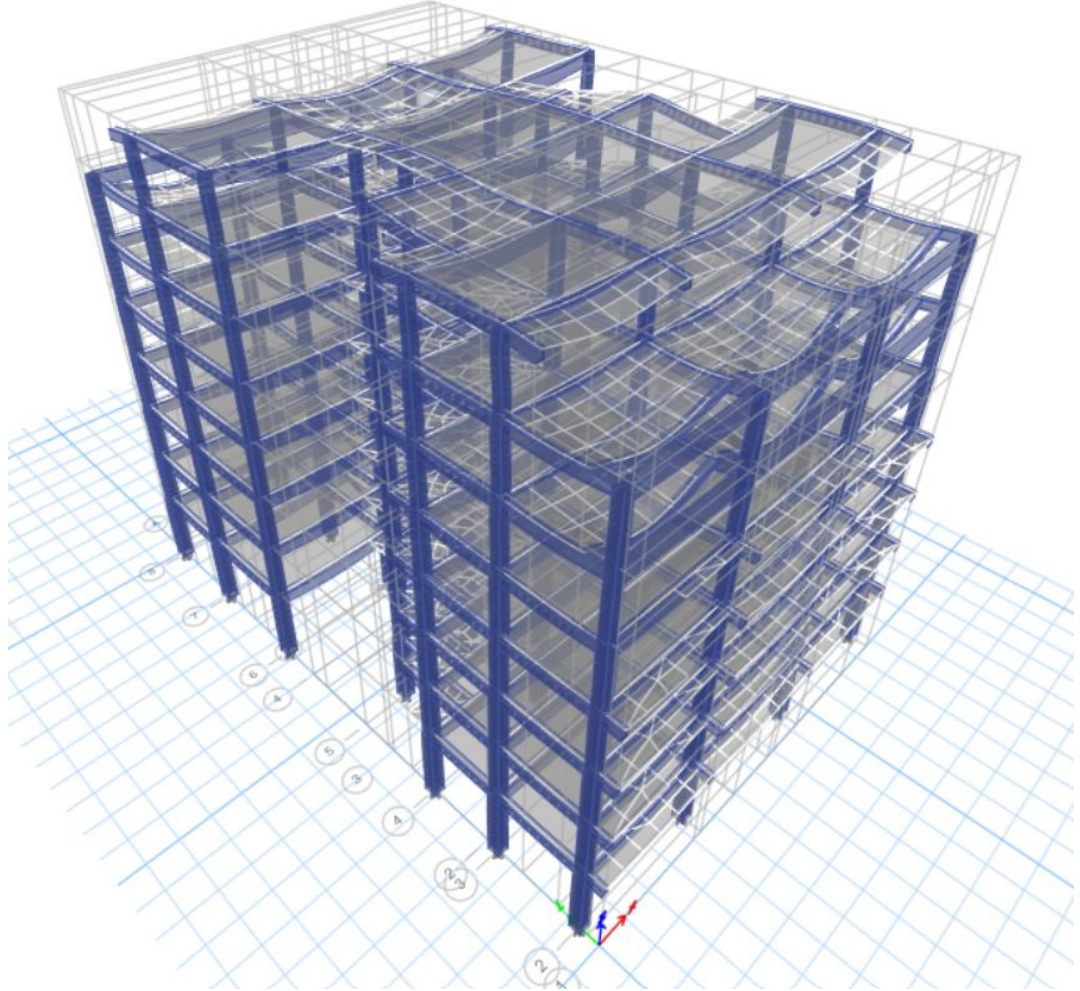
Figure IV. 8: Déformation verticale.
