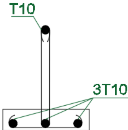
Figure III. 13: Ferrailage de poutrelle sur travée.
