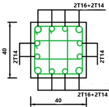
Figure V. 4: Schéma de ferrailage de poteau 40x40.
