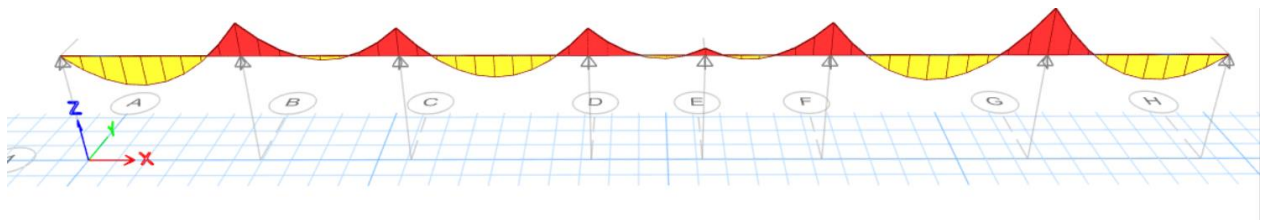
Figure III. 10: Diagrammes des Moments à ELS.
