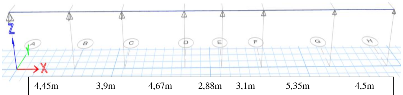
Figure III. 7: Schéma de la Poutrelle à 7 travées.
