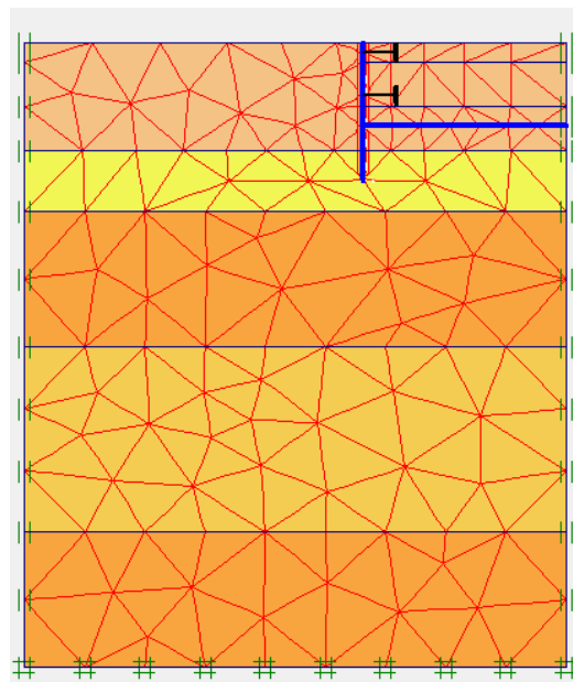
Figure IV.4. Représentation du maillage obtenu à l'aide du logiciel PLAXIS
