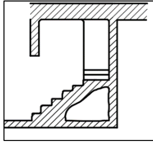
Figure 156: coupe de l'escalier. Source: fait par l'auteur
