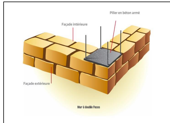
Figure 214 : la structure mixte béton et pierre. Source : OPVM
