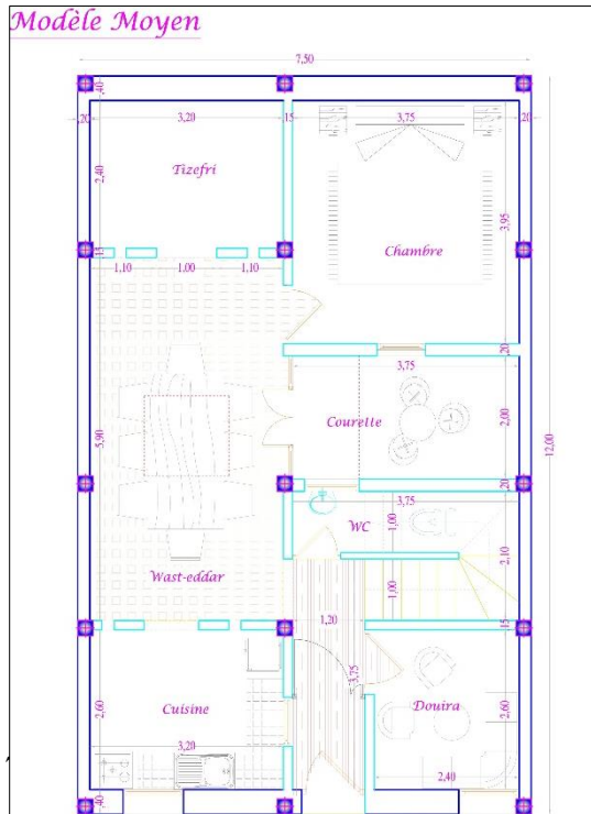
Figure 128: plan RDC de la maison model moyenne, ksar Tafilalet. Source : fondation amidoul.
