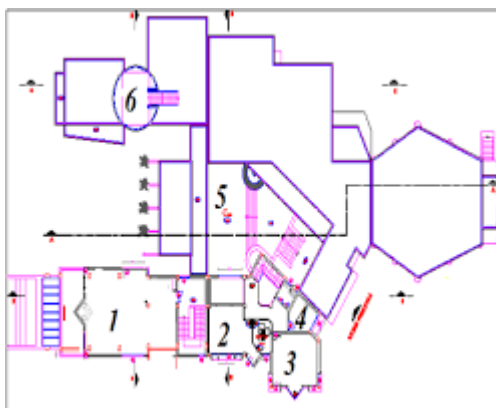
Figure 51: PLAN D' ETAGE DU CLS
