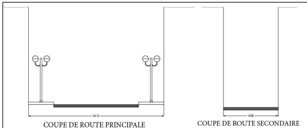
Figure 124: les coupes des voies principales et secondaires. Source : fait par l'auteur
