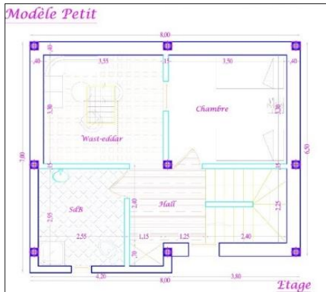
Figure 137: plan d'étage de la maison type petite. Source : fondation amidoule
