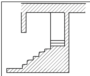
Figure 172: escaliers sur blocage de pierres. source: fait par l'auteur
