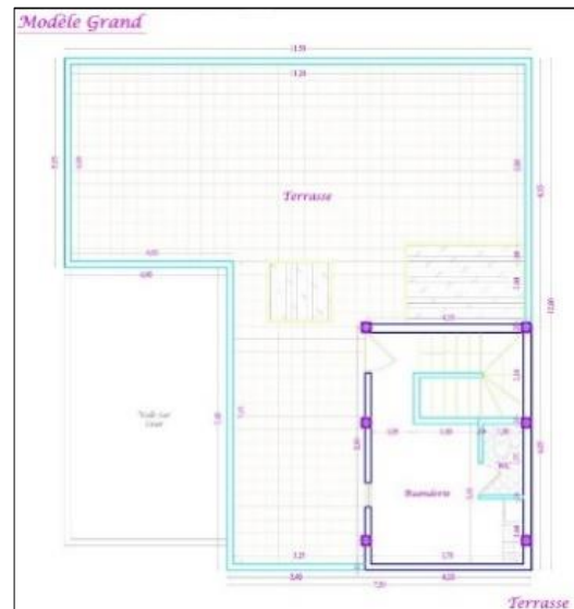
Figure 133: plan de Terrasse du type grand. Source: fondation amidoul
