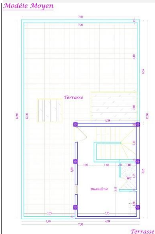
Figure 130: plan de l'étage de la maison du type moyen, ksar tafilalet. source : fondation amidoul
