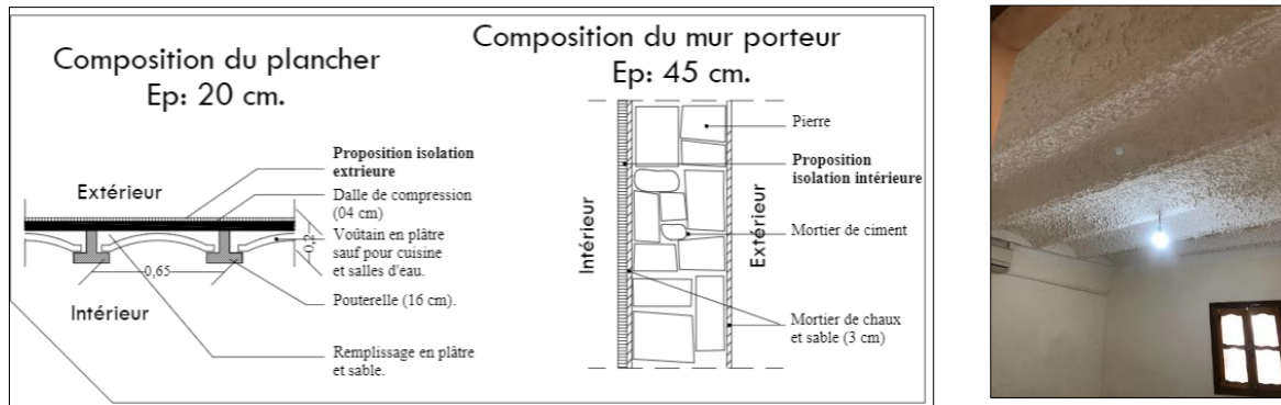
Figure 141: schéma et photo explicatif de la composition du plancher et du mur porteur
