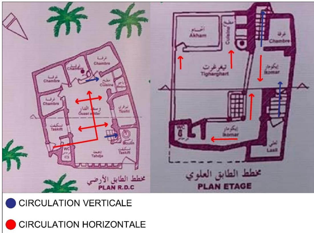
Figure 182: schéma qui montre les types de circulation dans la maison de la palmeraie. Source : plan de l'OPVM traité par l'auteur.
