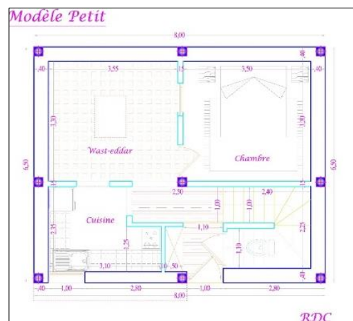
Figure 135: plan de RDC type petit. source: fondation amidoul
