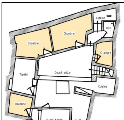
Figure 152: la chambre sur le plan. Source : plan modifié par l'auteur
