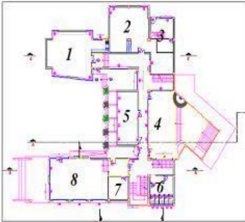
Figure 49: plan SOUS SOL DU CLS
