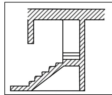
Figure 170: escaliers sur poutres de palmier. Source : fait par l'auteur
