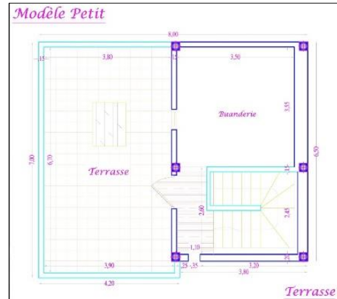
Figure 138: plan de terrasse de la maison type petite. Source : fondation amidoule
