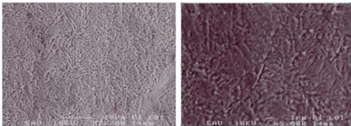
Figure 3.7 troisième microstructure du traitement thermique
