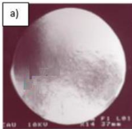
Figure 3.12 Surface du point de rupture d'échantillon de la 3ème séquence de traitement thermique [24]
