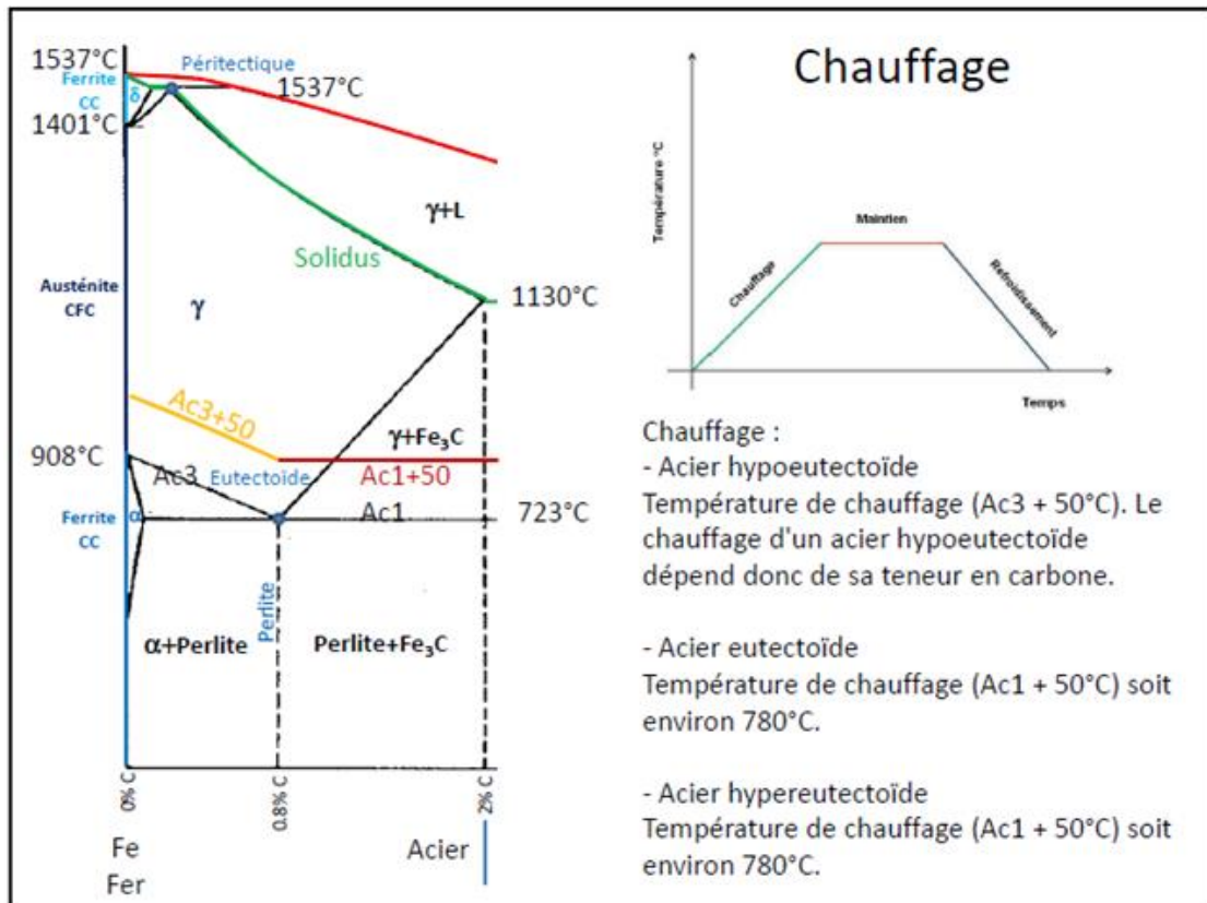
Figure 2.4 illustration principes et diagramme du recuit.[16]
