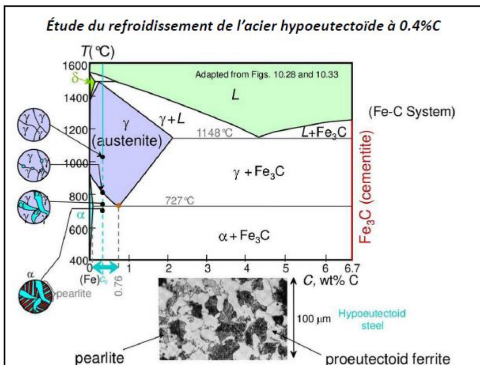
Figure 1.3 Diagramme d'équilibre Fer-Carbone.[6]
