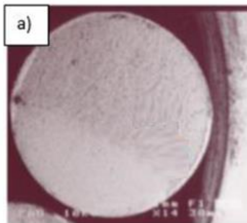
Figure 3.10 Surface du point de rupture d'échantillon de la première séquence de traitement thermique [24]
