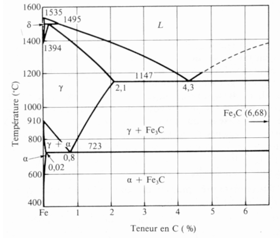
Figure 1.3 Diagramme d'équilibre Fer-Carbone.[6]
