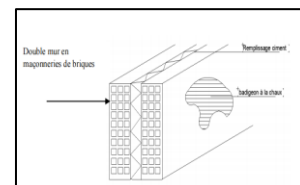
Figure 67 : Les composants des murs de l'hôtel des Ziban
