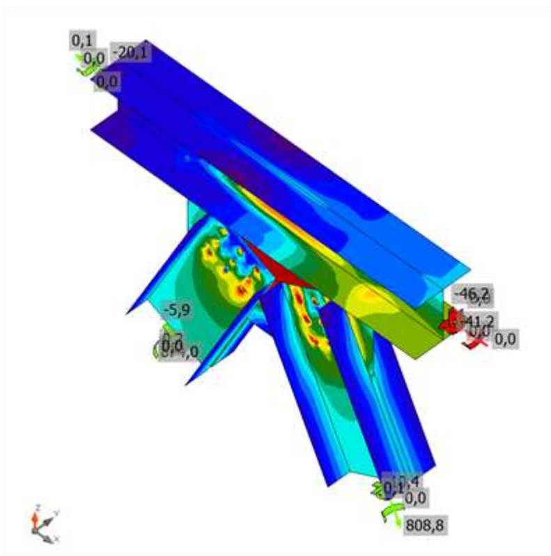
Contrainte équivalente, G+Q-1.5EX
