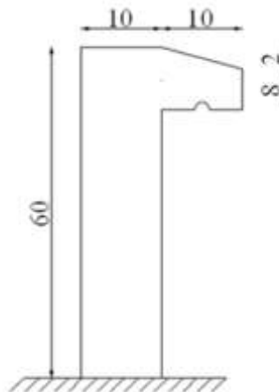
Figure IV. 5: Dimensions de l'acrotère.
