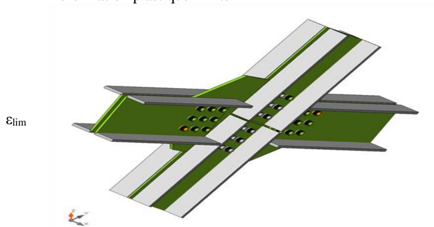
Vérification globale, G+Q-1.5EY
