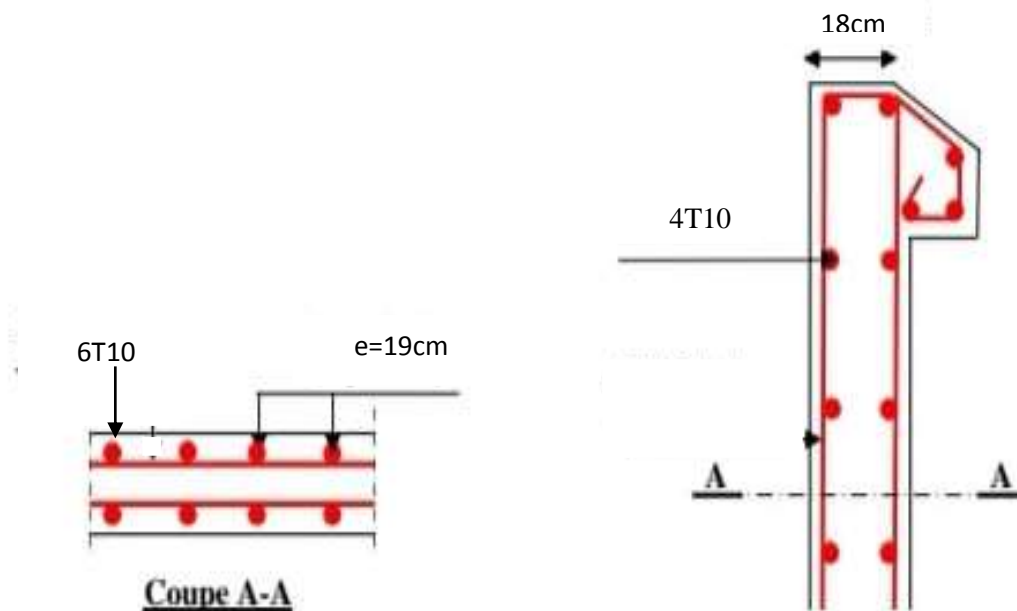
Figure IV. 7: Schéma de ferrailage de l'acrotère.
