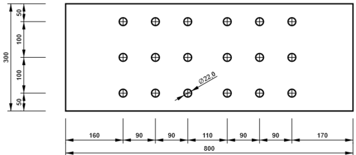
Figure VII. 17: les dispositions des boutons sur les Platines P20.
