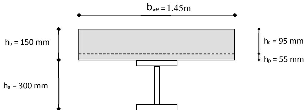
Figure II. 11: Largeur participante de la dalle.
