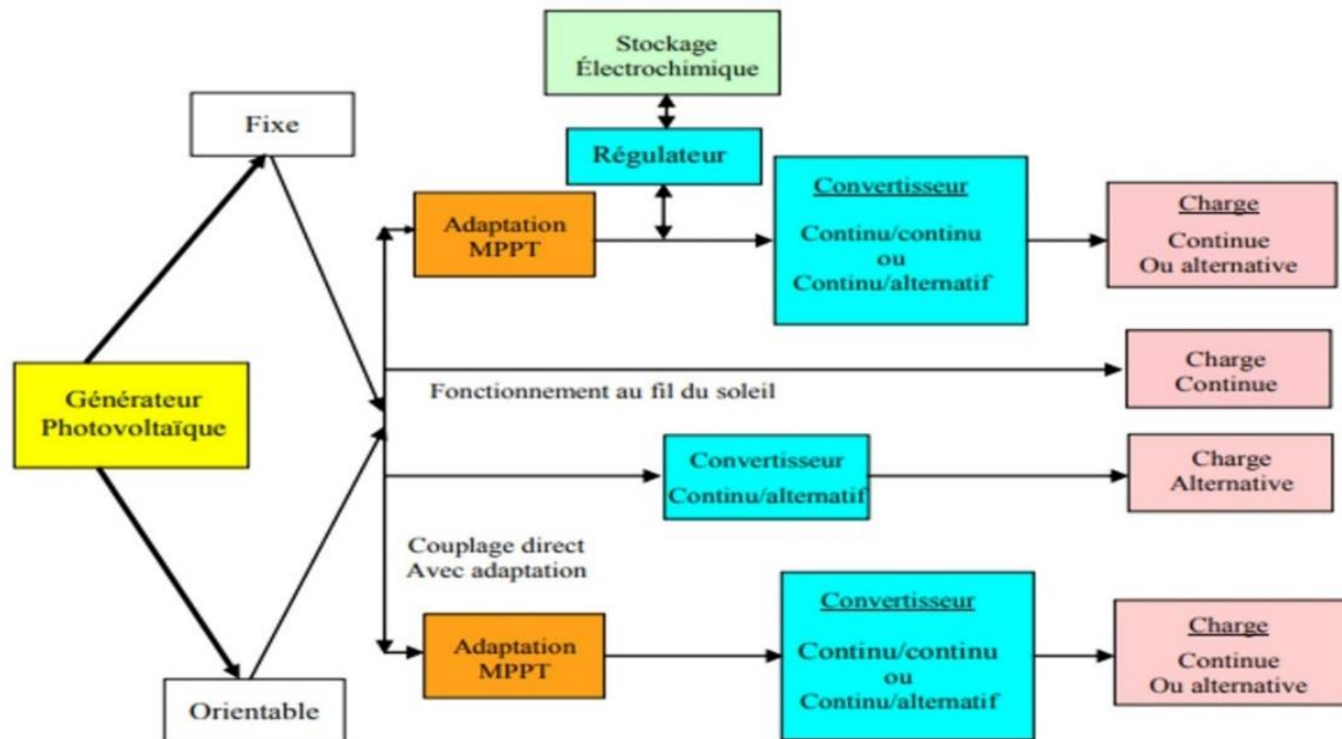
Figure I-7 : système photovoltaïque autonome.
