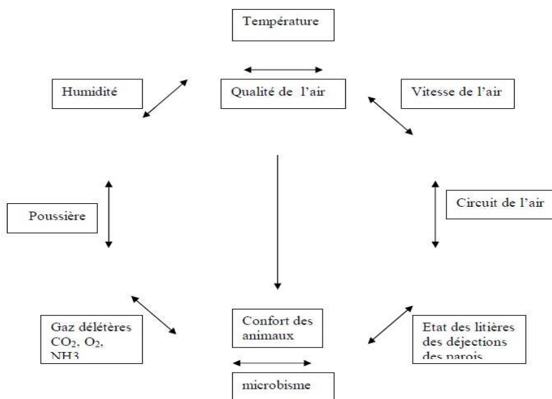
Figure 2: Paramètres définissant les conditions d'ambiance (ITAVI, 2001)
