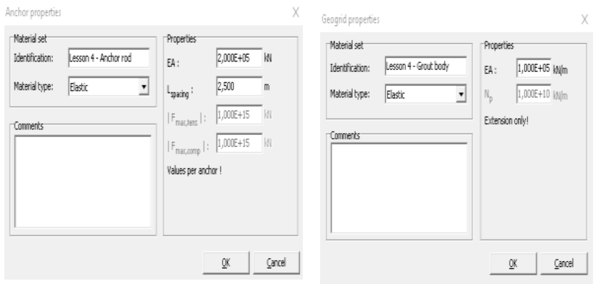
a) paramètre de tirant d'ancrage b) paramètres scellement.
