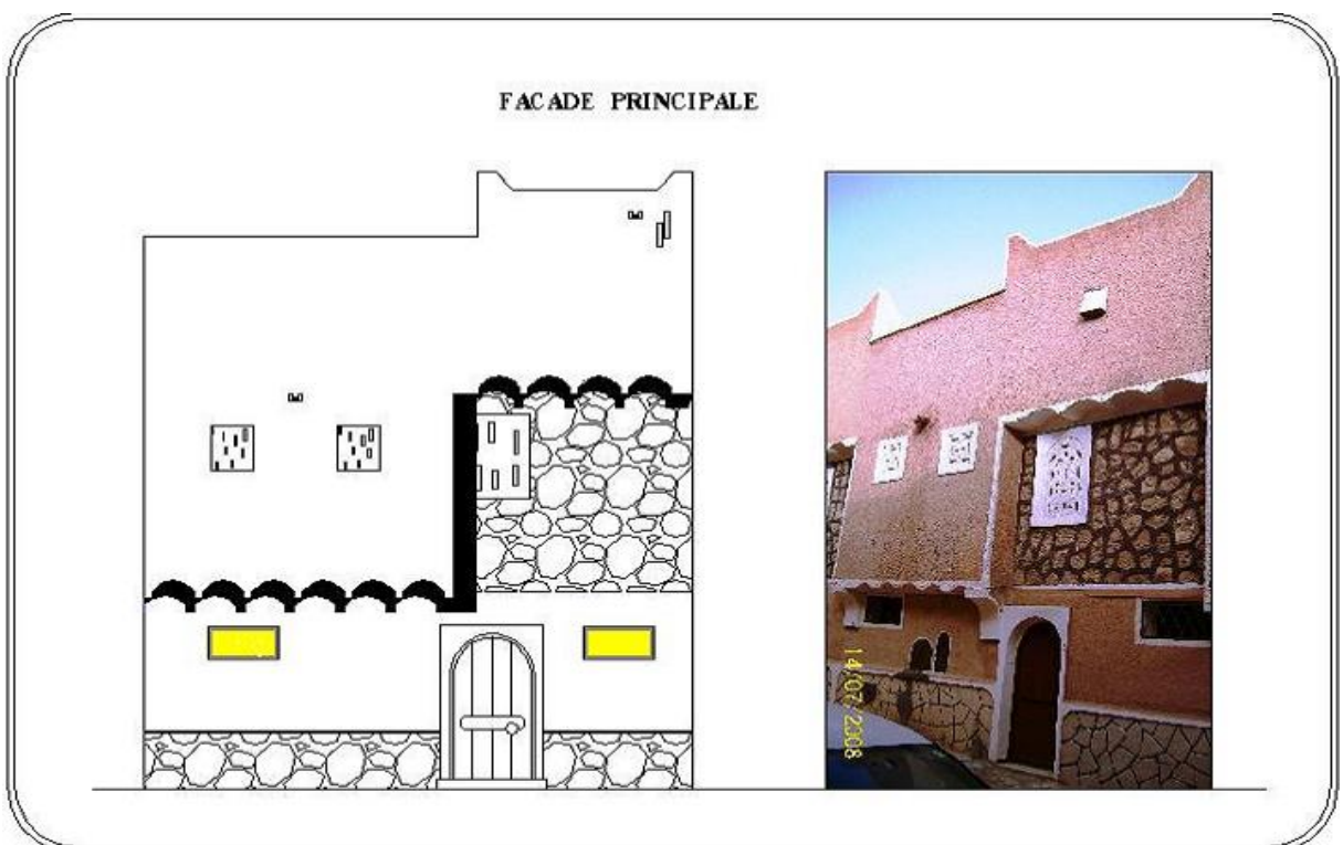
Figure II.20 : Façade principale et plan de la terrasse. [44]
