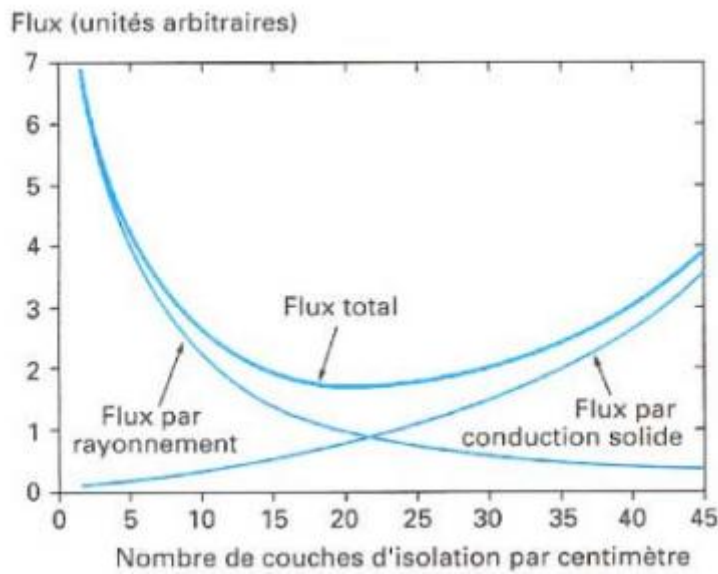
Figure 3.9 : Flux thermique transmis dans un superisolant en fonction du nombre de couches par unité d'épaisseur.
