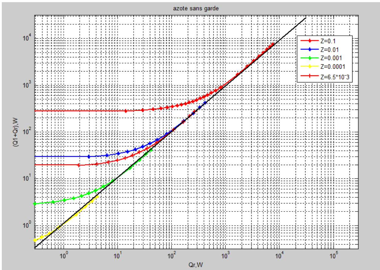
Figure 5.1 : pertes dans les conteneurs azote sans garde.
