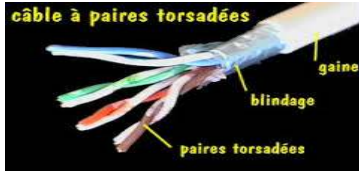
Figure I.5: Câble à paires torsadées non blindées et blindées
