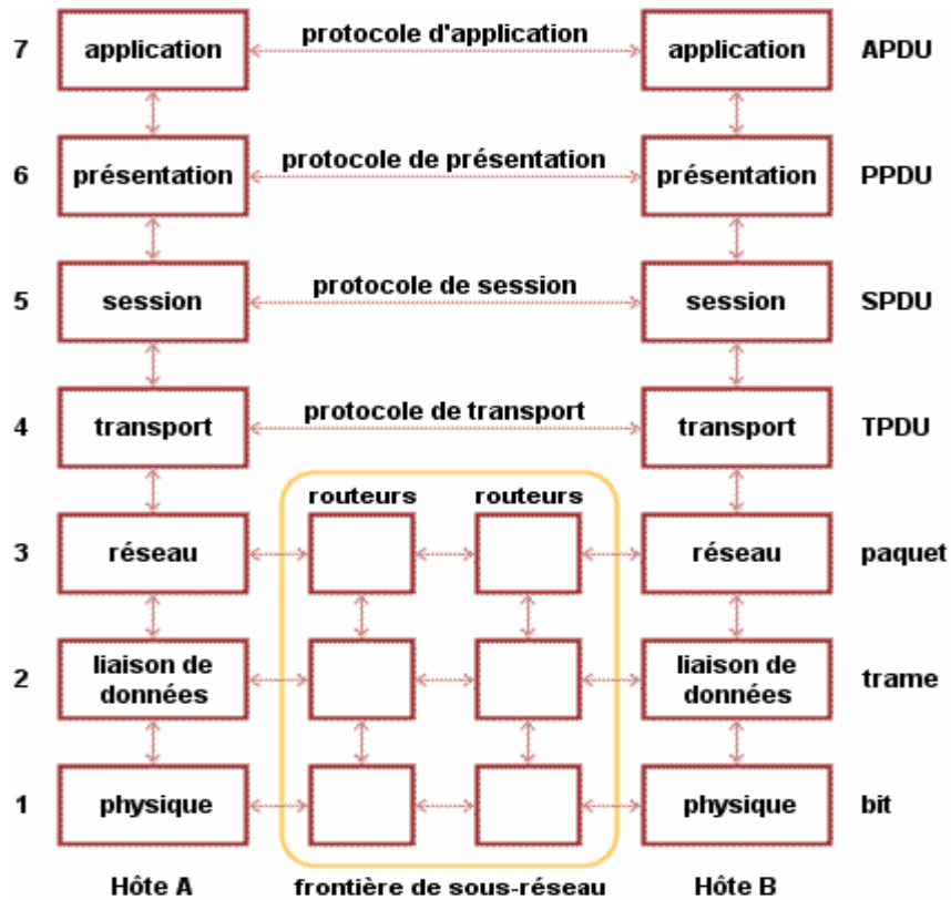
Figure I.8 : Le modèle OSI.
