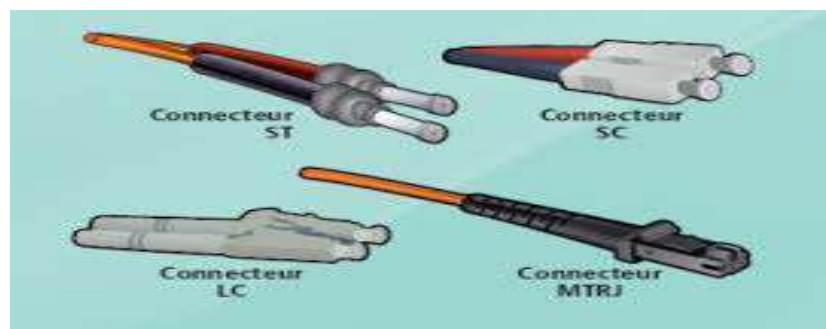
Figure I.7: Fibreoptique.
