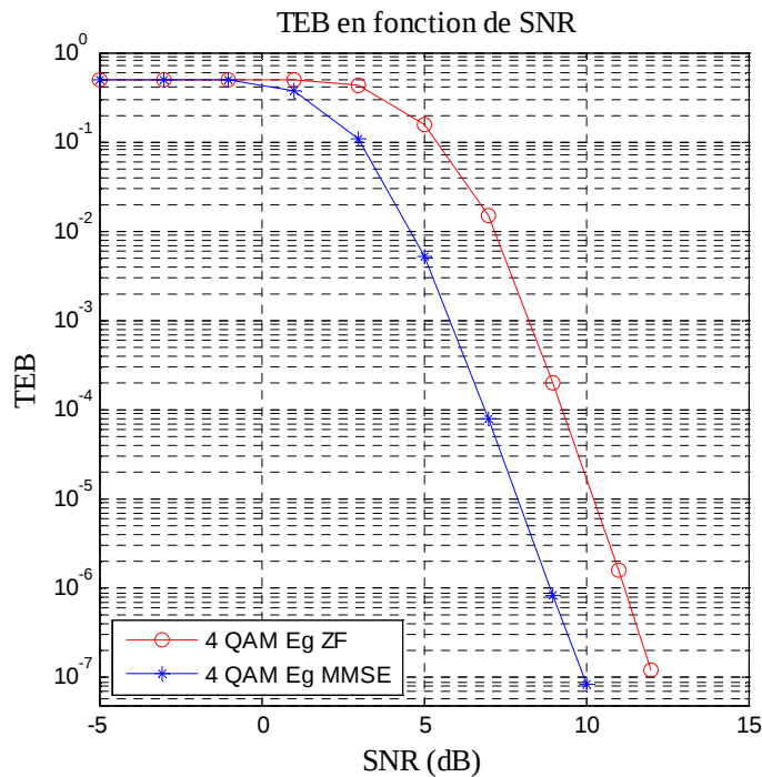
Figure 4.18 : Comparaison entre les égalisateurs ZF et MMSE (canal réel).
