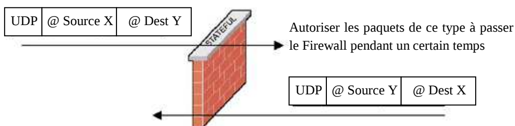
Figure 4. Filtrage de paquet avec état (UDP)
