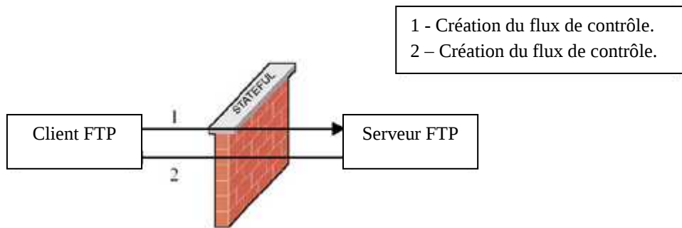
Figure 5. Filtrage de paquet avec état (FTP)
