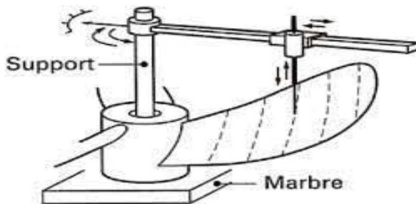
Fig.1.2: Principe du dispositif de contrôle des pales [7]
