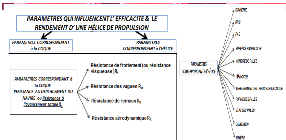
Fig.3.9: Paramètres liés au rendement.
