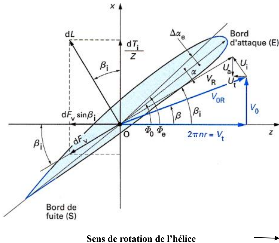
Fig.2.11: Différentes grandeurs intervenant dans le fonctionnement. [7]
