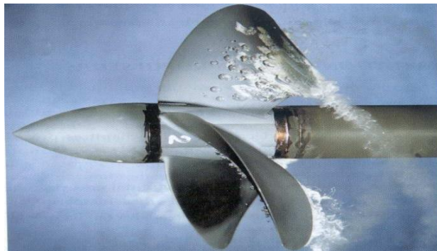
Fig.3.4: Cavitation à bulles suivie d'un nuage de cavitation. [7]
