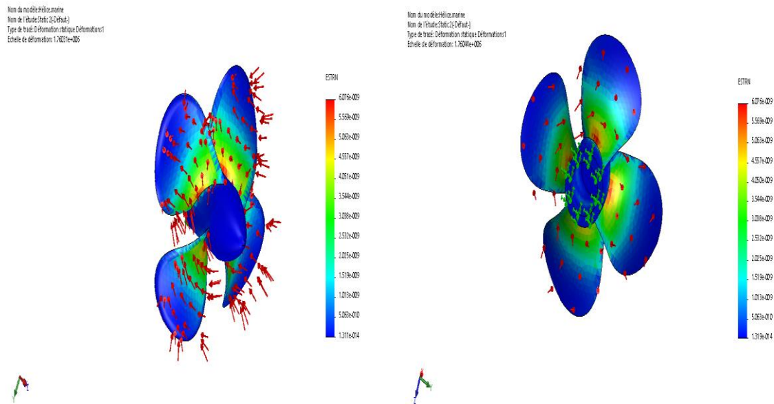
Fig.4.9: Déformation sur les faces des pales.
