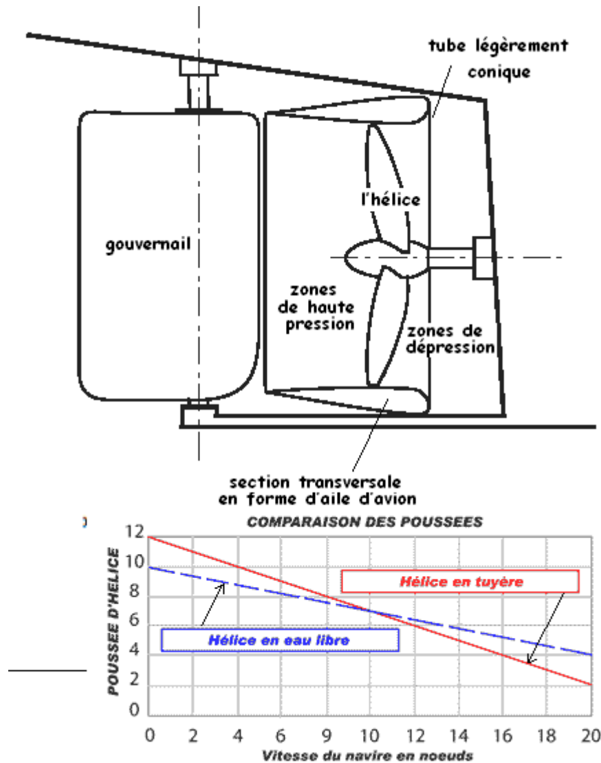
Fig. 3.11: Influence de la tuyère sur le rendement.
