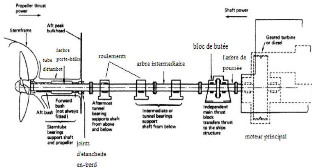
Fig.3.1: Système de transmission.
