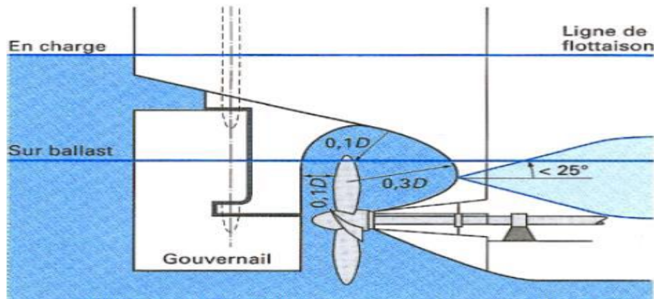
Fig. 3.10: Espace optimal entre l'hélice et la coque.
