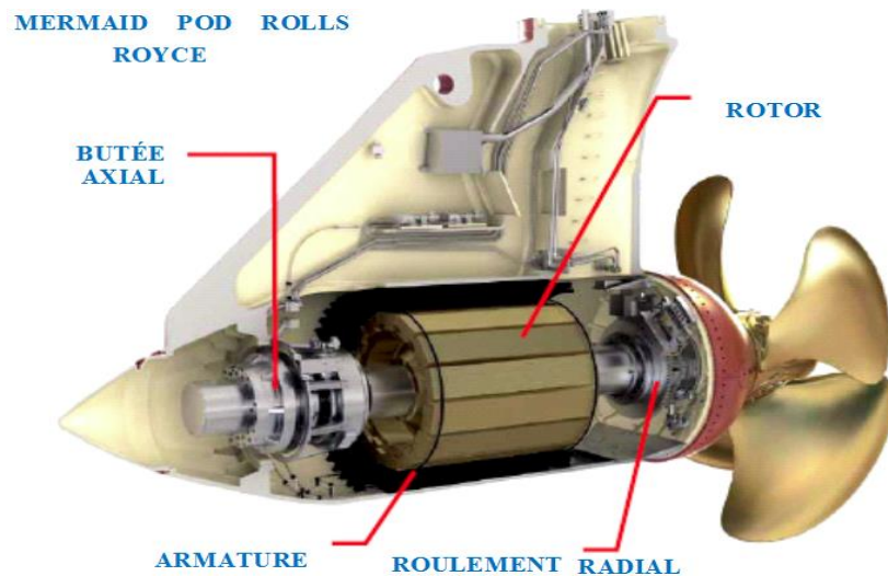
Fig.1.9 : Hélice POD. [6]
