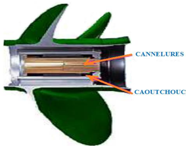
Fig.1.10: Détails du moyeu intérieur [5]
