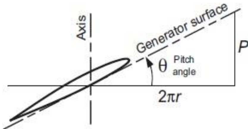
Fig.2.6: Pas géométrique d'hélice. [7]
