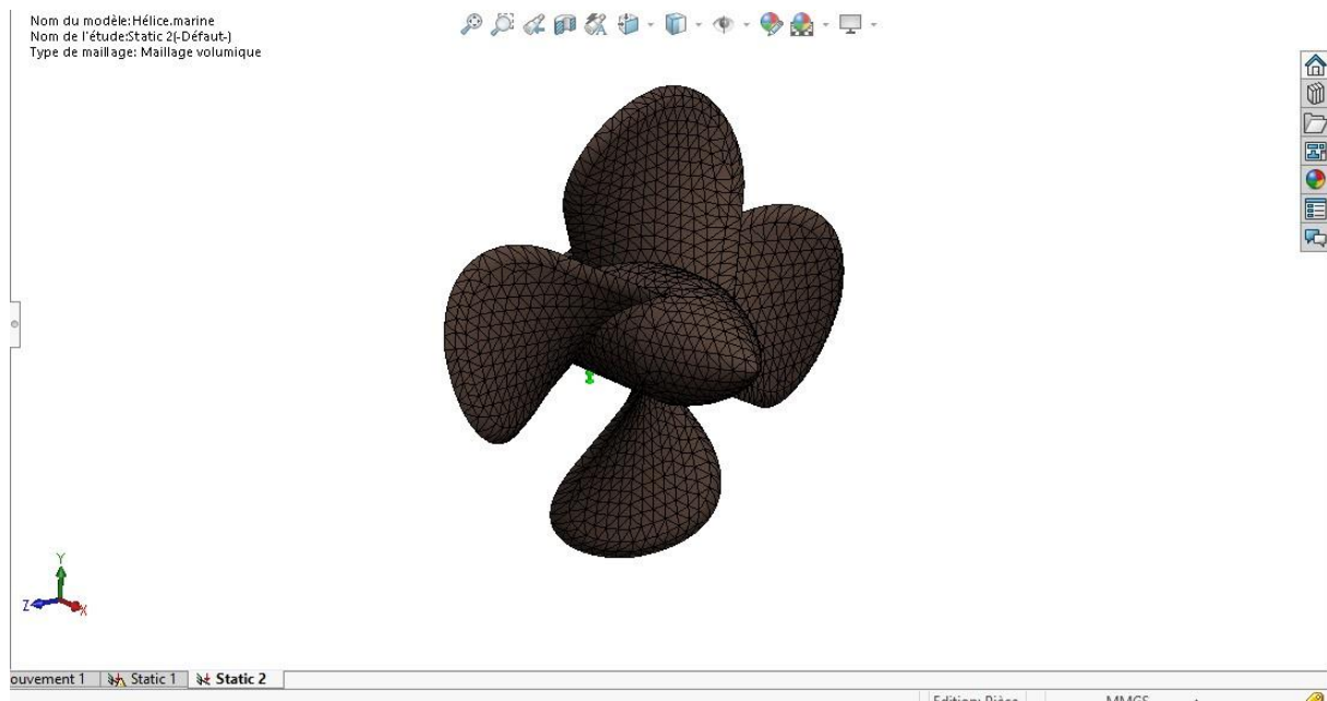
Fig.4.7: Maillage volumique de l'hélice
