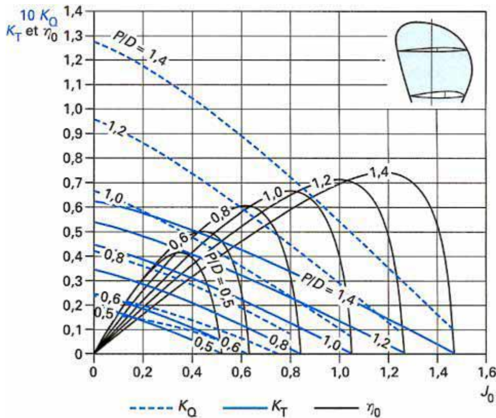
Fig.2.13: Courbes de performance hydrodynamique des hélices B4-70, avec en médaillon le contour développé [7]
