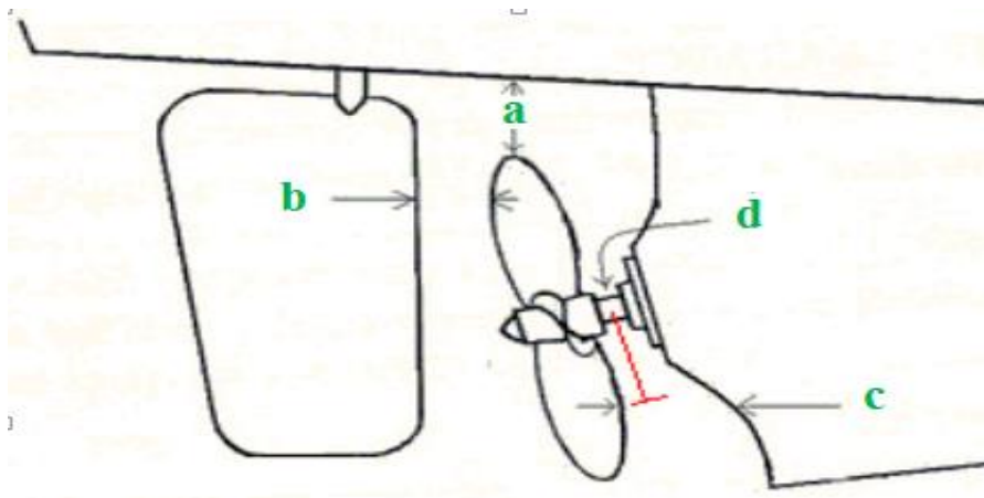
Fig.3.13: Espacement normalisé.
