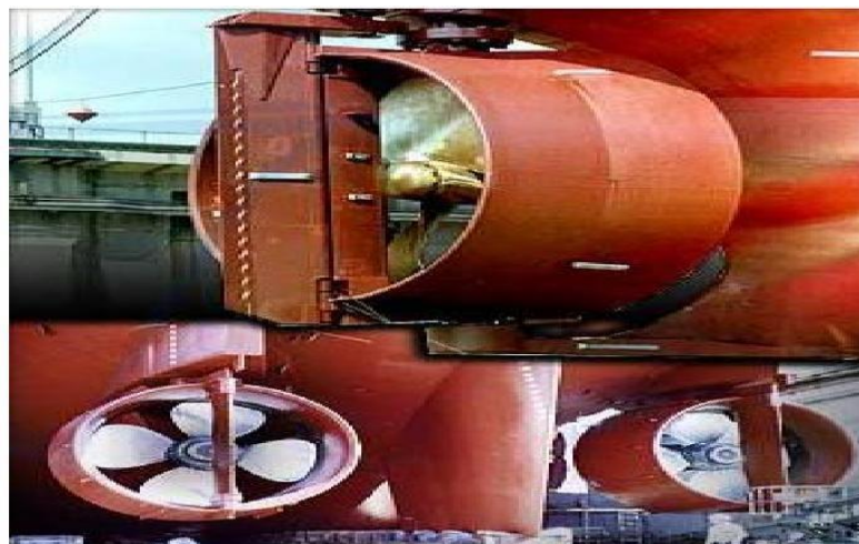
Fig.1.5: Hélice sous tuyères. [13]
