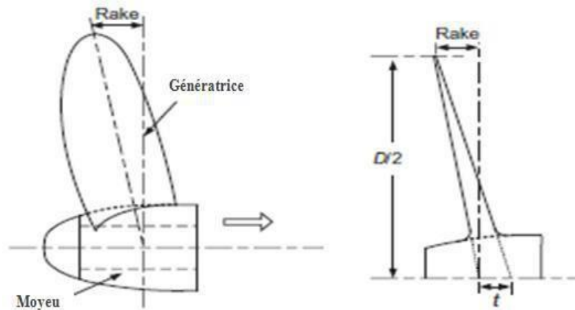
Fig.2.7: Rake positif d'une pale. [6]
