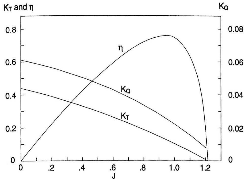
Fig.2.12: Exemple de courbes de performance hydrodynamique d'une hélice. [7]
