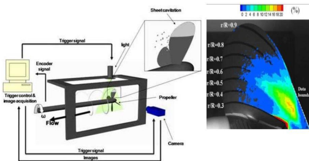
Fig. 4.11: Dispositif expérimental de la cavitation. [1]
