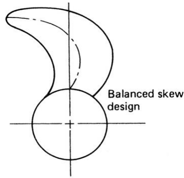
Fig.2.9: Dévers balancé d'une hélice. [7]
