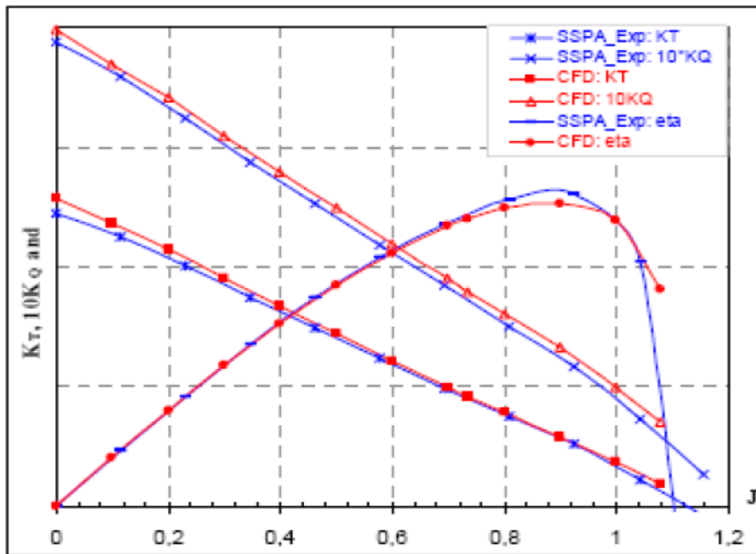
Fig.4.13: Caractéristiques hydrodynamiques. [3]
