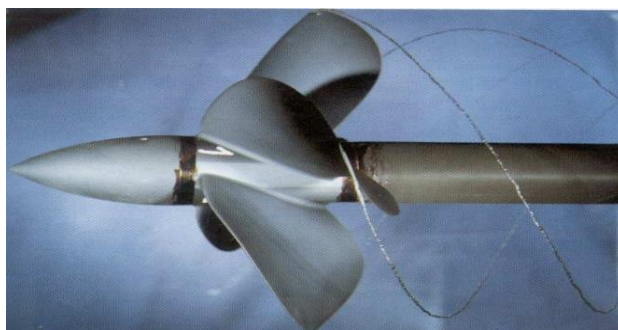
Fig.3.6 : Cavitation de tourbillon marginal. [7]
