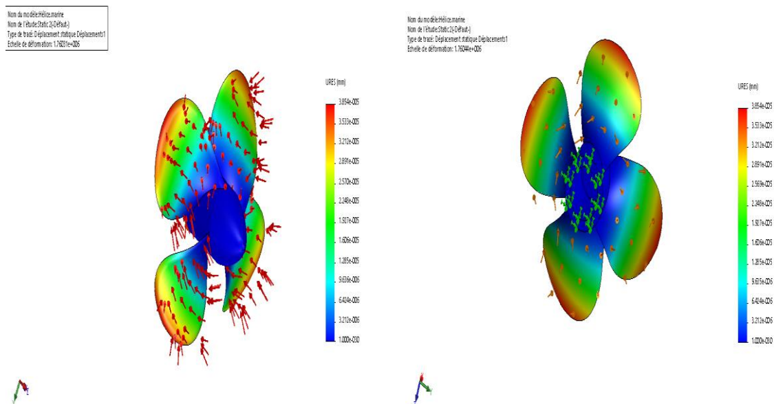
Fig.4.10: Déplacement sur les faces des pales
