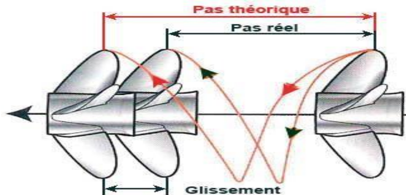
Fig.2.5: Glissement et pas.[8]
