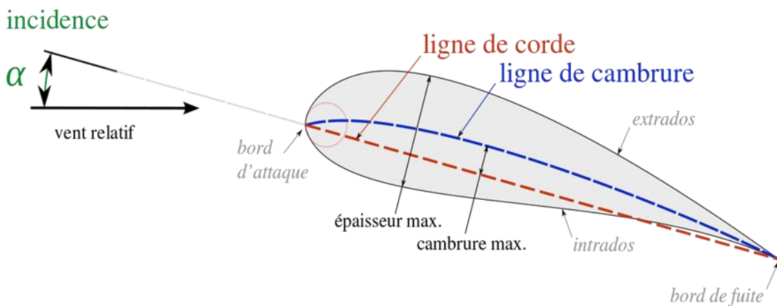
Fig.2.2: Détails de profil d'une pale [4]
