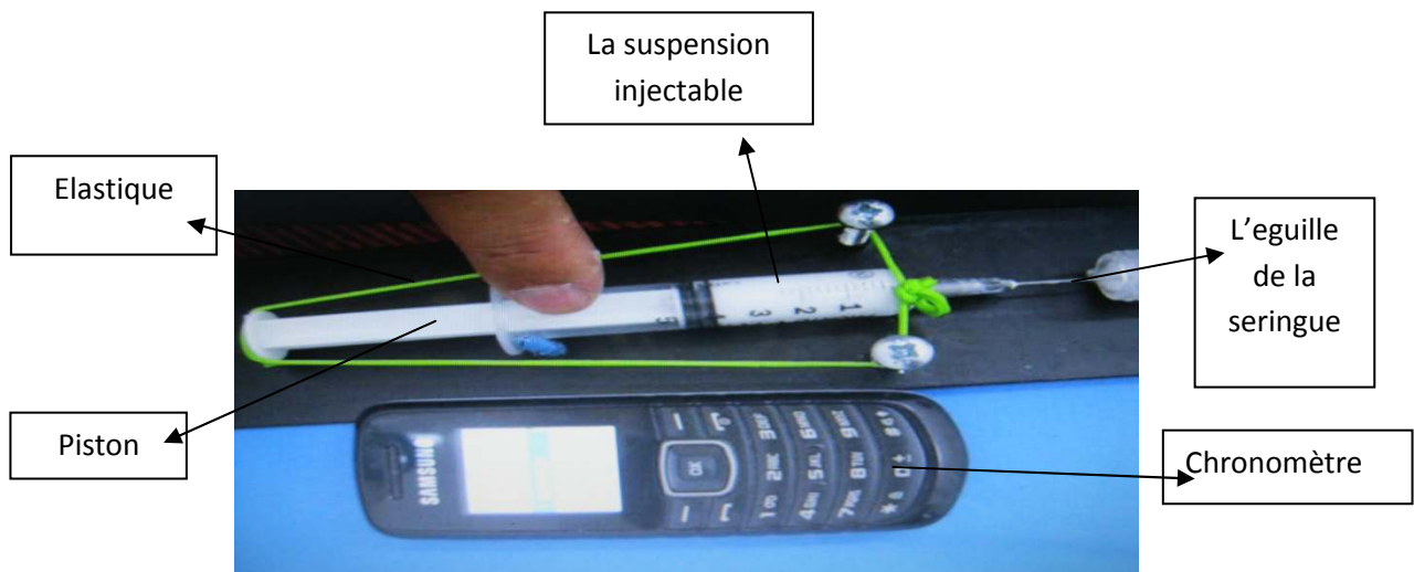
Figure (III.5) : Le montage de l'essai de l'écoulement
