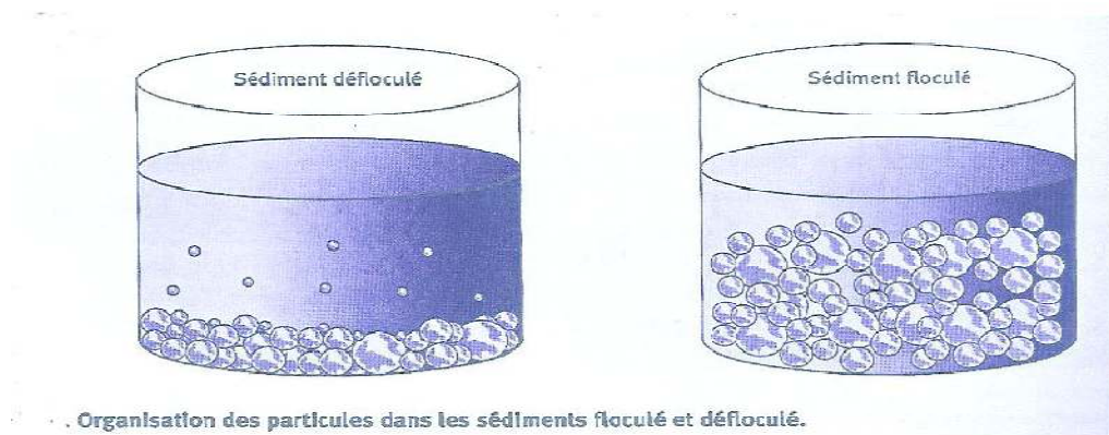
(Figure I.1) : Représentation de la sédimentation des suspensions floculées et défloculée
