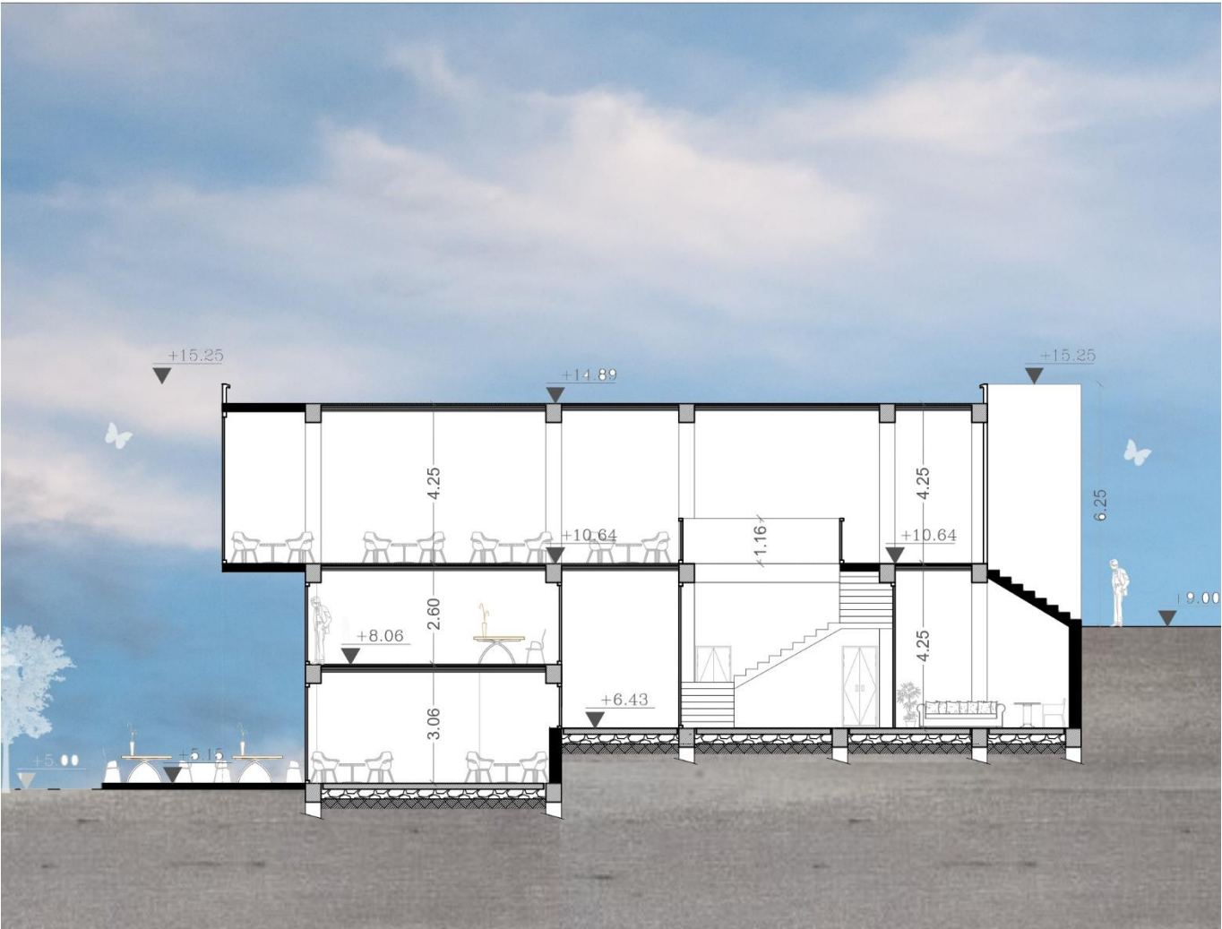
LA COUPE C-C
