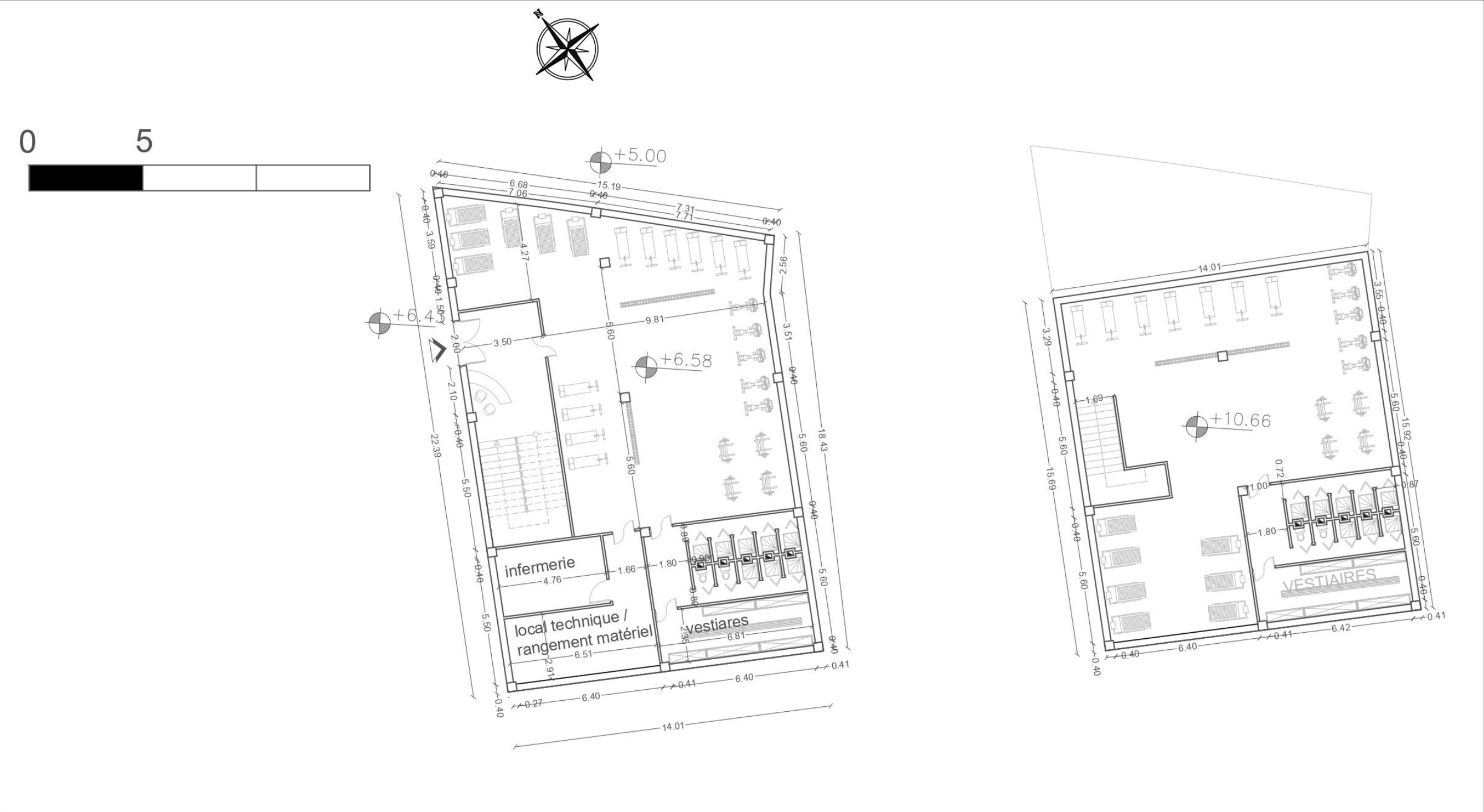
SOCLE : REZ-DE-CHAUSSEE SALLE DE SPORT
