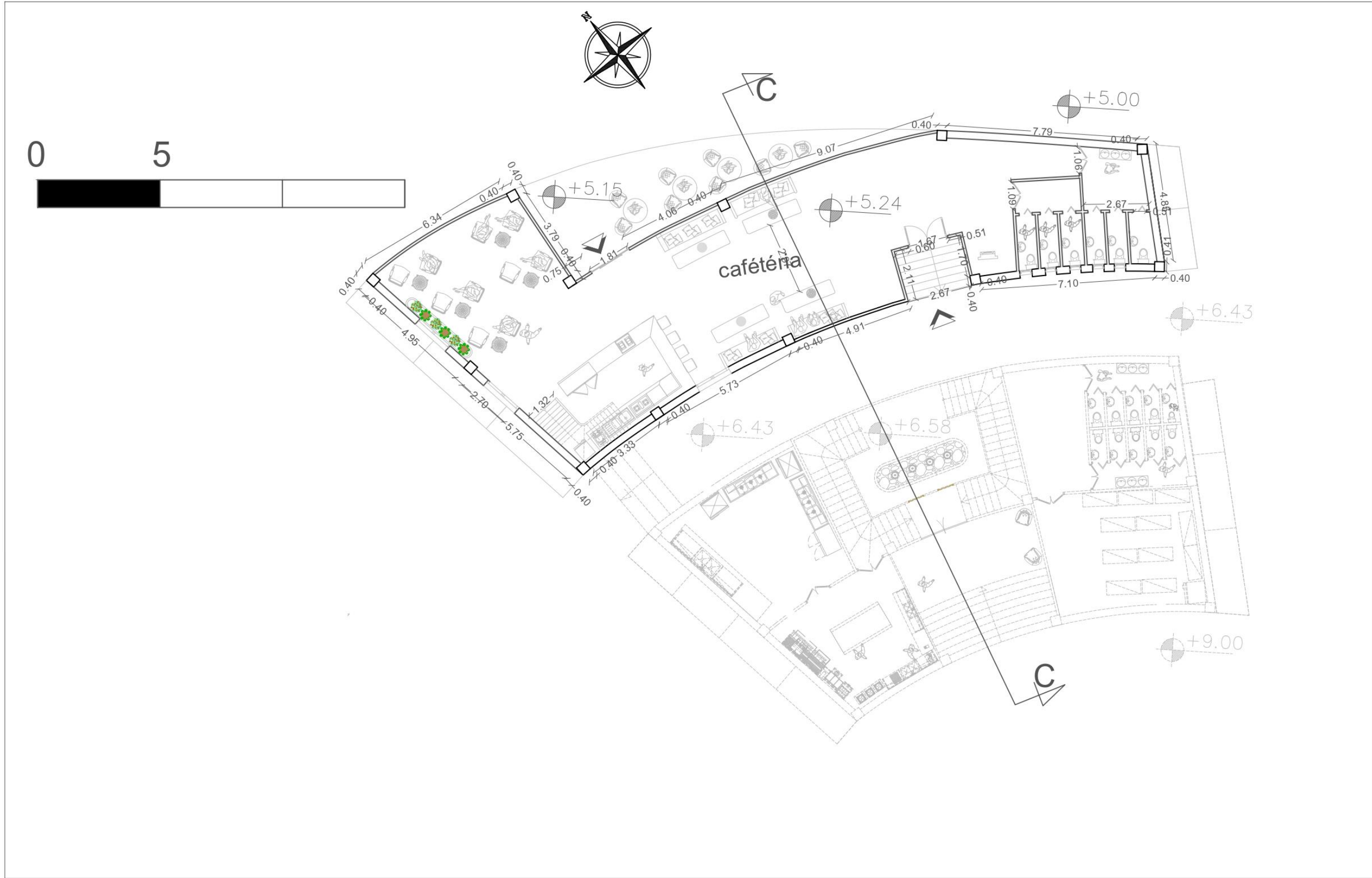
SOCLE : REZ-DE-CHAUSSEE CAFETERIA
