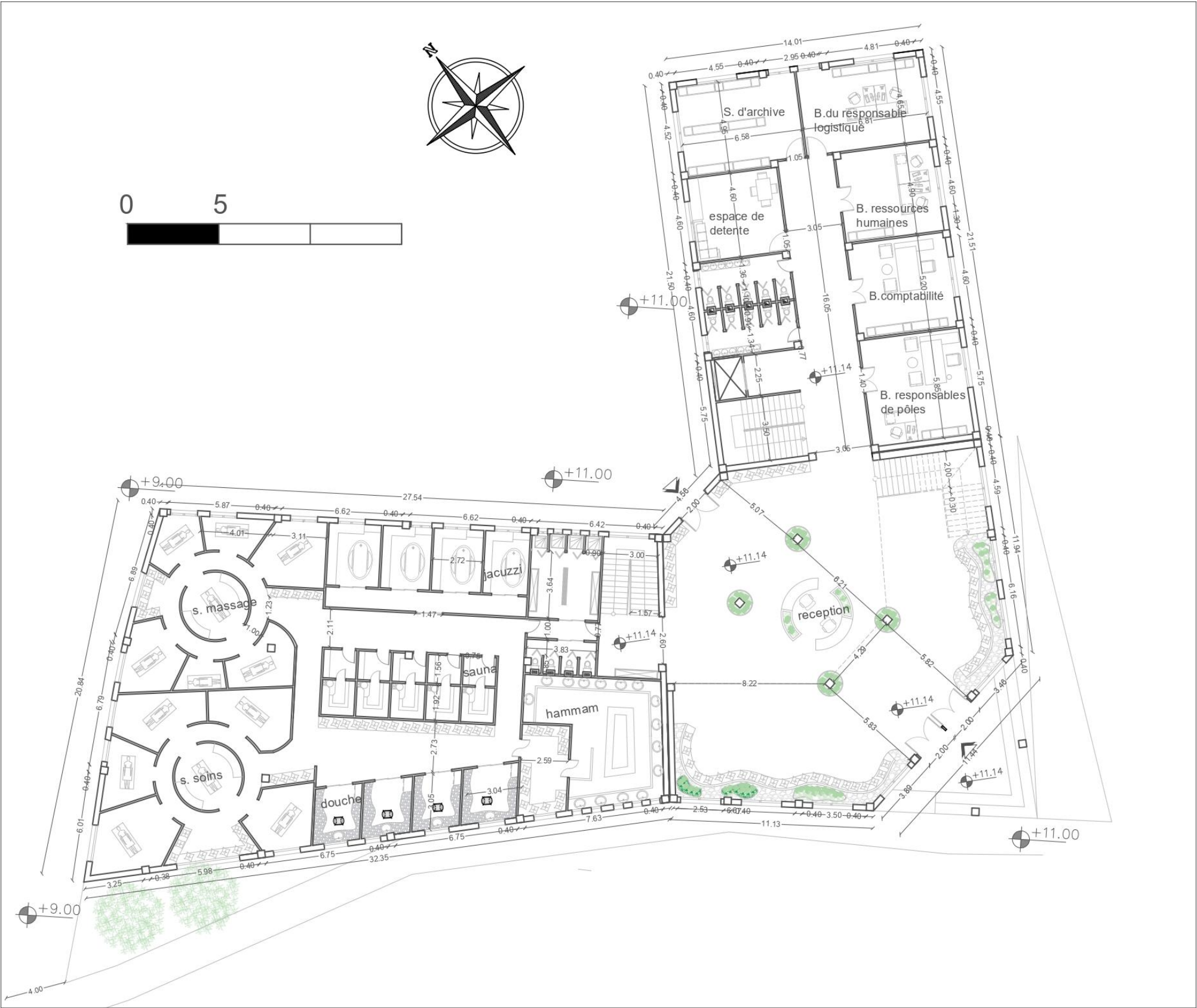
SOCLE : REZ-DE-CHAUSSEE D'ADMINISTRATION +SPA
