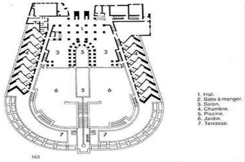
Figure 63 :plan de l'hotel gourara , source : Dubar 1963
