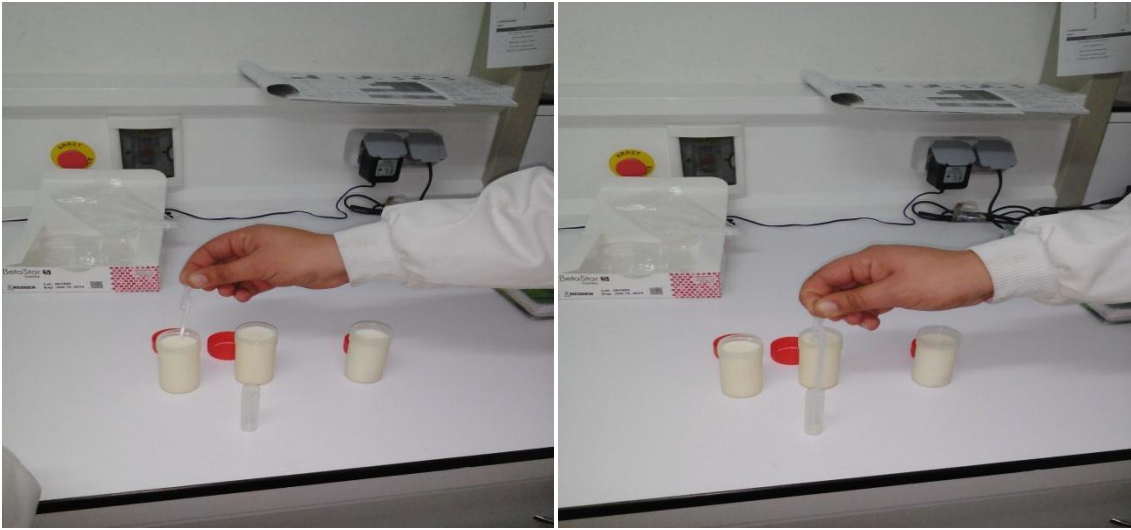
Figure 6 : le remplissage de tube en plastique avec le produit (le lait)
