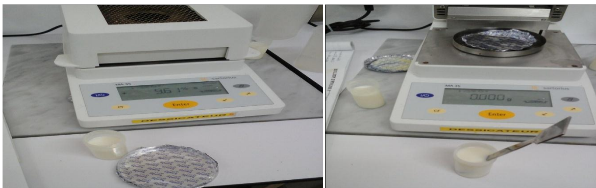
FIGURE 36 : le dessiccateur (appareil de mesure l'extrait seque)
