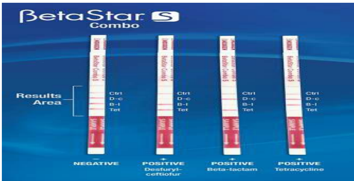
FIGURE8 la lecture selon la notice
