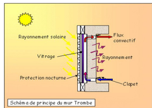
Transmise par conduction à travers le mur Figure II-12: Principe de mur capteur (ADE2008)
