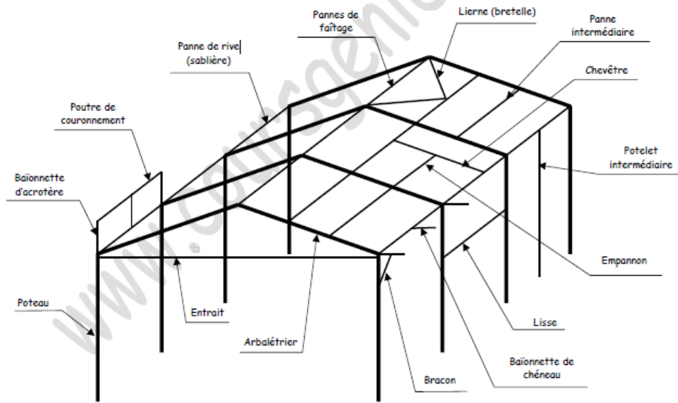
Schéma structure de charpente métallique 1
