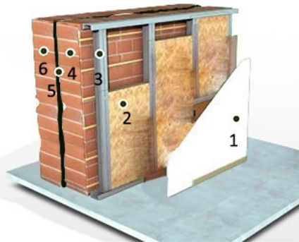
Schéma composition de Mur
